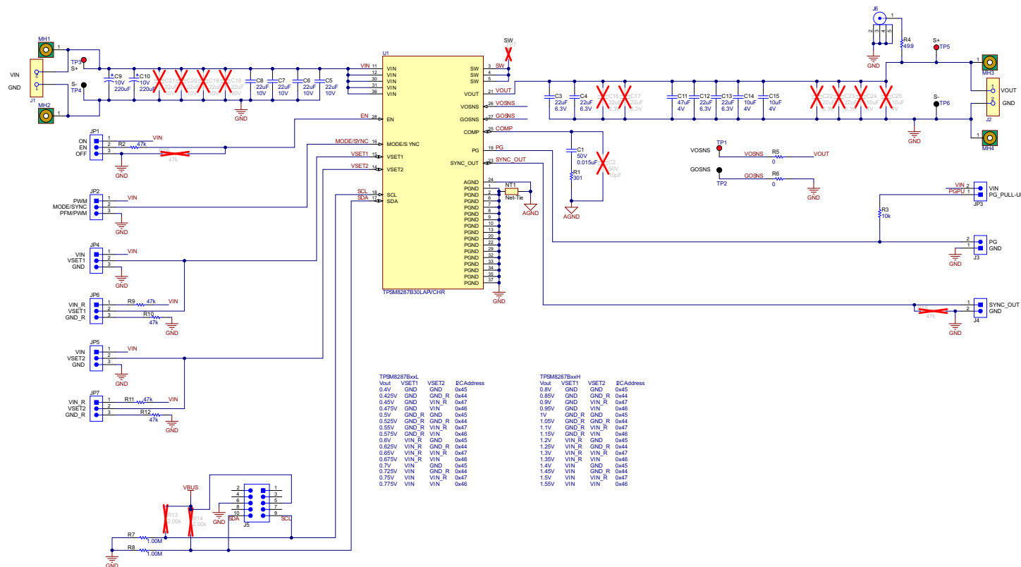
图 5-1. TPSM8287B30LAPEVM 原理图
