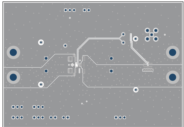
图 5-5. 内层 2
