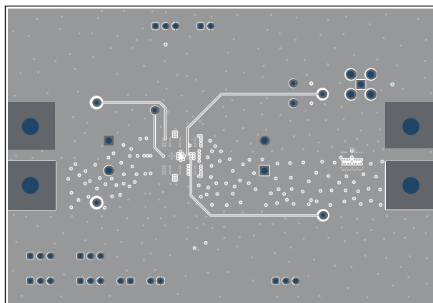
图 5-10. 底层
