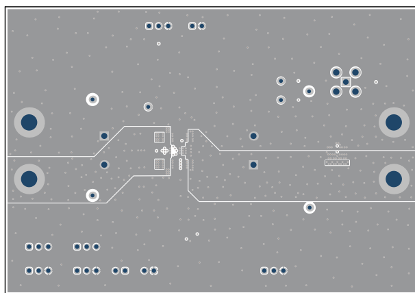
图 5-8. 内层 5
