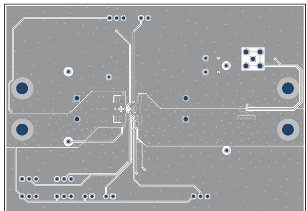
图 5-7. 内层 4
