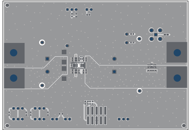
图 5-3. 顶层
