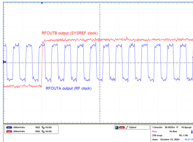
图 4-30. SYSREF 同步中继器模式
