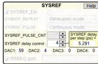
图 4-23. SYSREF 延迟控制
