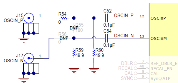
图 2-3. 参考时钟
