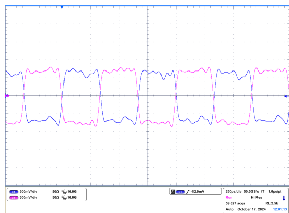
图 4-34. 非同步示例 1
