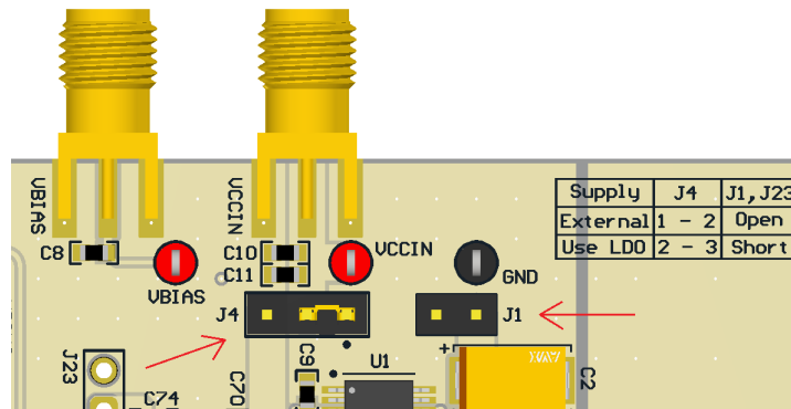
图 2-2. 电源跳线
