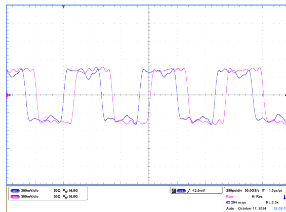
图 4-37. 类别 3 同步
