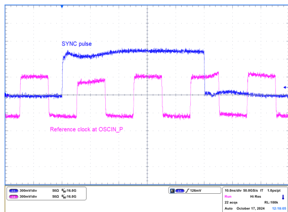
图 4-36. 时间关键型 SYNC 脉冲
