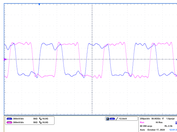
图 4-35. 非同步示例 2
