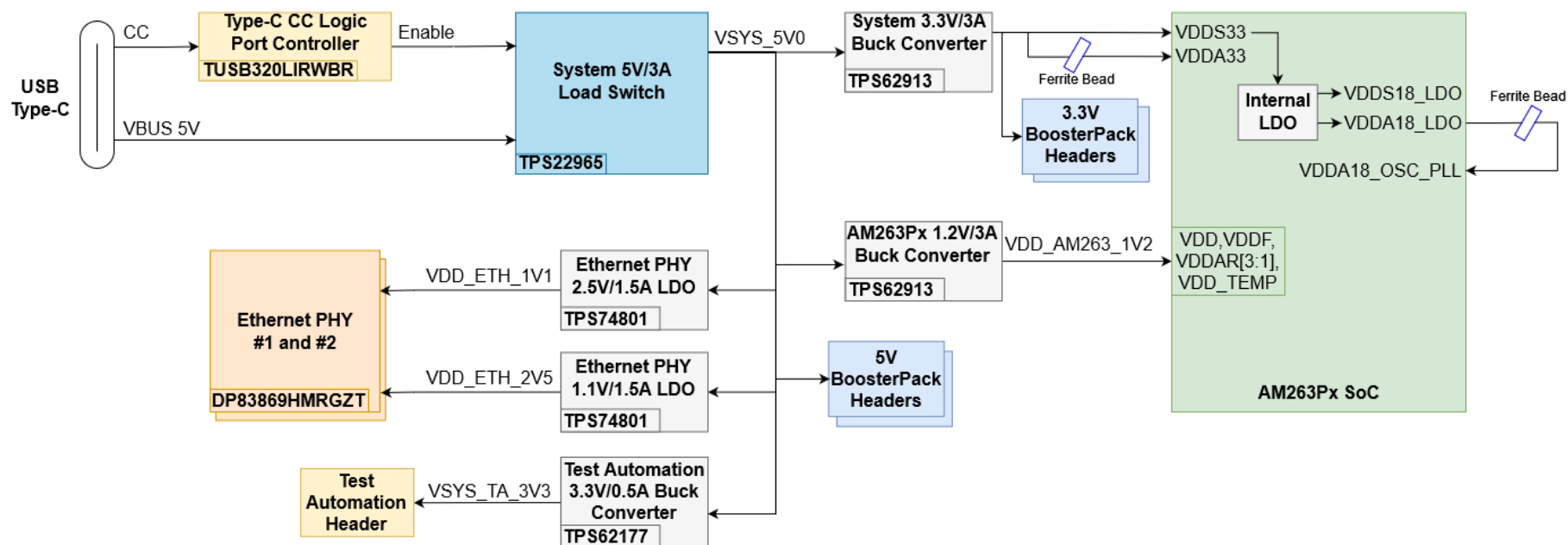
图 2-4. AM263Px LaunchPad 的电源树图
