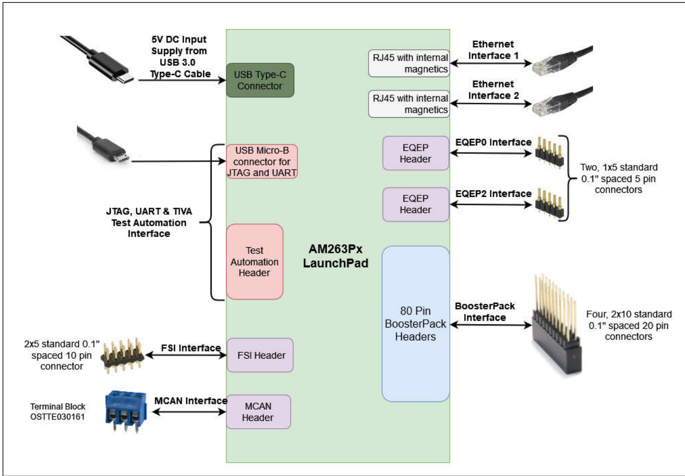
图 1-2. 系统架构
