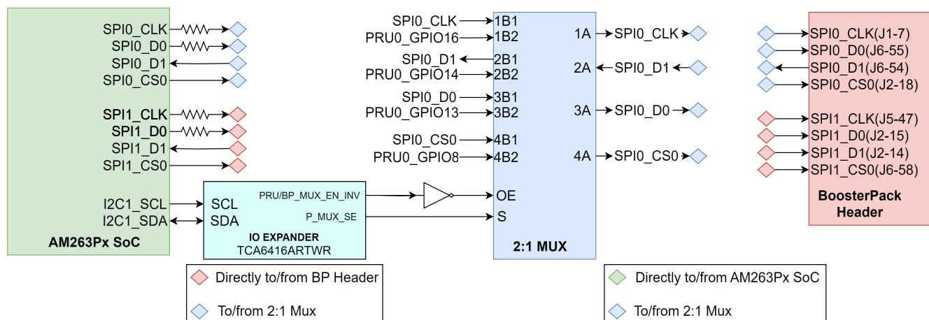
图 2-21. SoC SPI 至 BoosterPack — LP-AM263P 修订版 A
