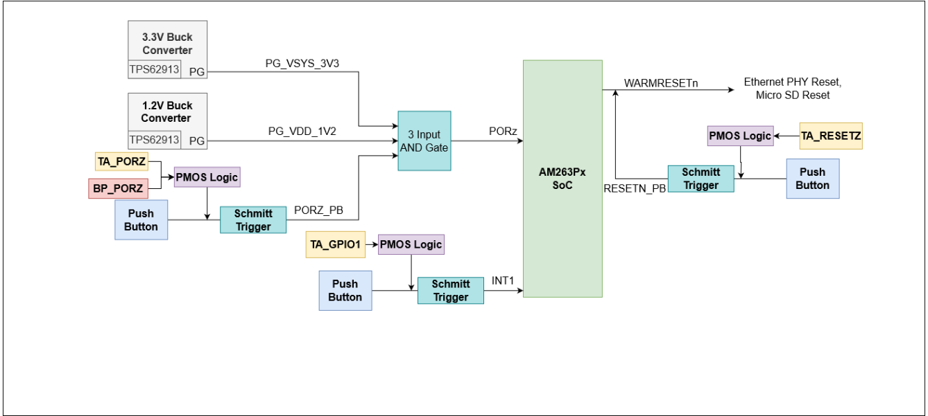
图 2-9. 复位架构
