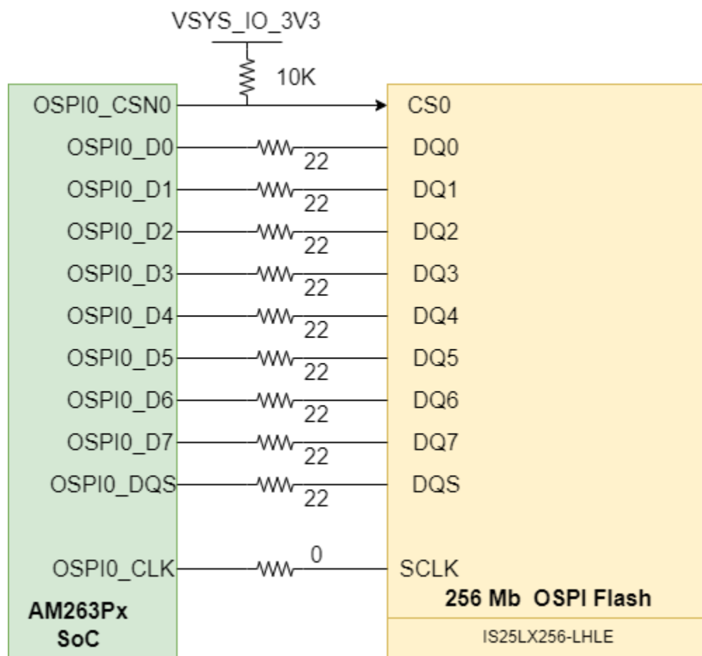
图 2-13. OSPI 闪存接口
