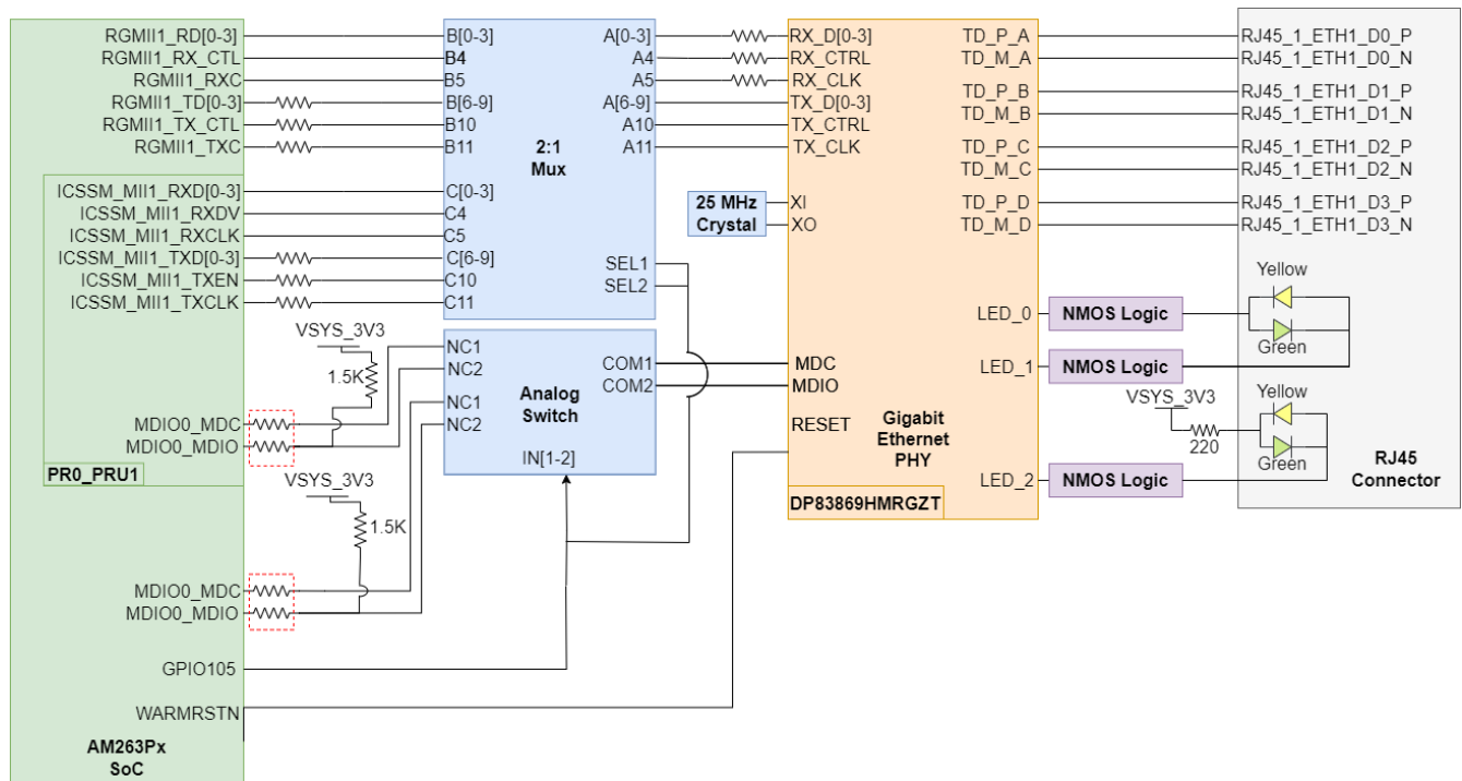
图 2-16. 以太网 PHY #1
