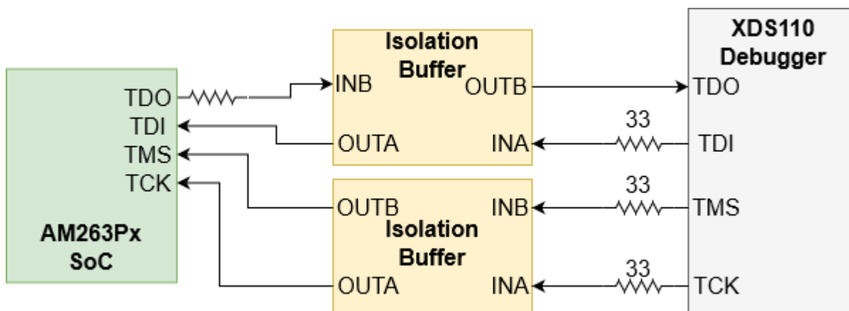
图 2-25. JTAG 与 XDS110 的接口
