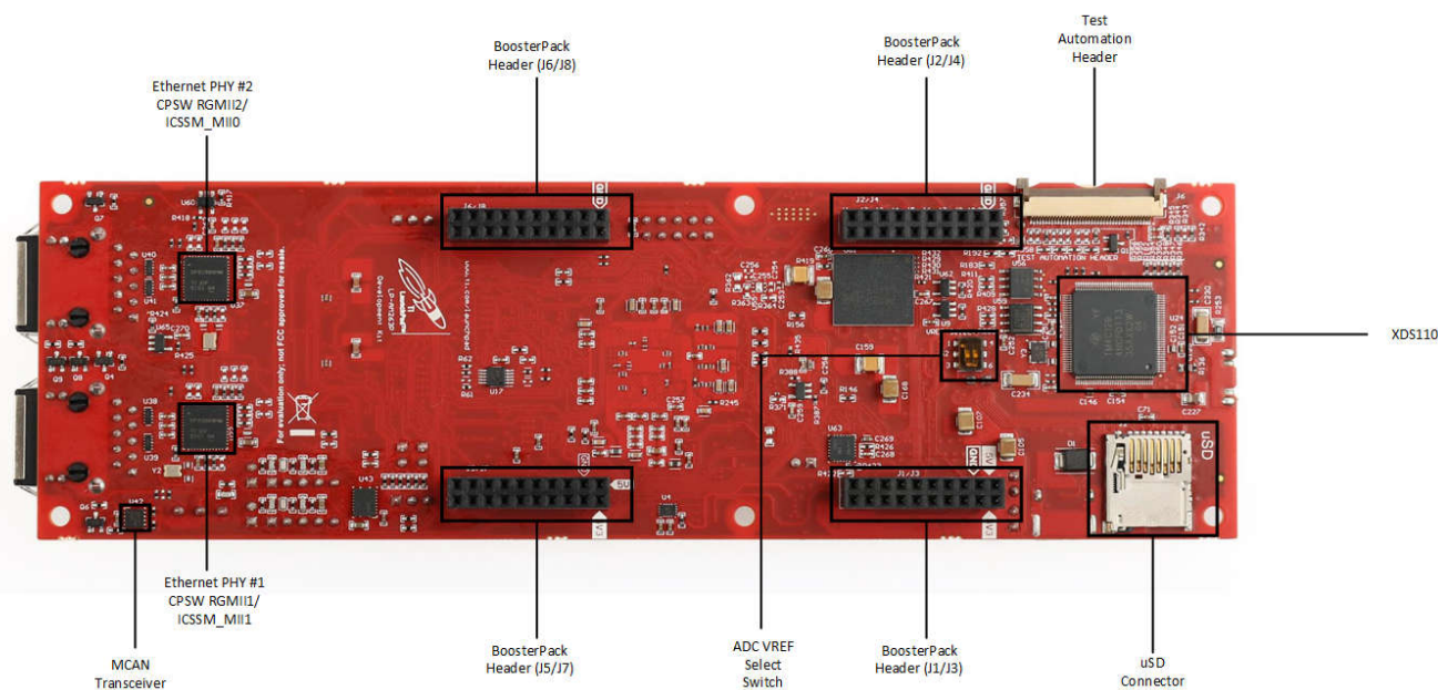
图 1-4. AM263Px LaunchPad 底部元件标识
