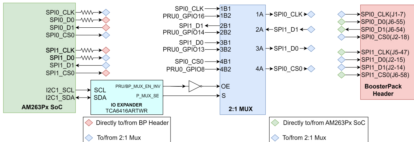
图 2-20. SoC SPI 至 BoosterPack — LP-AM263P 修订版 E2
