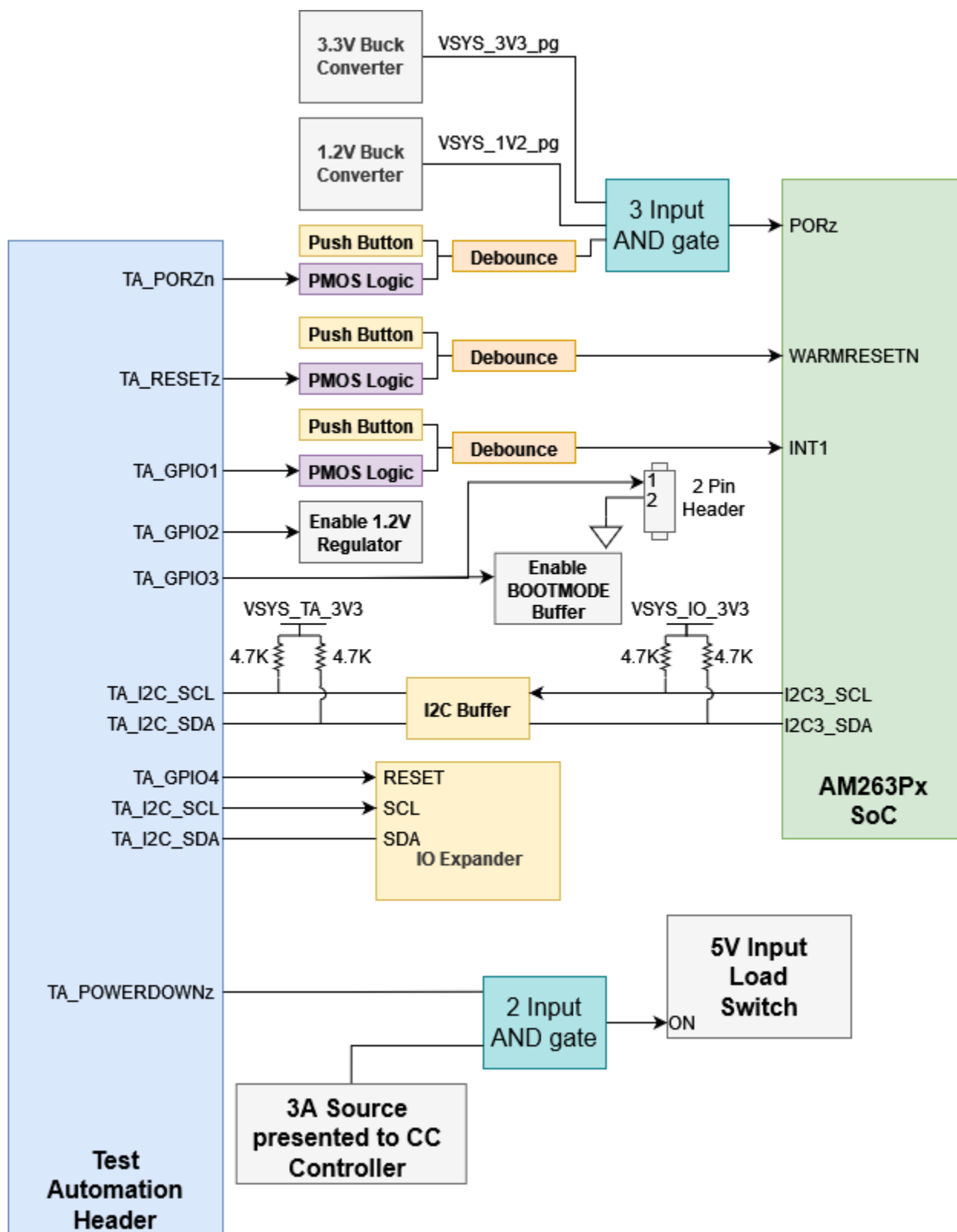
图 2-26. 测试自动化接头
