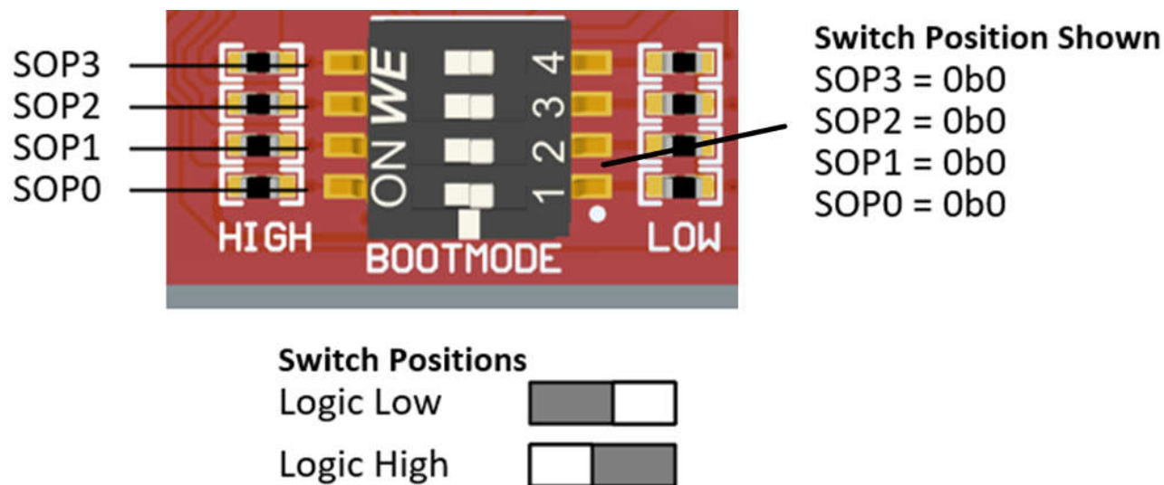
图 2-6. 引导模式 DIP 开关位置 — LP AM263P SW1 SOP 开关
