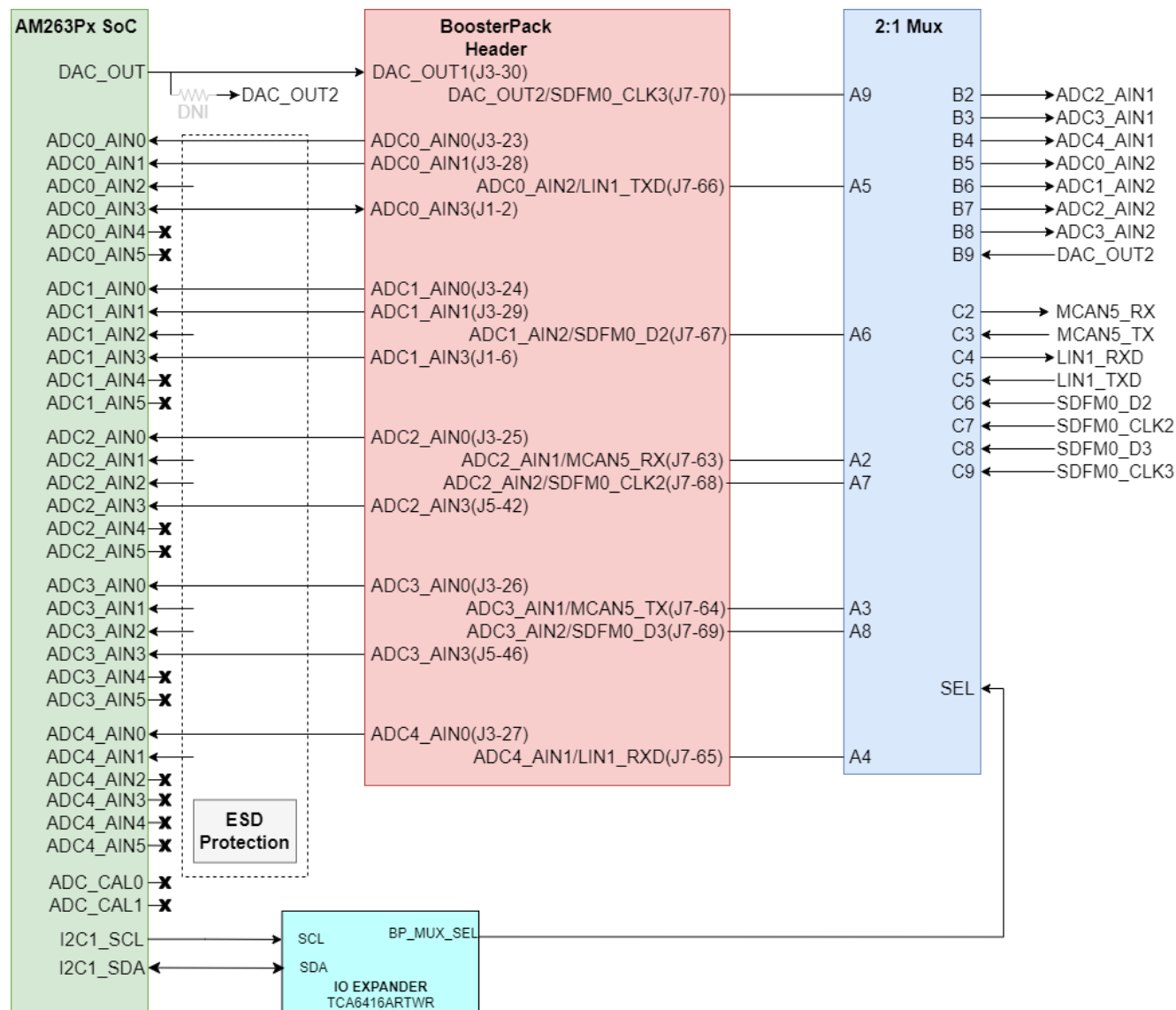
图 2-28. ADC/DAC 信号路径
