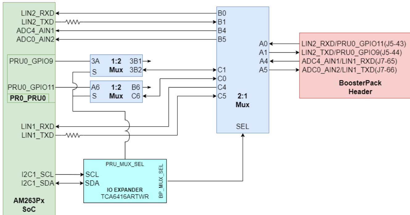
图 2-27. LIN 实例到 BoosterPack 接头
