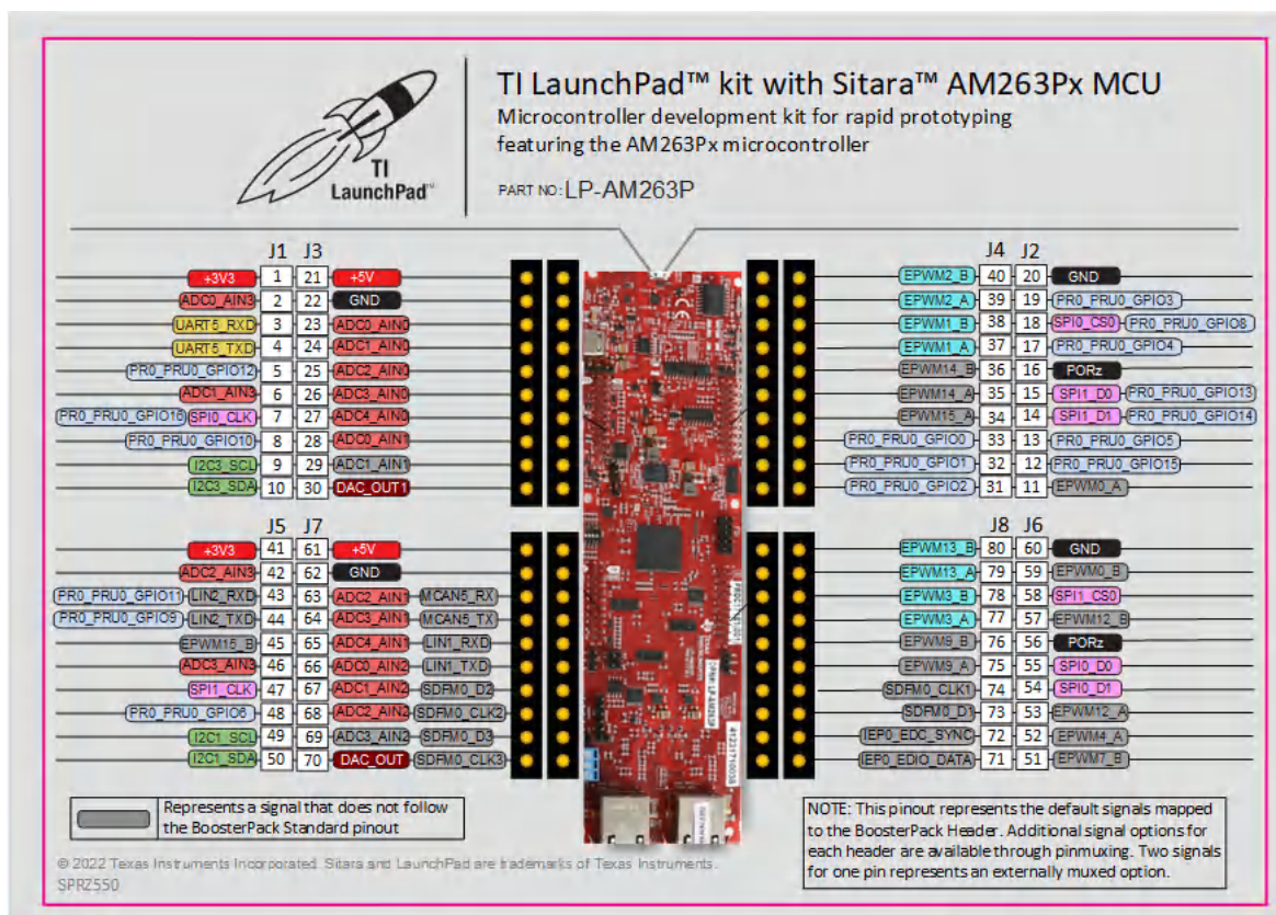
图 2-32. AM263Px LaunchPad BoosterPack 引脚排列
