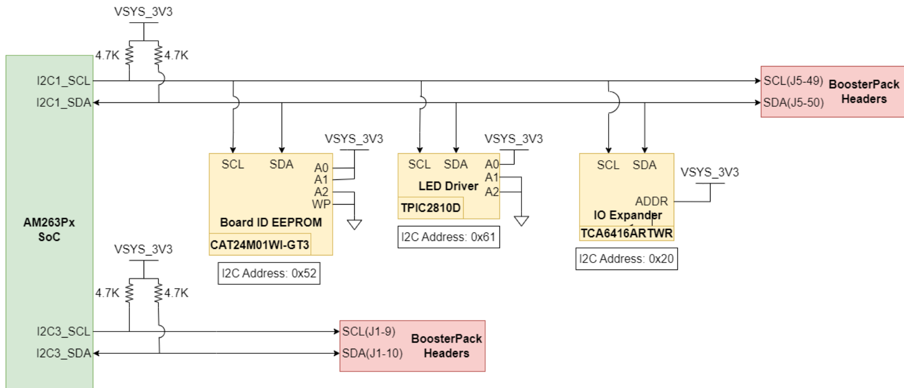
图 2-18. I2C 目标
