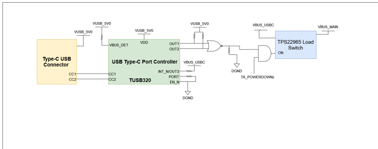
图 2-2. Type-C CC 配置
