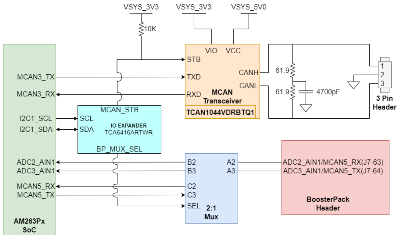
图 2-23. MCAN 收发器和 BoosterPack 接头
