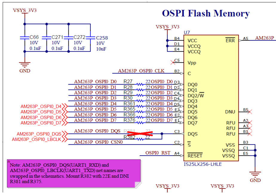
图 5-1. LP-AM263P 原理图中的 OSPI DQS 和 LBCLK 网络注意事项
