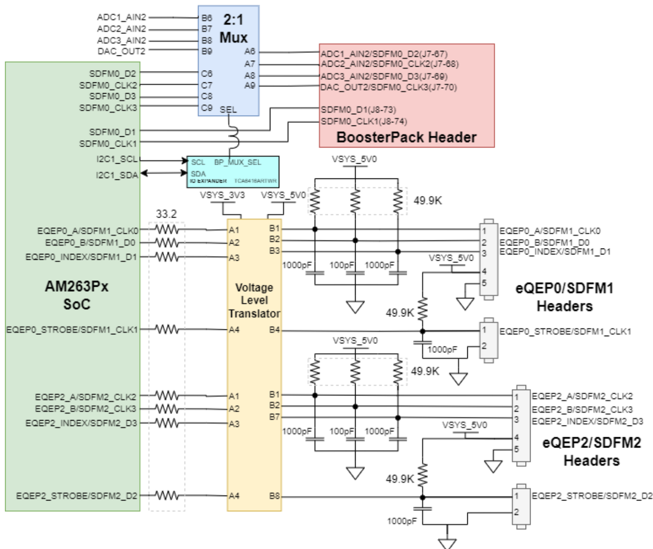
图 2-30. EQEP 和 SDFM 信号映射
