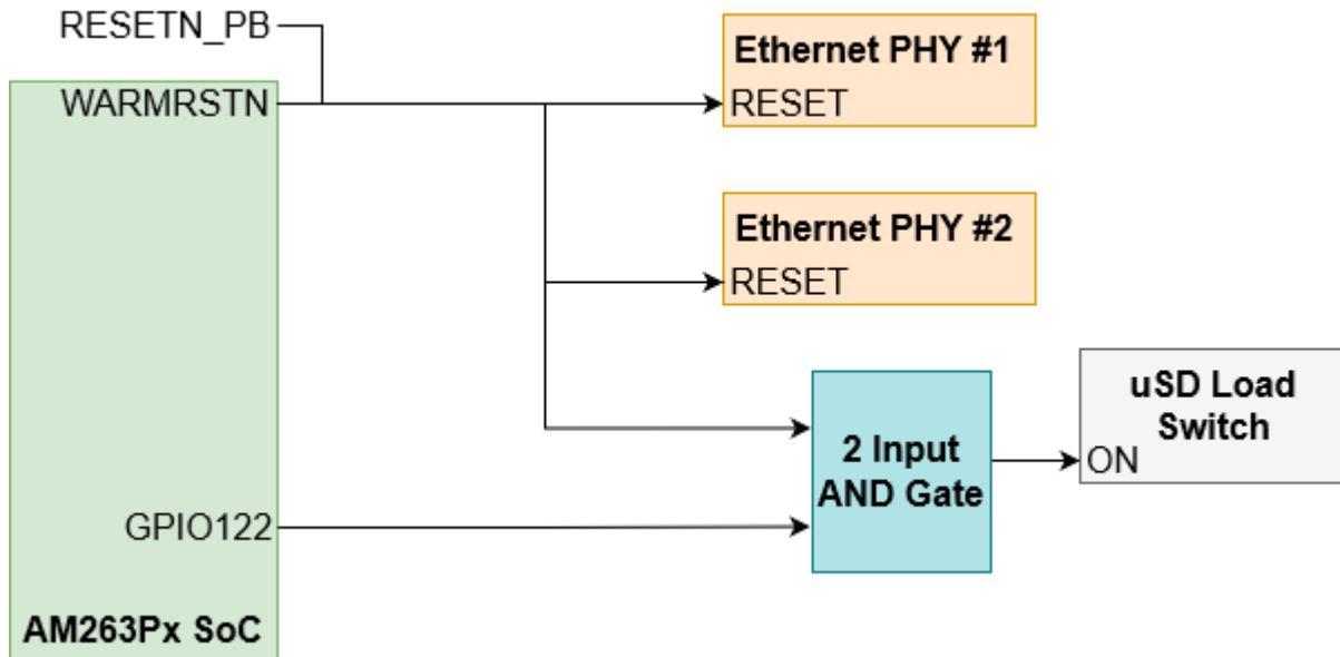
图 2-11. WARMRESETn 复位信号树
