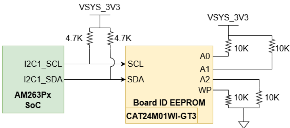
图 2-15. 电路板 ID EEPROM
