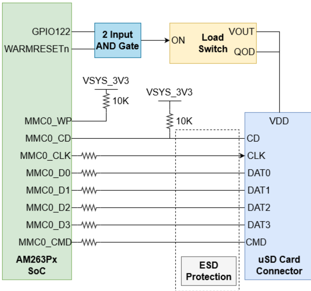
图 2-14. Micro SD 卡连接器
