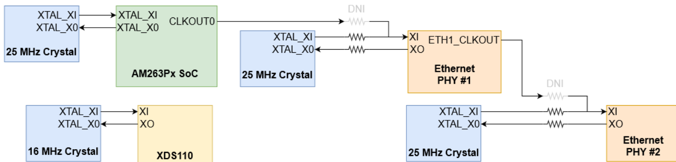
图 2-12. AM263Px LaunchPad 时钟树
