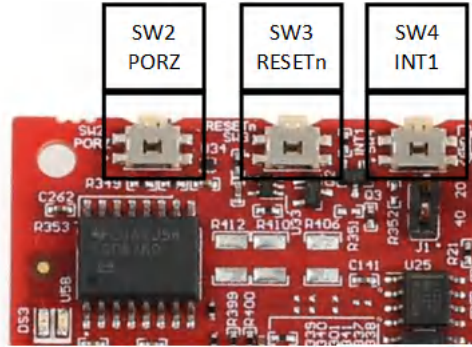
图 2-5. 按钮
