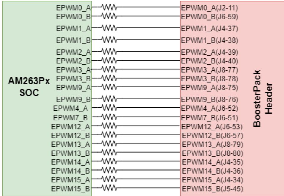
图 2-31. EPWM 信号到 BoosterPack 接头的映射
