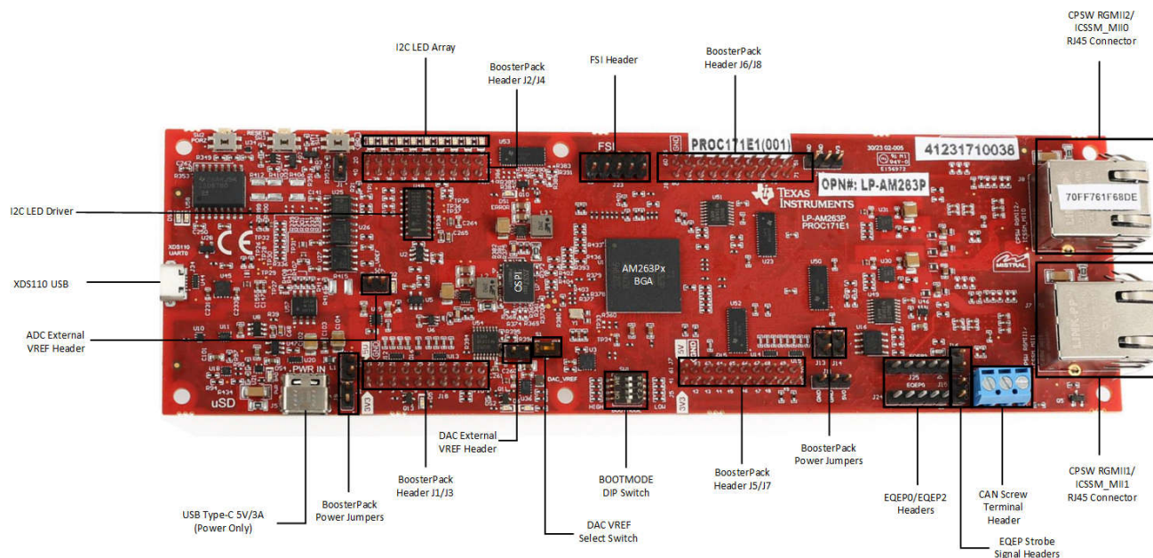
图 1-3. AM263Px LaunchPad 顶部元件标识
