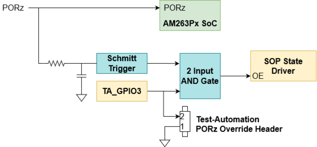
图 2-10. PORz 复位信号树
