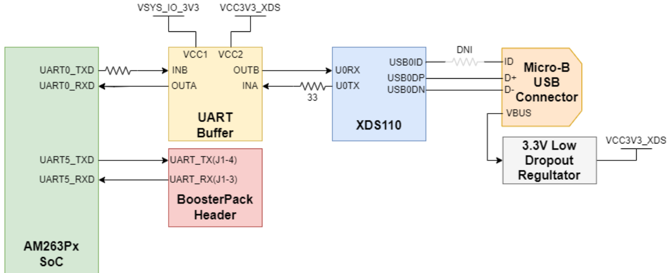
图 2-22. UART
