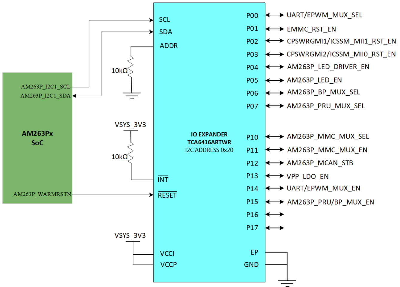
图 2-7. IO 扩展器
