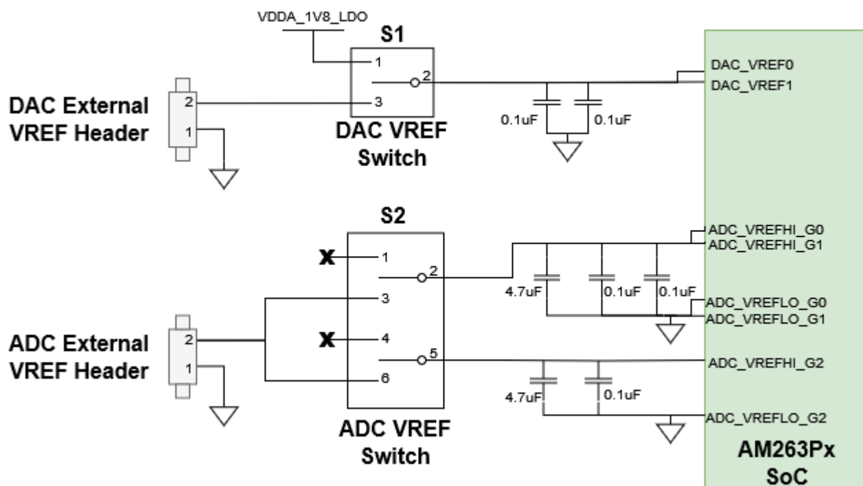
图 2-29. ADC 和 DAC VREF 开关
