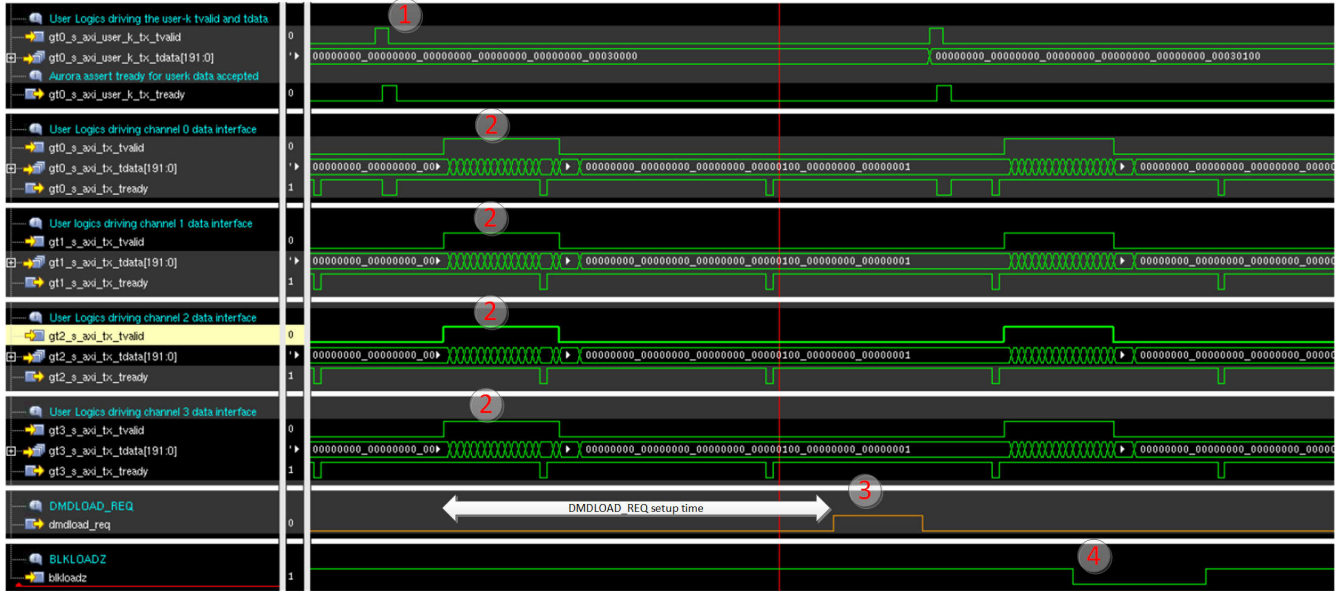
图 8-20. 三个 DMD 行的加载操作的 DMDLOAD_REQ 建立时间
