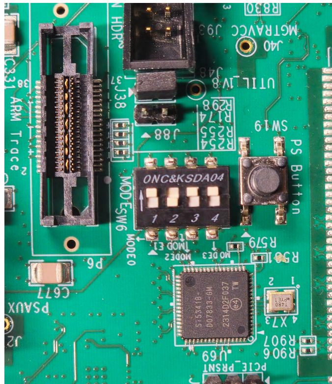
图 8-10. FPGA 配置模式 2 (QSPI)
