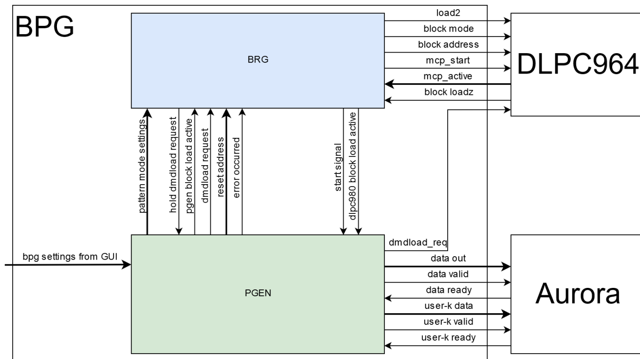
图 6-2. BPG 模块硬件方框图
