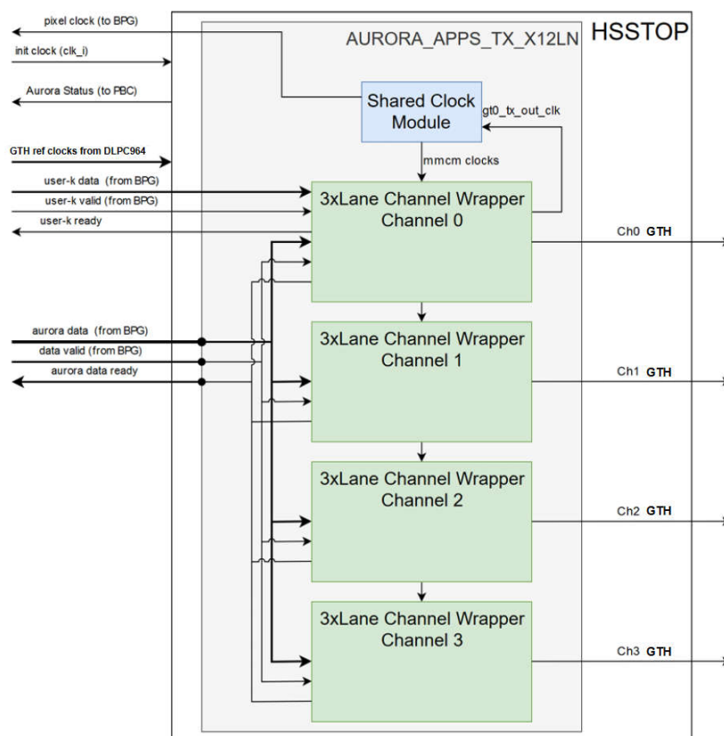
图 6-8. HSSTOP 模块硬件方框图
