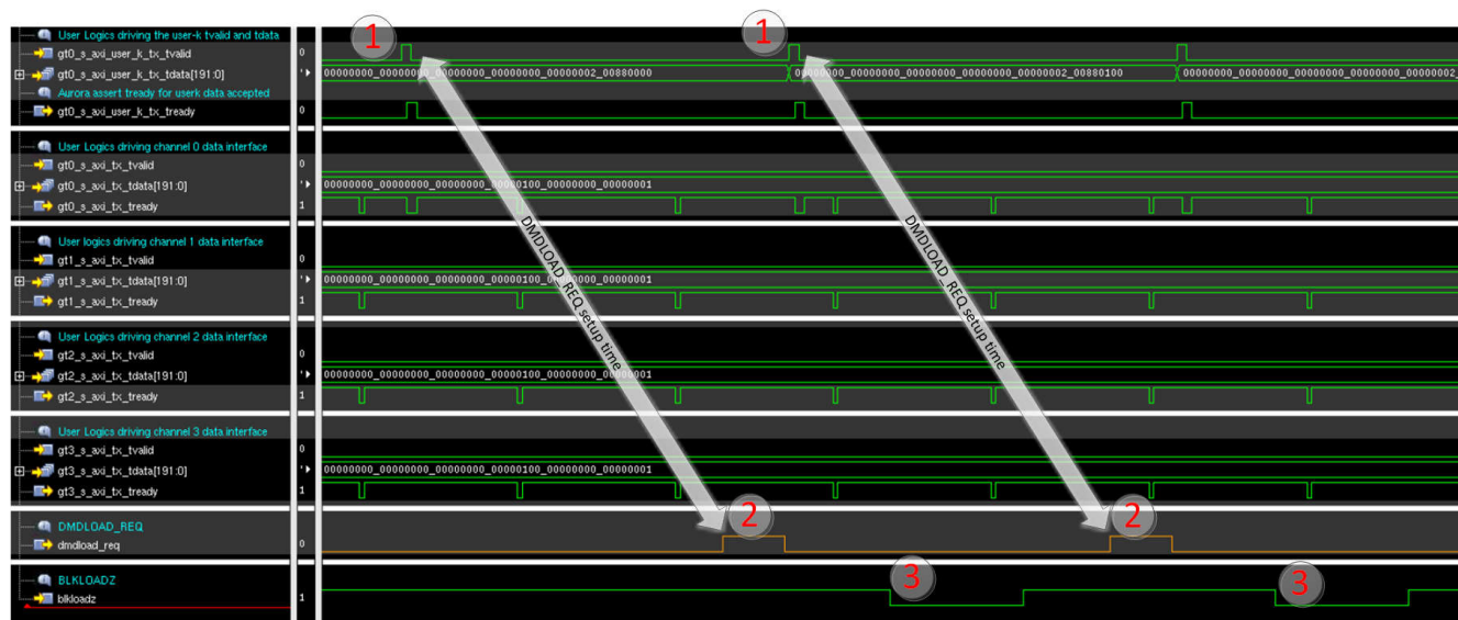
图 8-21. 块置位操作的 DMDLOAD_REQ 建立时间
