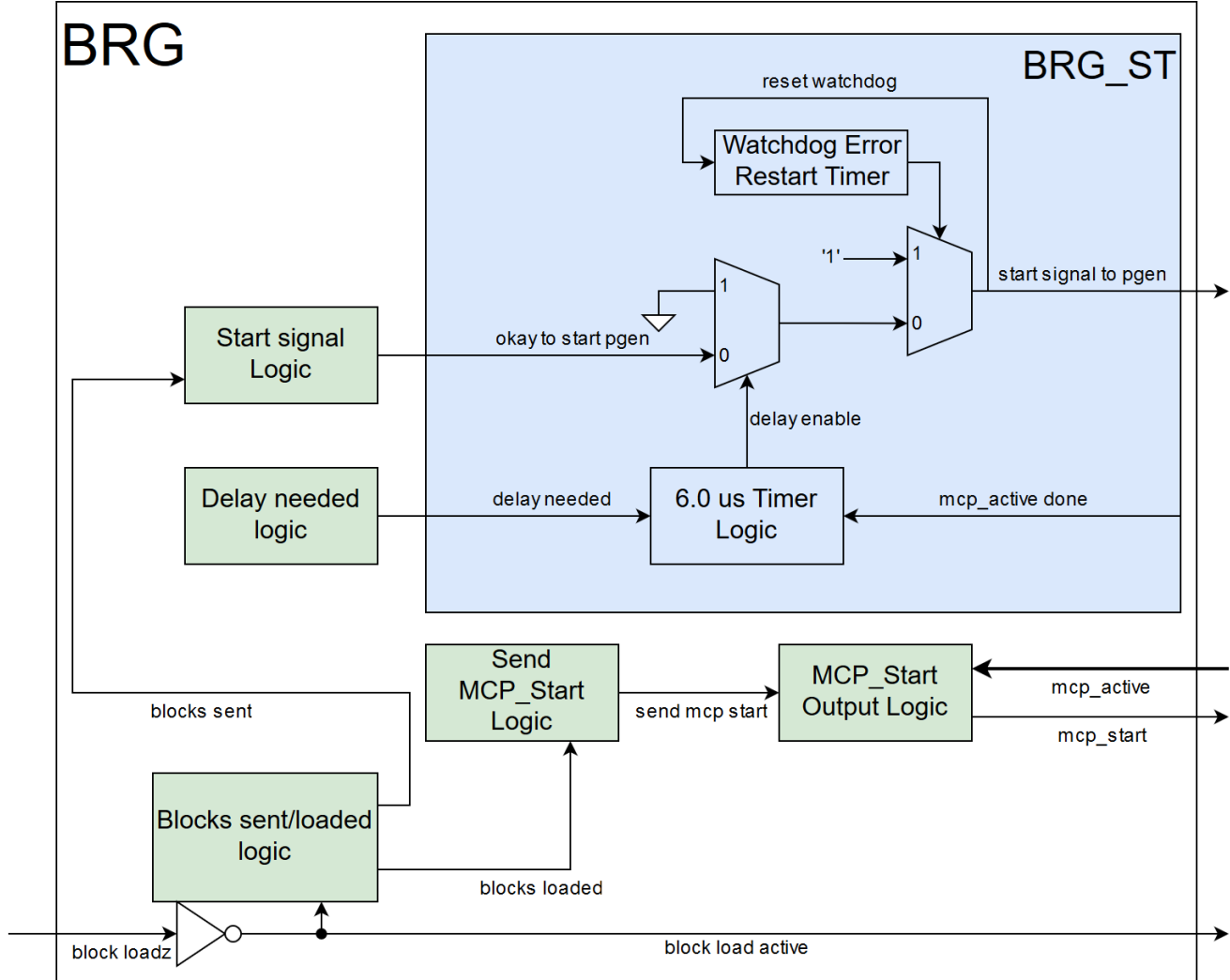
图 6-3. BRG 模块硬件方框图
