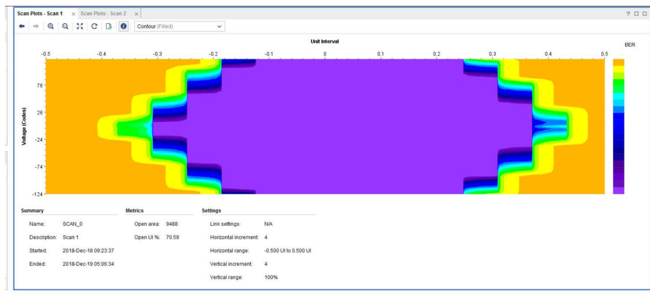
图 8-26. 使用 TI EVM 硬件时 Aurora Channel0 Link0 的 IBERT 眼图扫描
