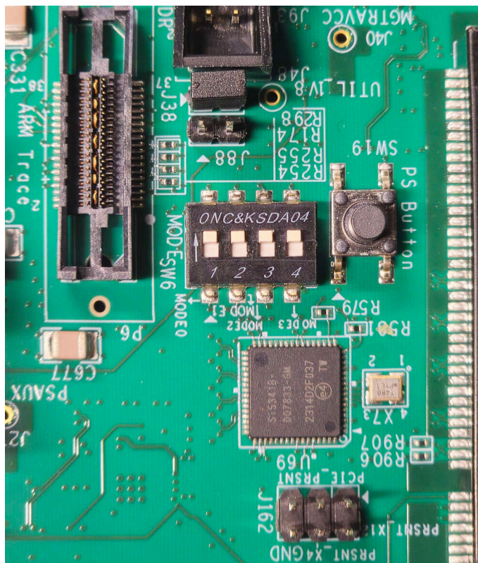
图 8-9. FPGA 配置模式 1 (JTAG)
