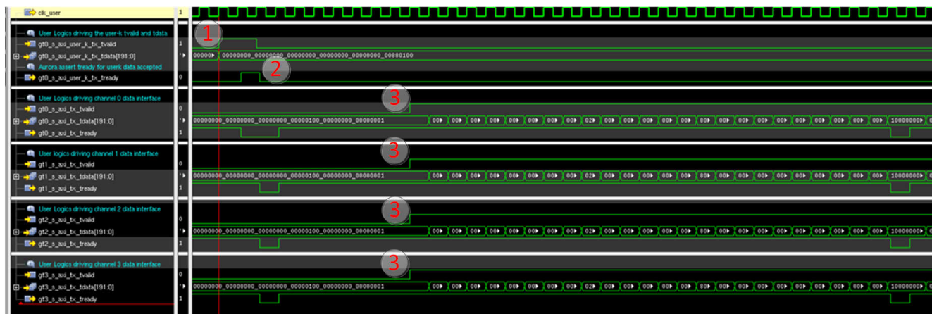
图 8-17. 块以块控制字开始的波形
