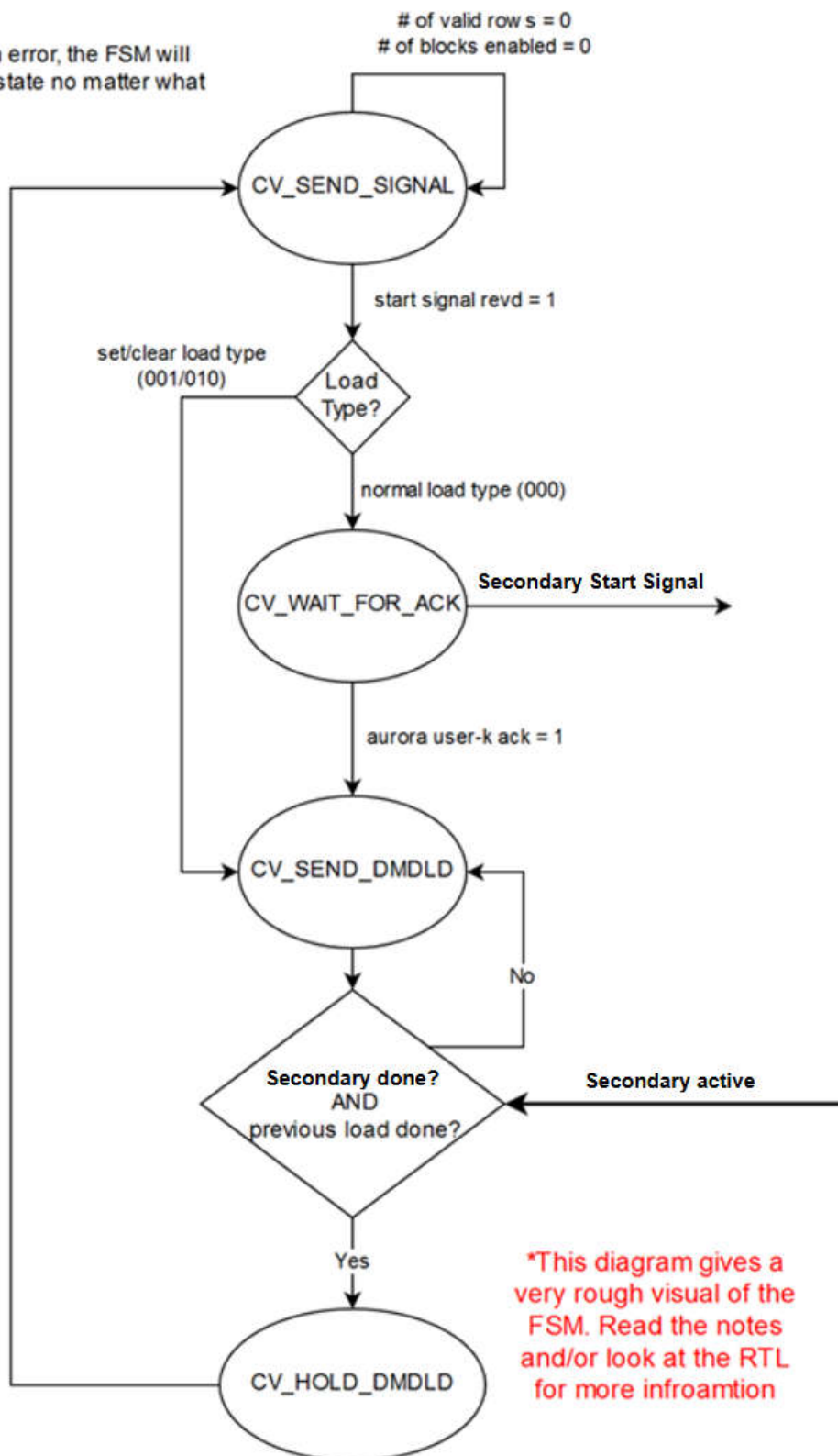
图 6-6. PGEN_MCTRL FSM
