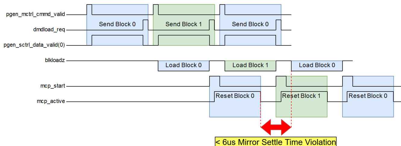
图 6-4. BRG_ST 时序
