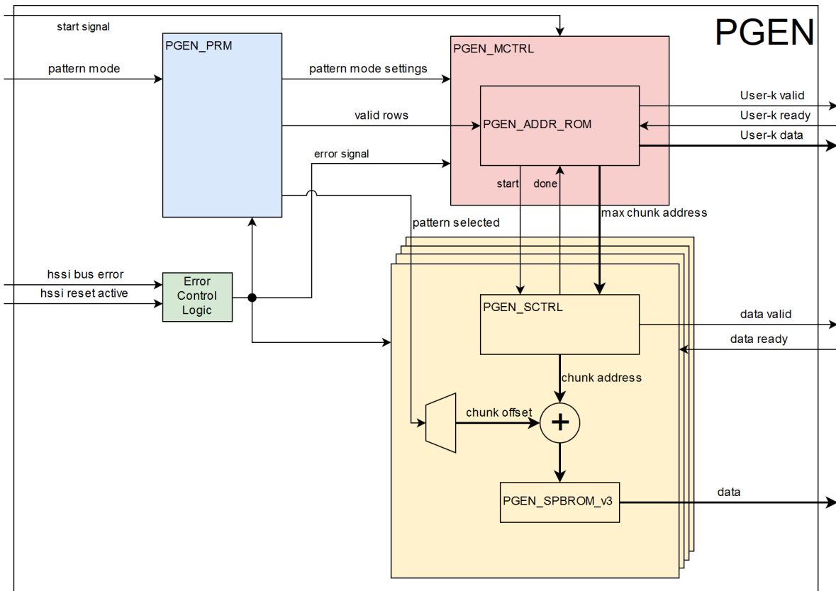
图 6-5. PGEN 模块
