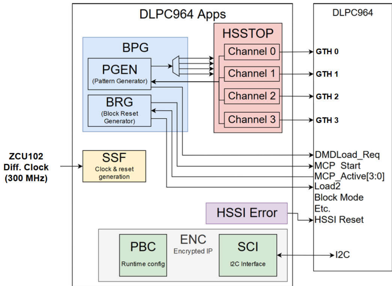
图 6-1. Apps FPGA 硬件方框图
