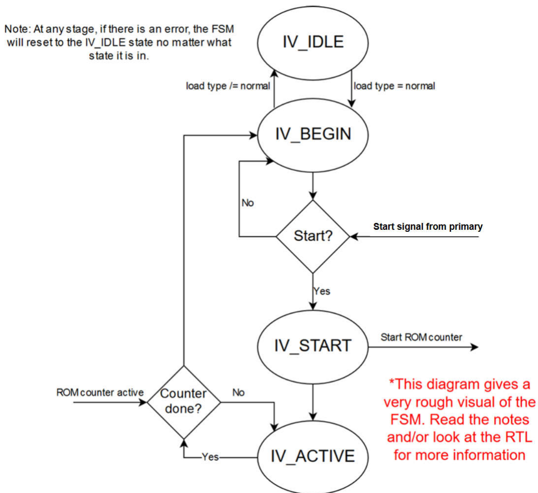
图 6-7. PGEN_SCTRL FSM
