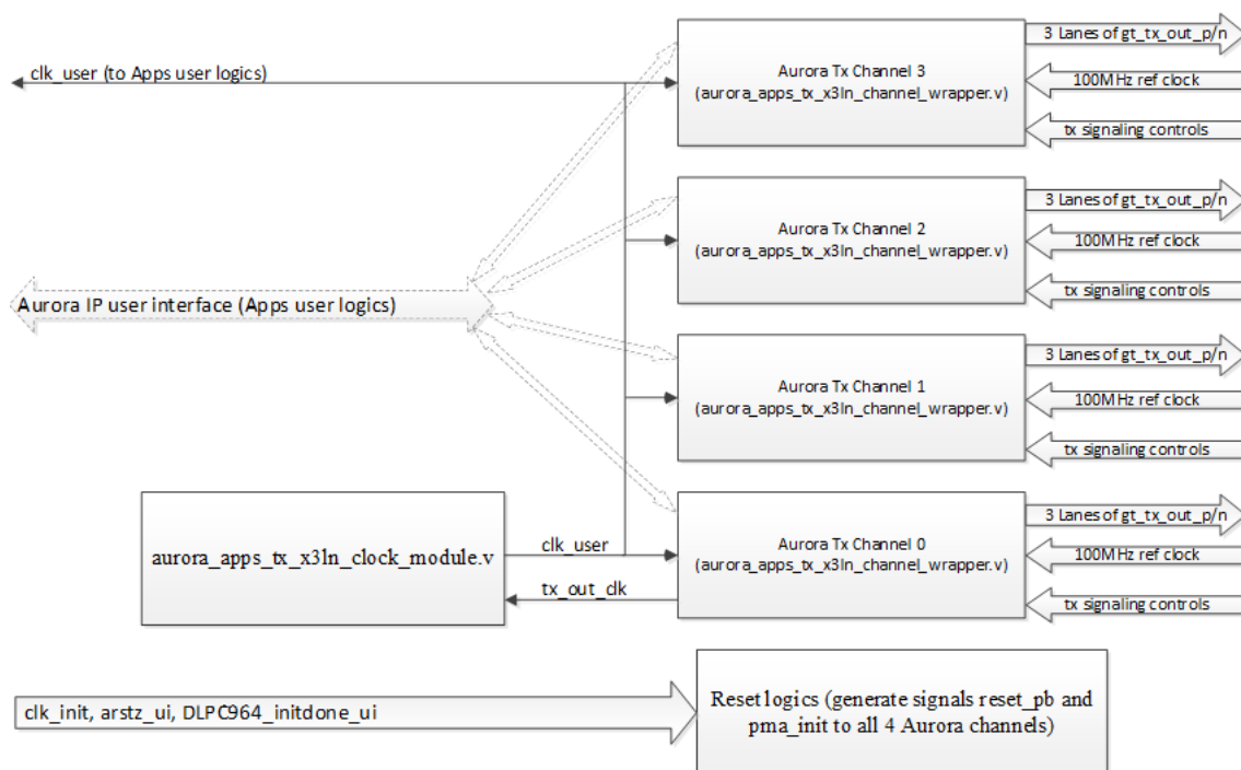
图 8-16. Aurora_apps_tx_x12ln.v RTL 方框图
