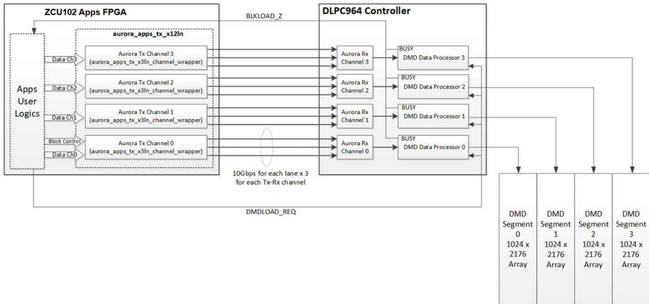
图 8-11. DLPC964 系统方框图
