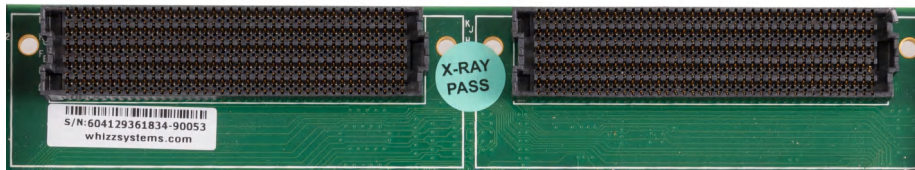
图 2-5. AMD EVM HPC FMC 公连接器
