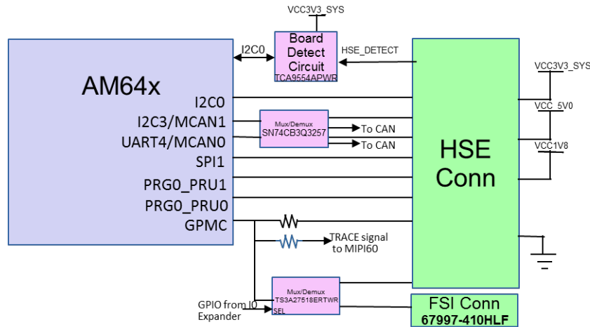
图 2-27. AM64x/AM243x 高速扩展连接器
