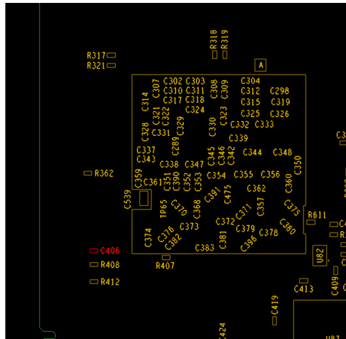
图 5-7. C406 的 PCBA 底面
