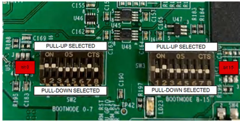
图 2-9. AM64x/AM243x EVM PCB，引导模式选择开关 ( SW2、SW3 )
