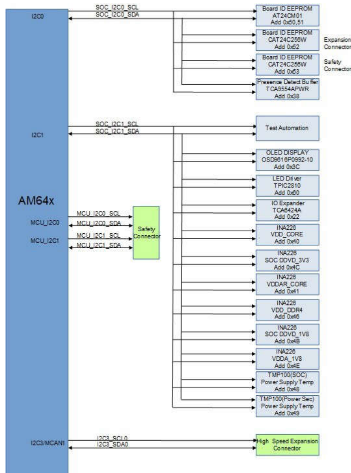
图 2-31. AM64x/AM243x I2C 接口和外设地址分配
