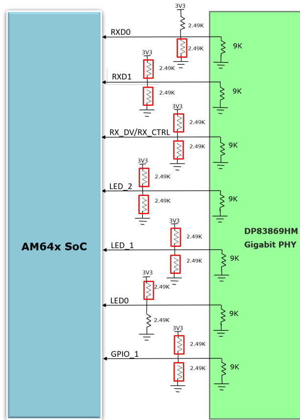
图 2-22. AM64x/AM243x 以太网接口 - ICSSG1 以太网自举设置
