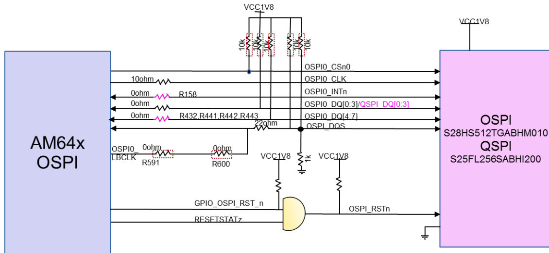
图 2-18. AM64x/AM243x OSPI 接口
