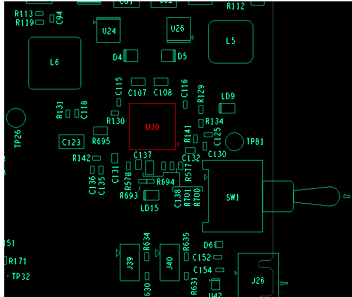
图 5-6. U30 的 PCBA 顶面
