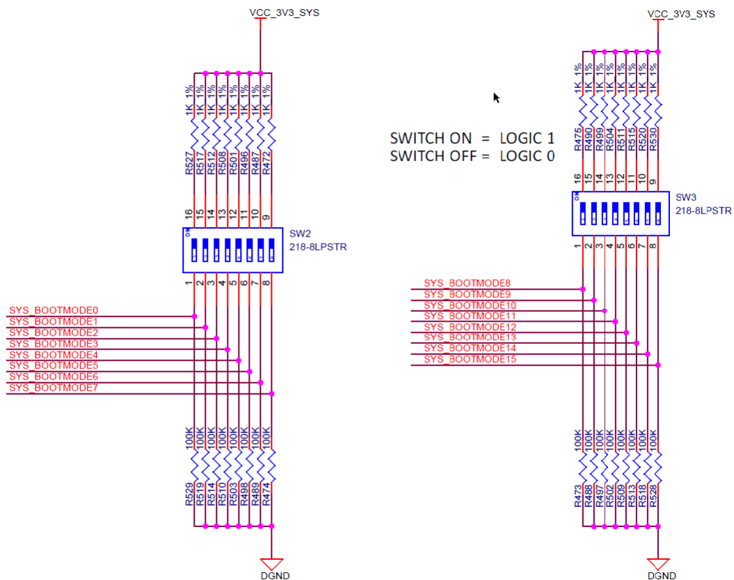
图 2-8. AM64x/AM243x EVM 原理图摘录，引导模式选择开关 ( SW2、SW3 )
