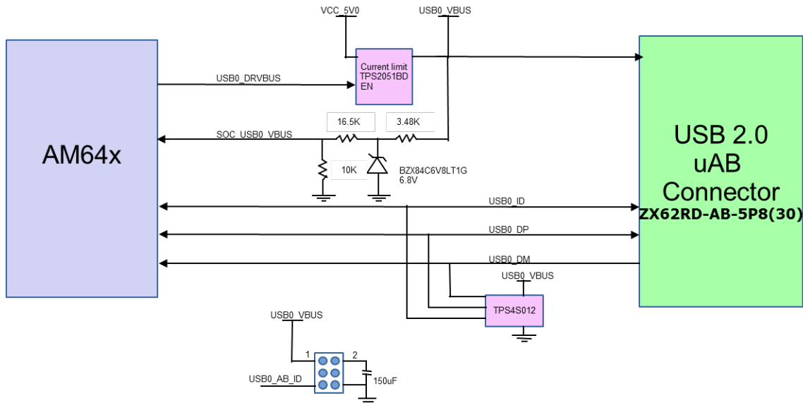
图 2-25. AM64x/AM243x USB 2.0 主机接口
