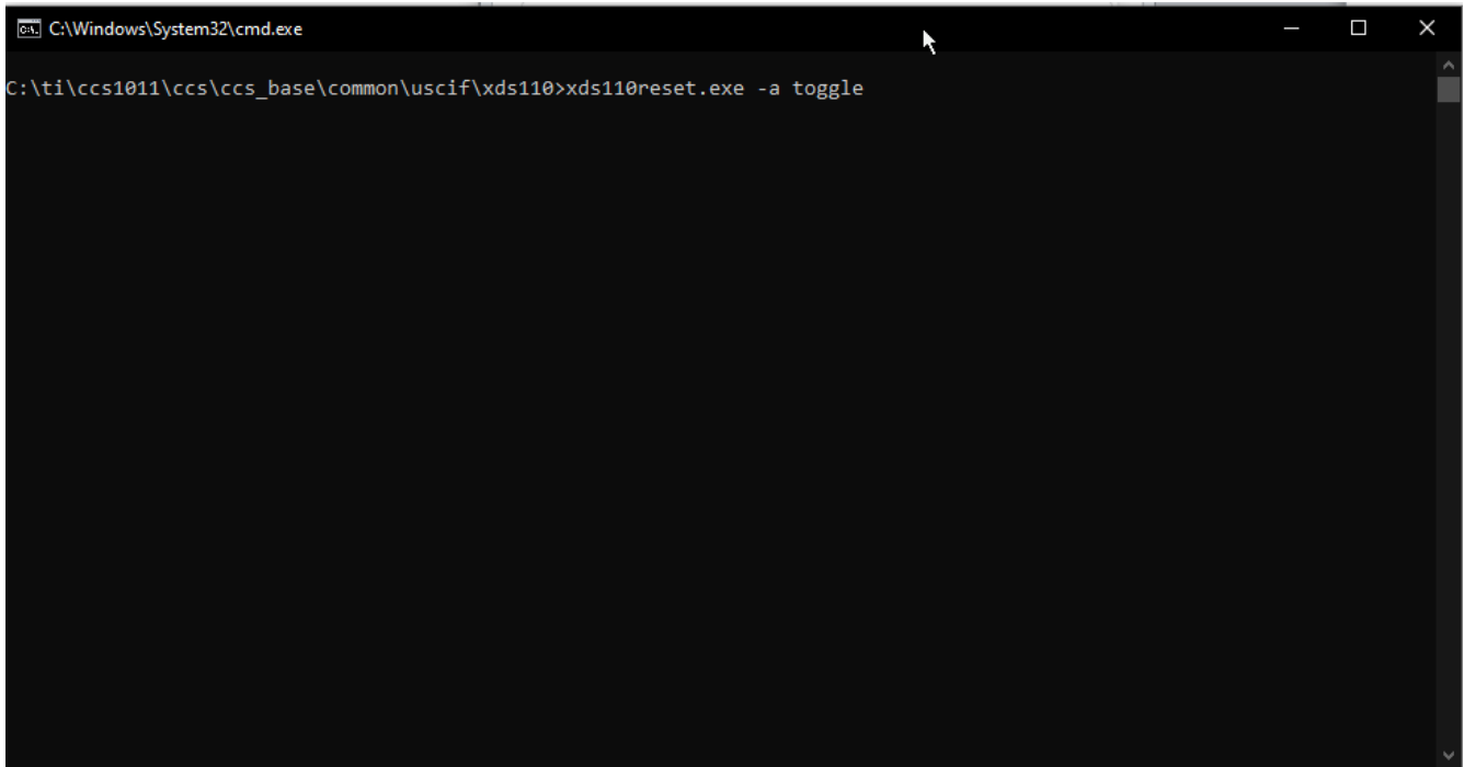
图 5-3. XDS110 debug reset 实用程序命令行功能
