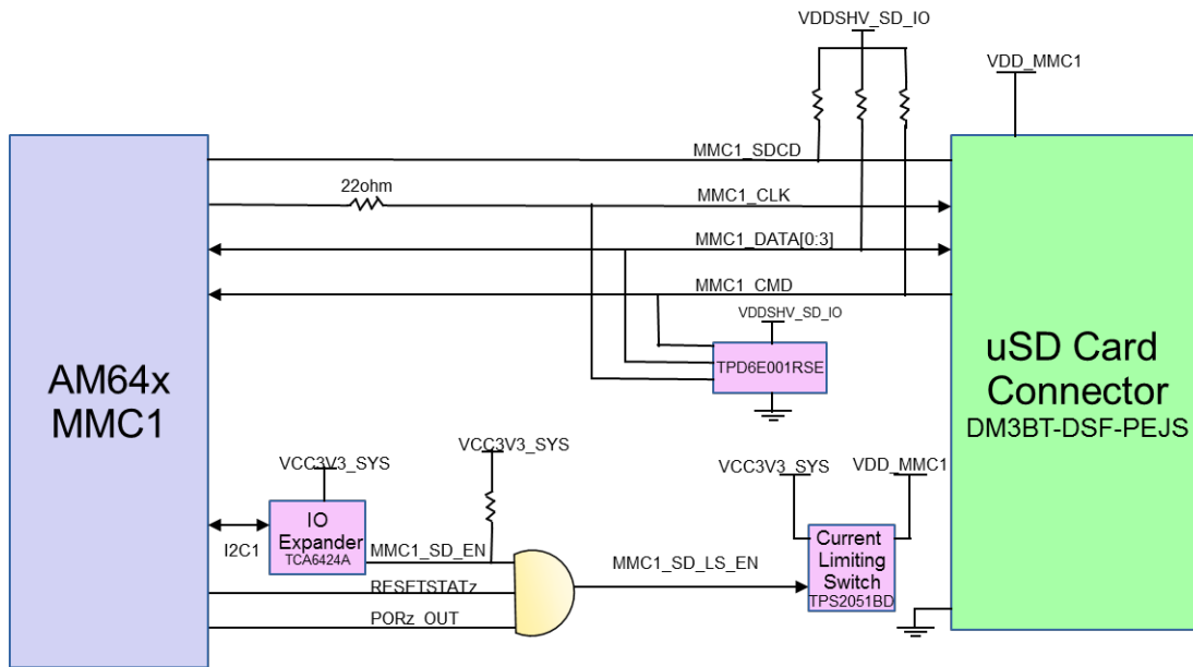
图 2-16. Micro SD 接口
