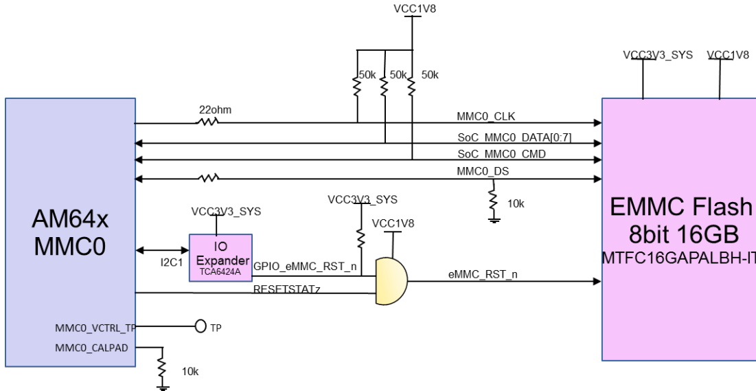
图 2-17. eMMC 接口
