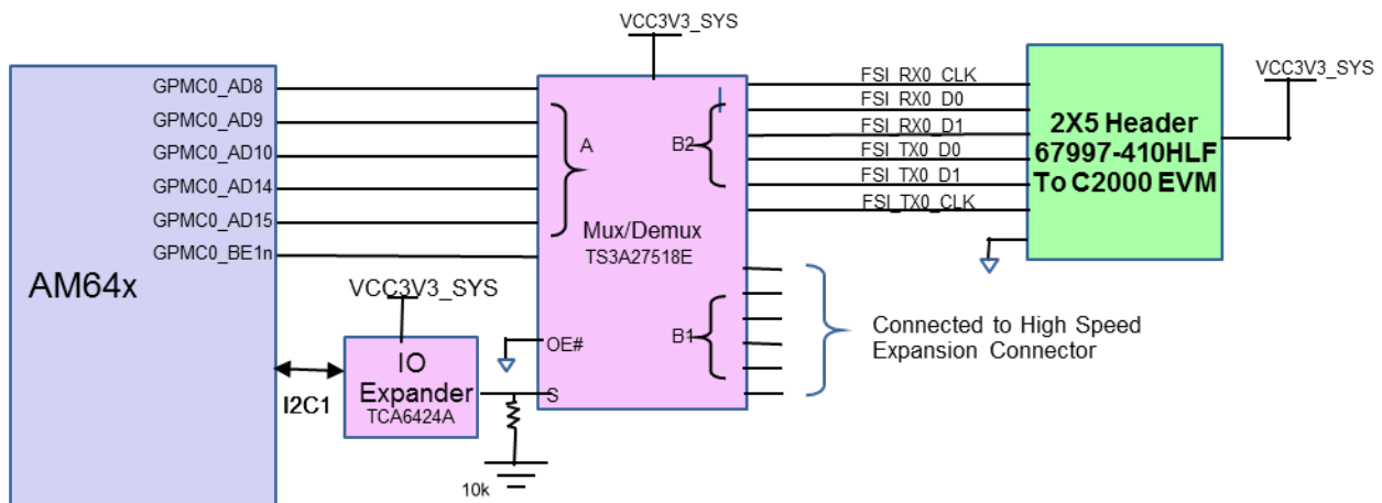
图 2-32. AM64x/AM243x FSI 接口
