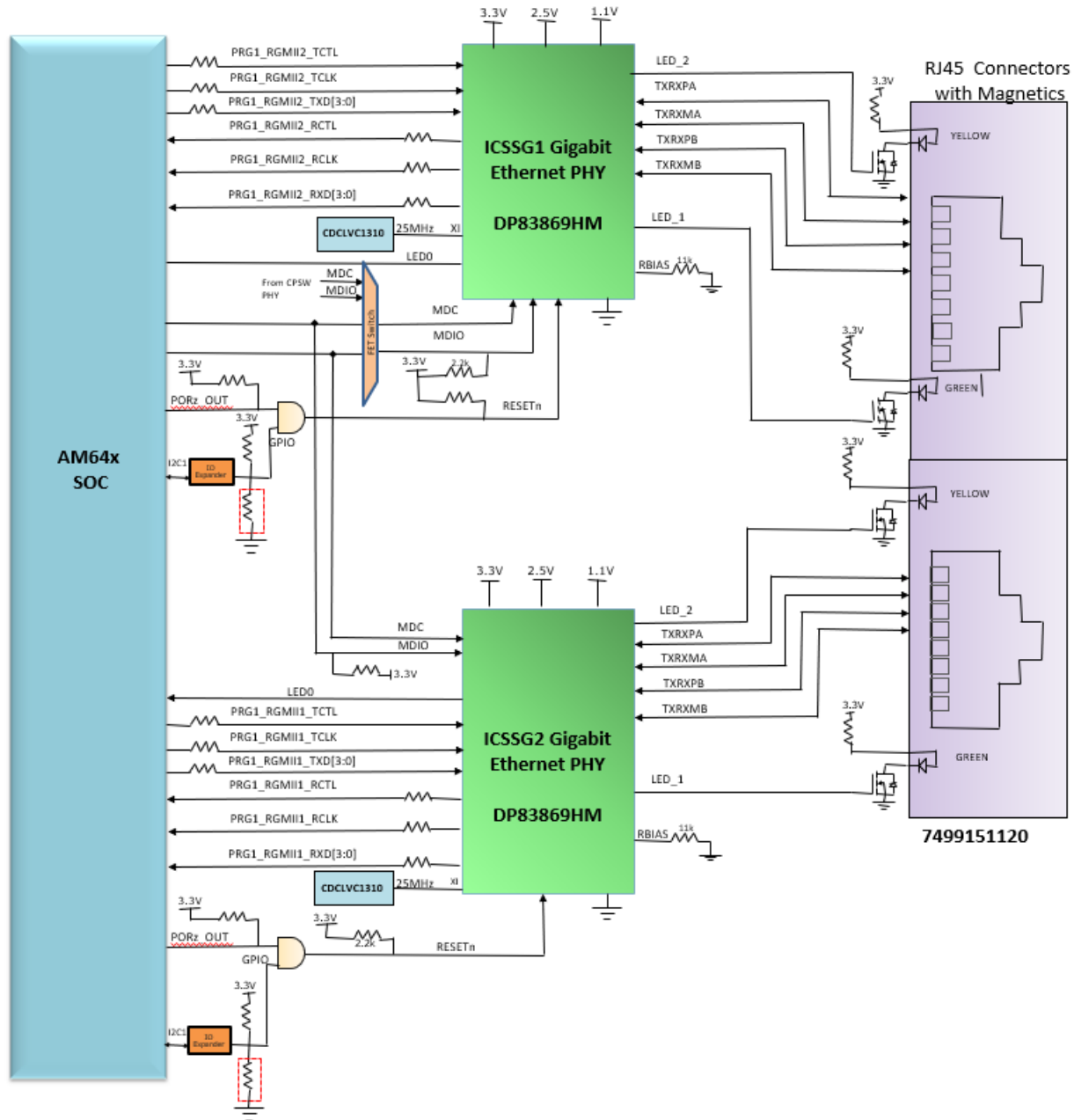
图 2-20. 以太网接口 - ICSSG 域
