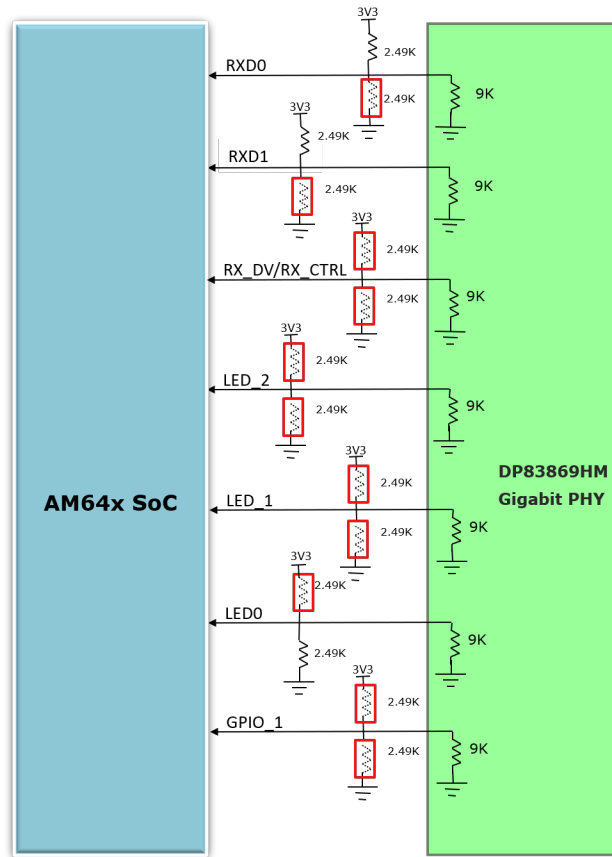
图 2-23. AM64x/AM243x 以太网接口 - ICSSG2 以太网自举设置
