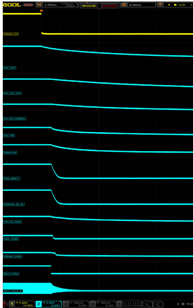
图 2-6. 断电序列
