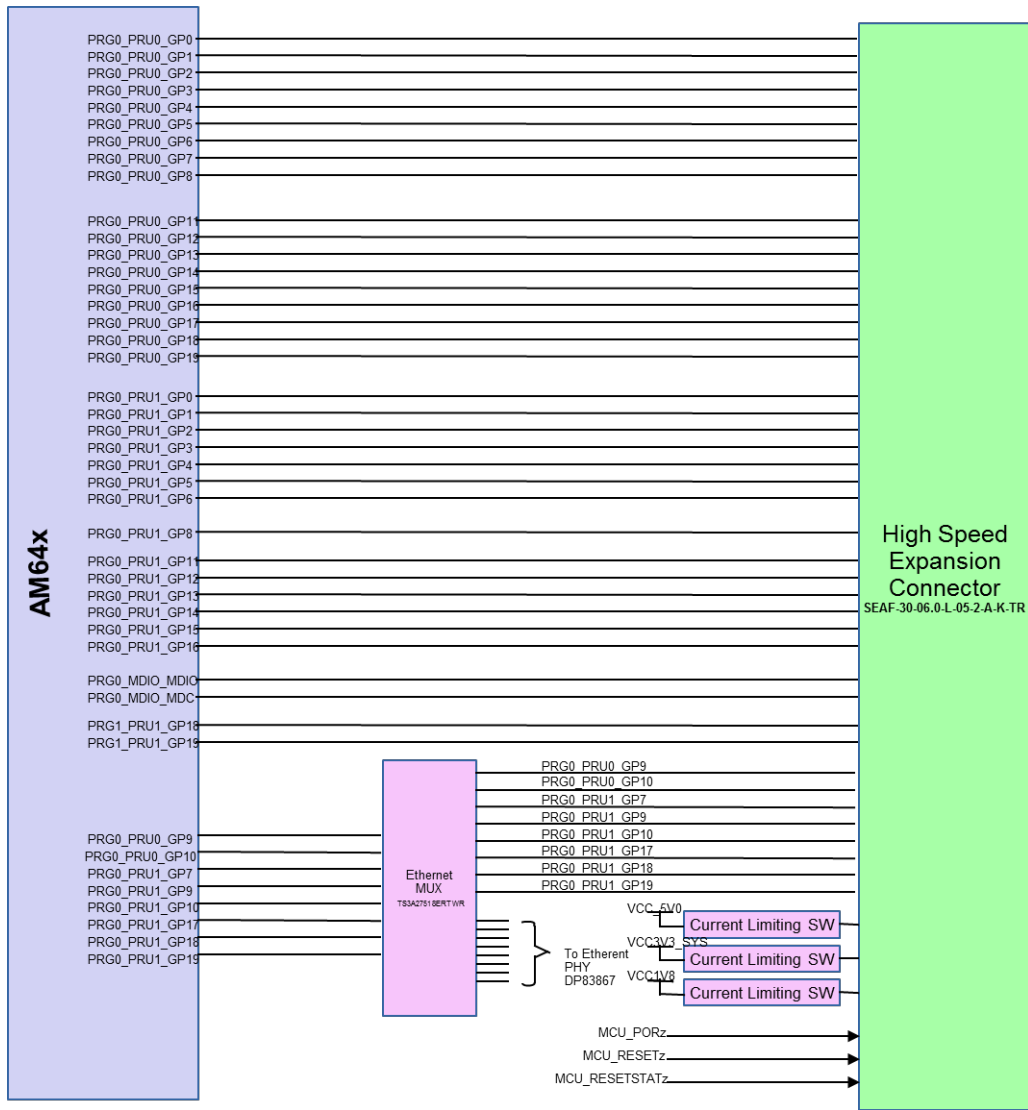
图 2-29. AM64x/AM243x 高速扩展连接器 - 第 2 部分
