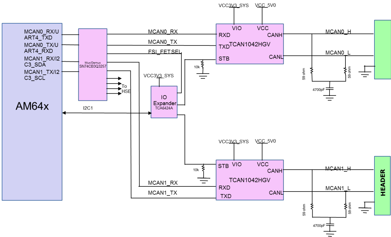
图 2-30. AM64x/AM243x CAN 接口
