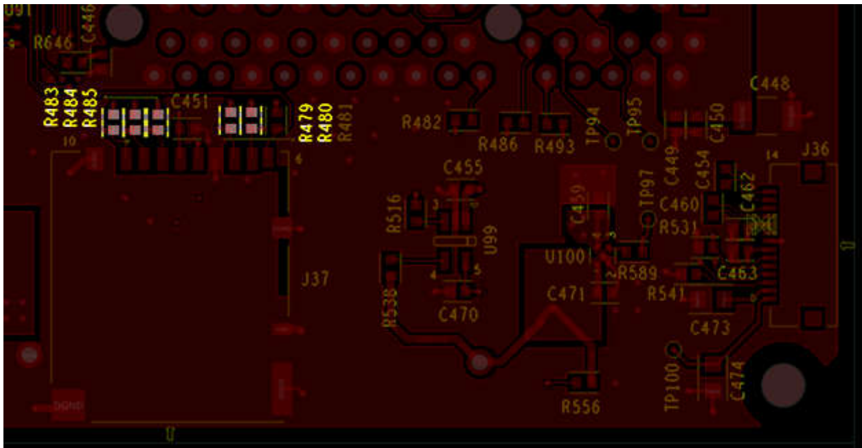
图 5-5. MMC1 布局
