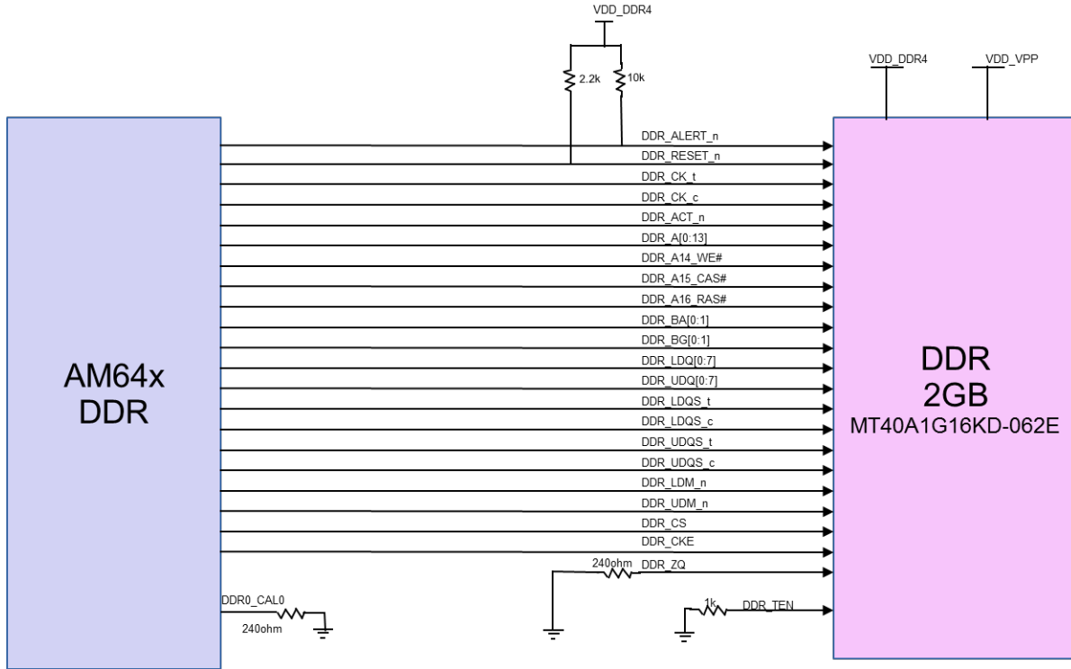
图 2-15. AM64x/AM243x DDR4 接口
