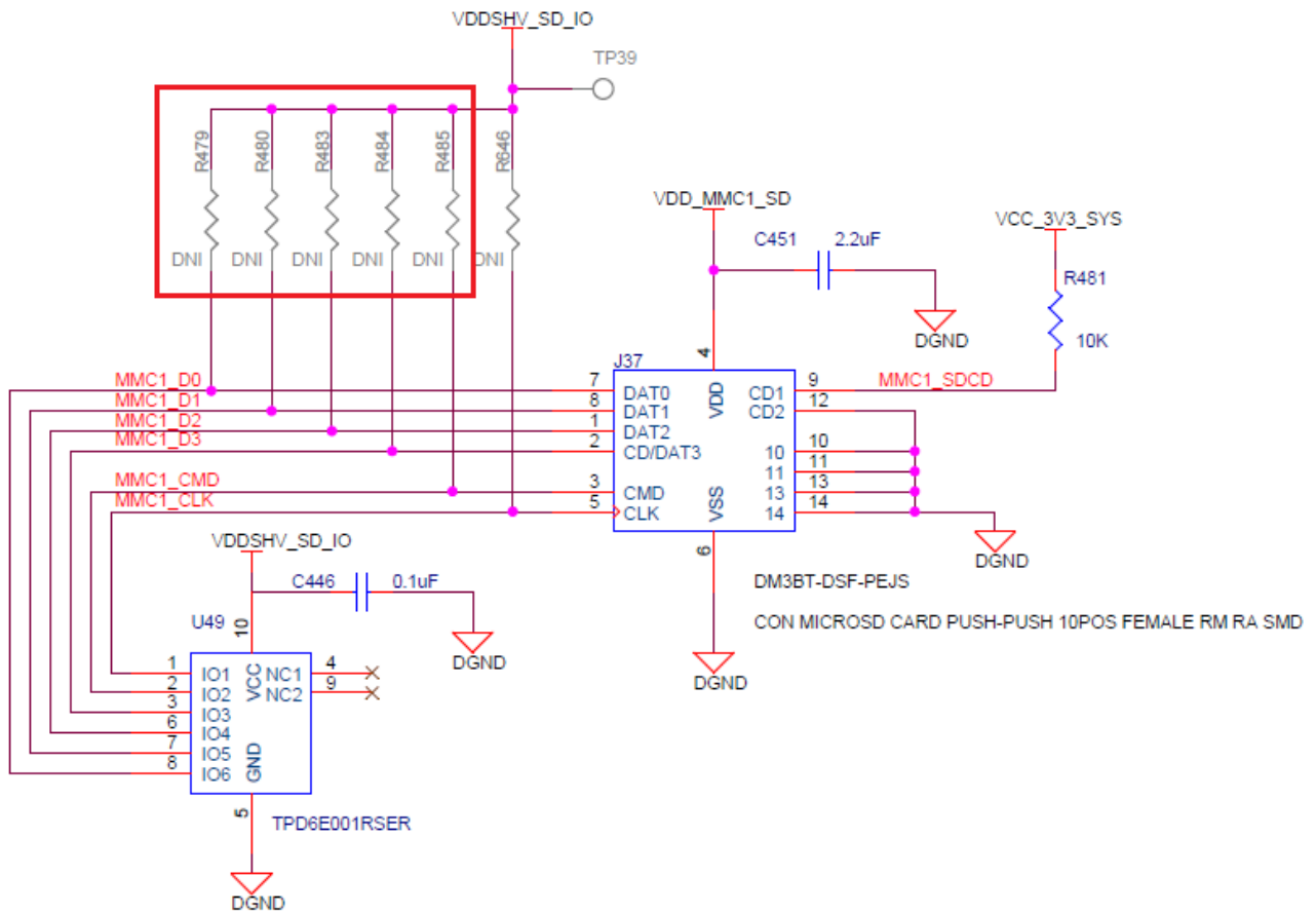
图 5-4. MMC1 原理图
