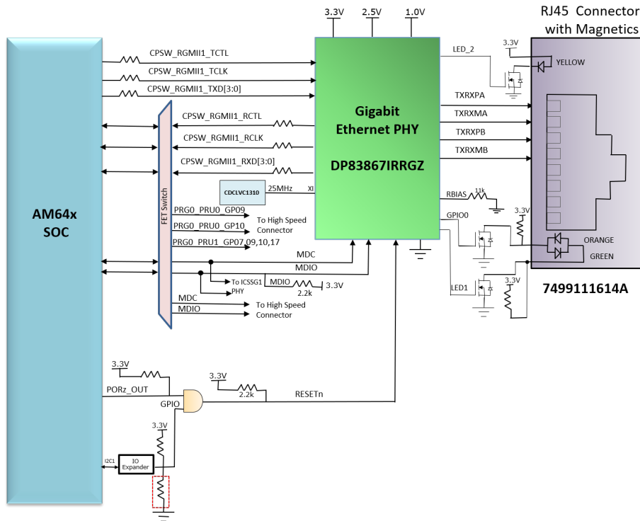
图 2-19. 以太网接口 - CPSW 域
