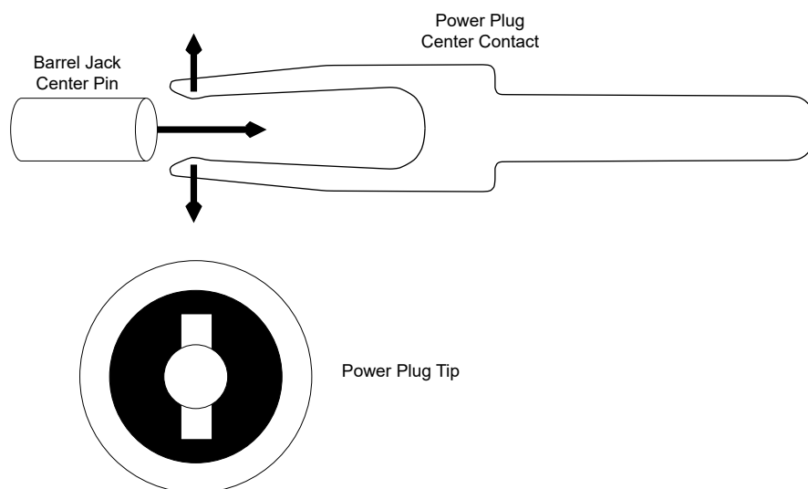
图 2-3. 带“调谐叉”中心触点的推荐电源插头图示
