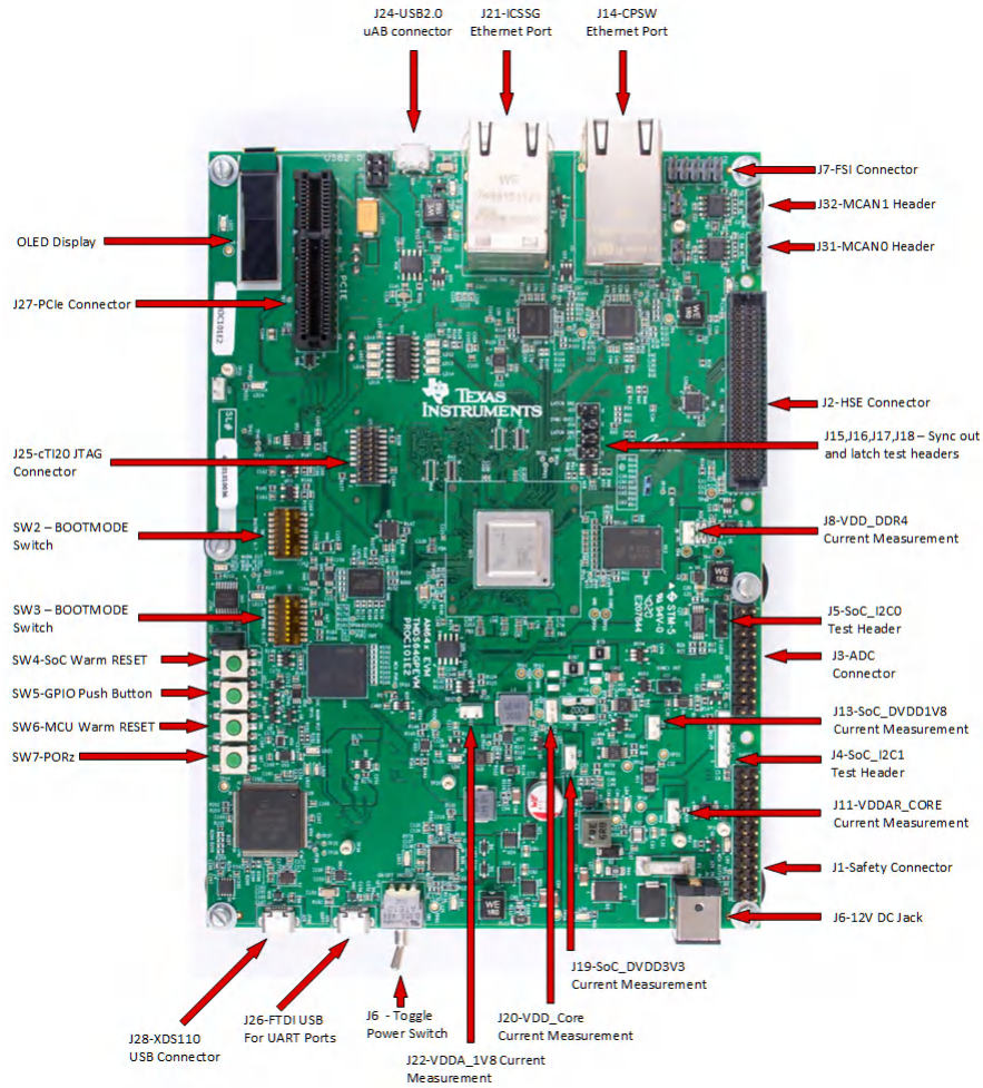
图 2-1. AM64x/AM243x EVM 板顶视图
