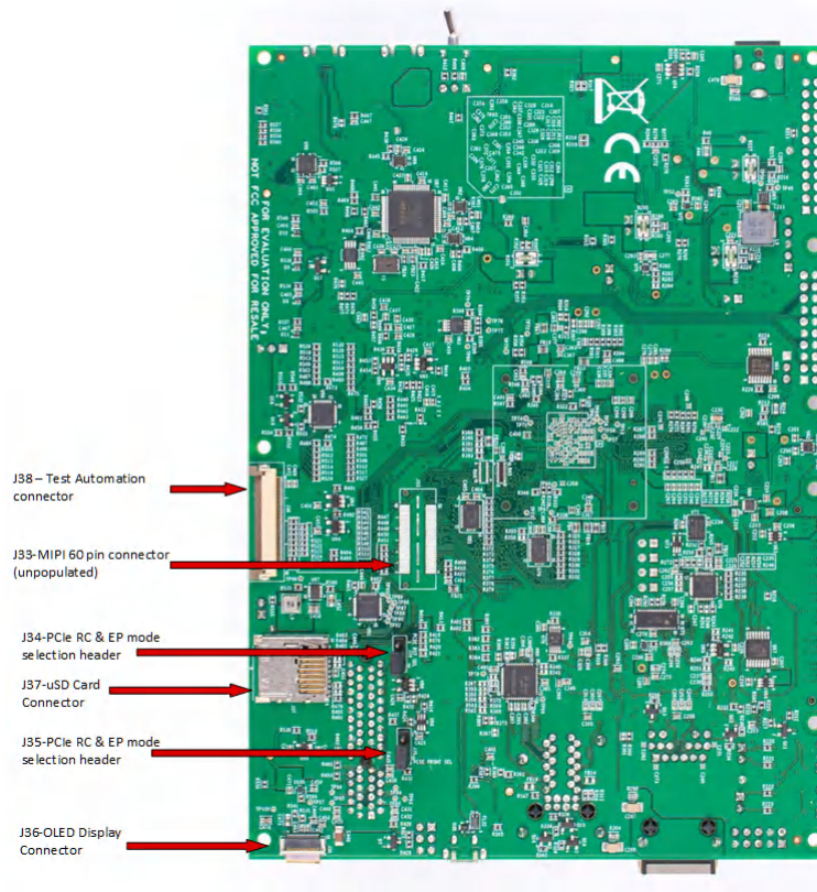
图 2-2. AM64x/AM243x EVM 板底视图
