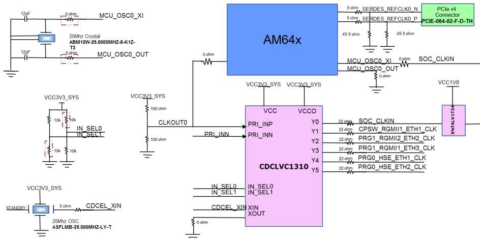
图 2-10. AM64x/AM243x EVM 时钟树
