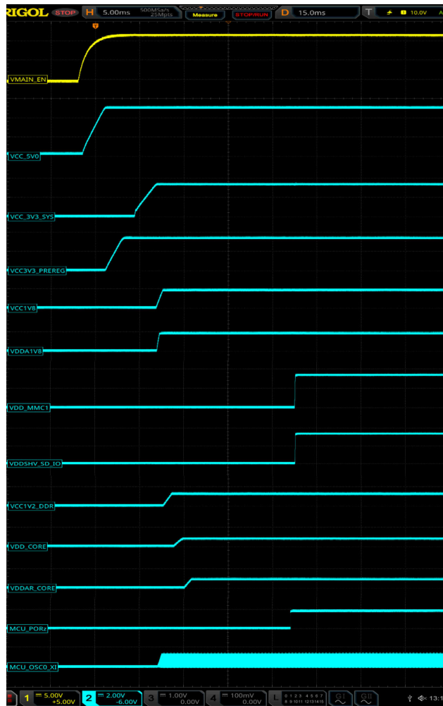
图 2-5. 上电序列
