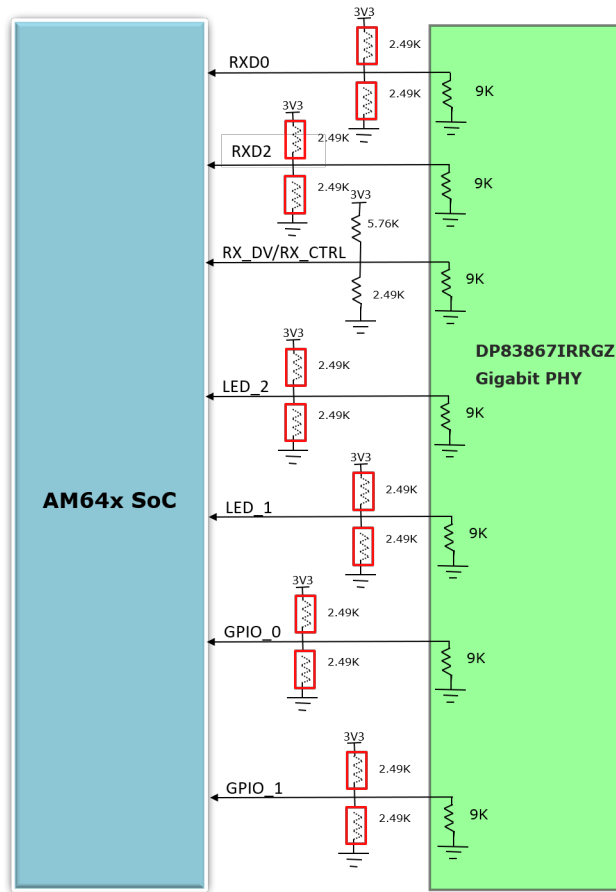
图 2-21. AM64x/AM243x 以太网接口 - CPSW 以太网自举设置
