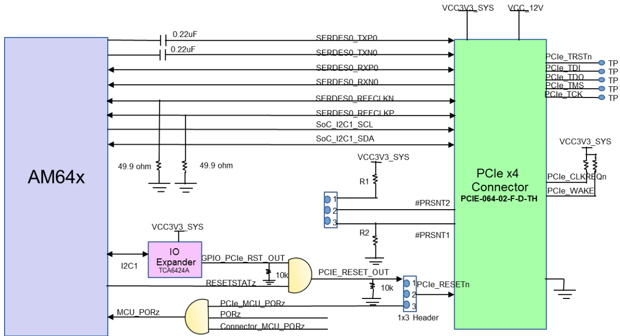
图 2-26. AM64x/AM243x PCIe 接口
