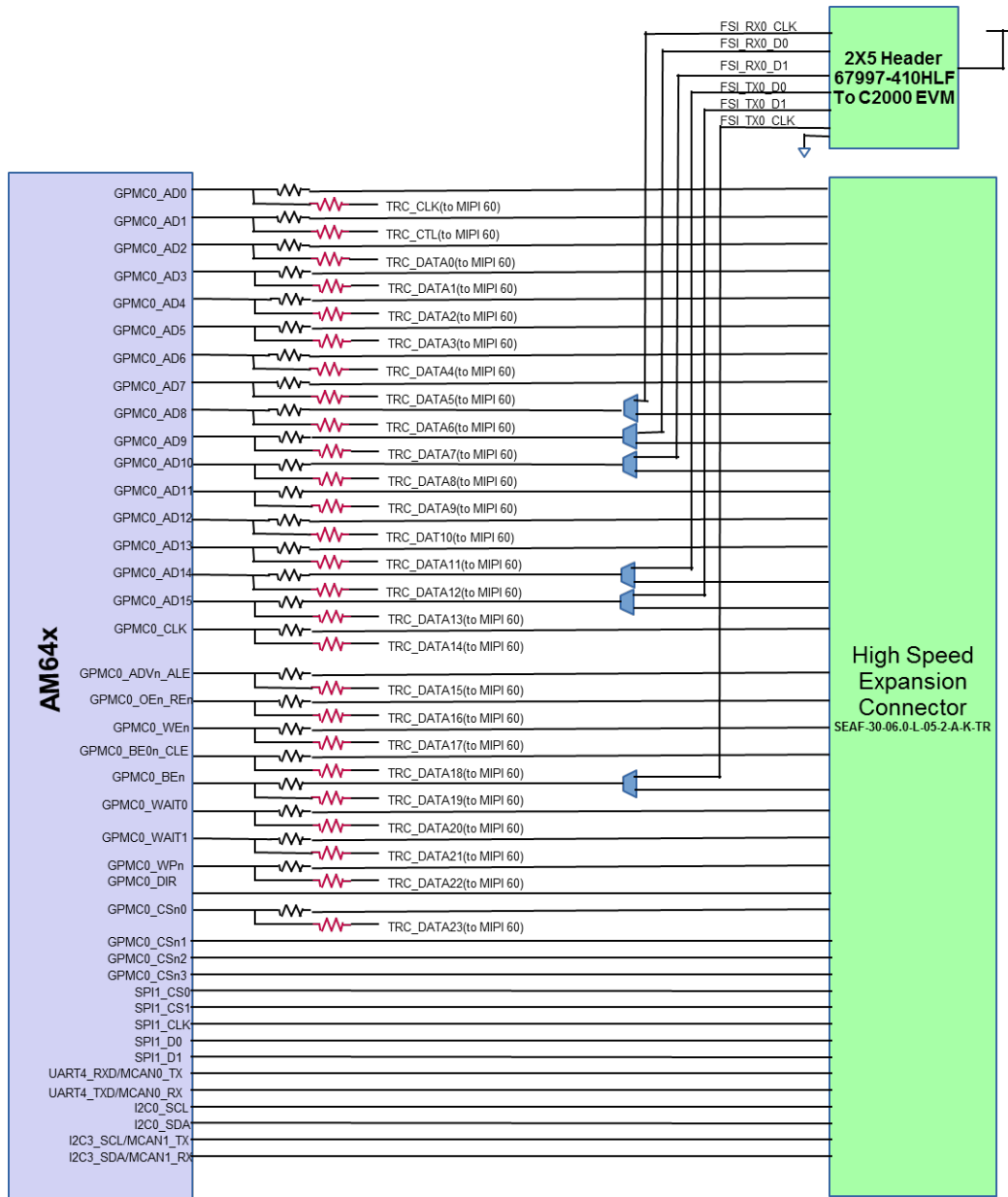
图 2-28. AM64x/AM243x 高速扩展连接器 - 第 1 部分
