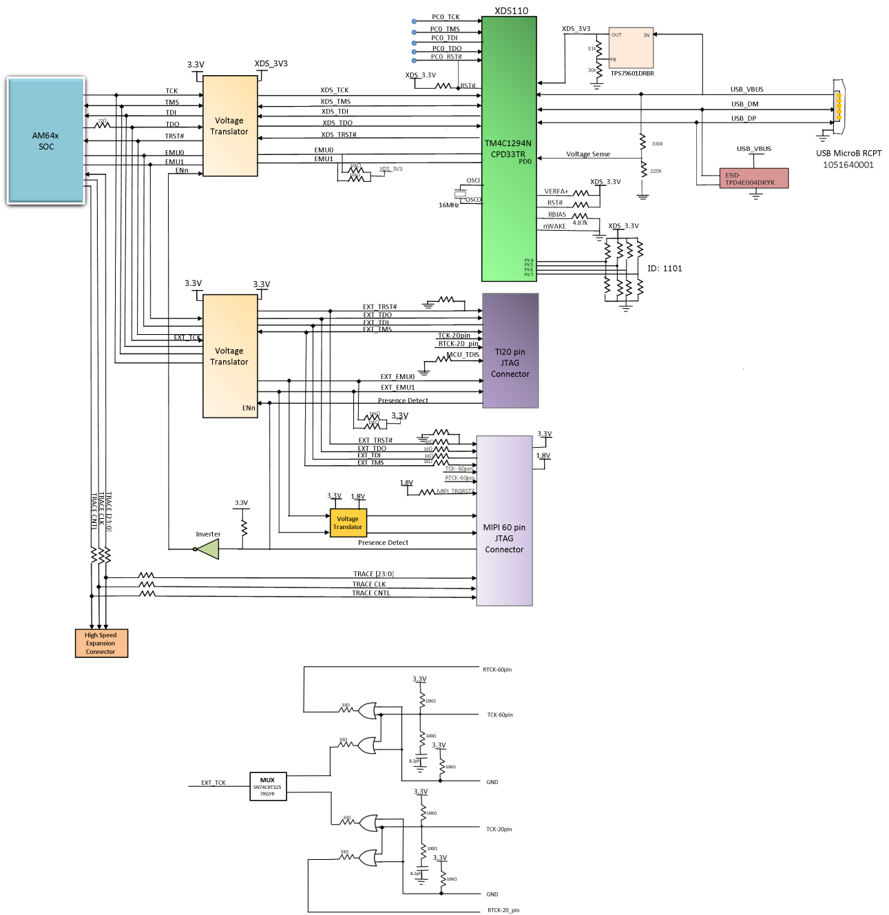
图 2-12. JTAG 接口
