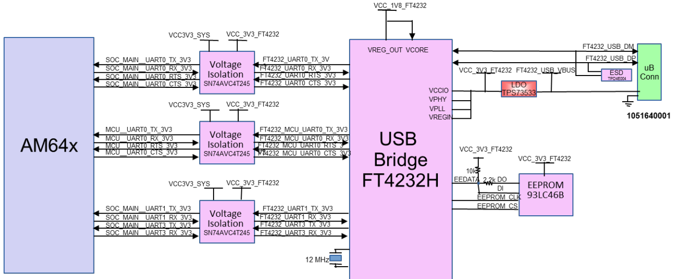
图 2-14. AM64x/AM243x UART 接口
