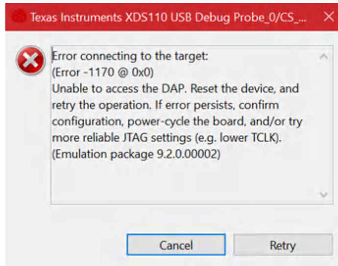
图 5-2. XDS110 CCS 连接错误对话框
