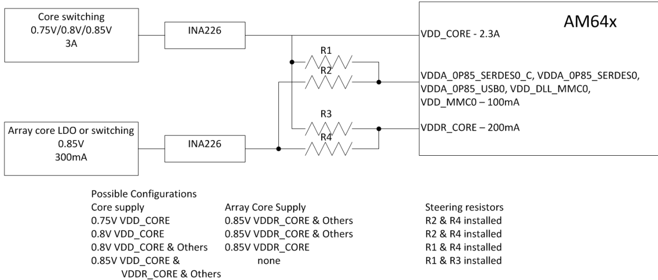
图 2-7. AM64x/AM243x 内核电源和阵列内核电源选项
