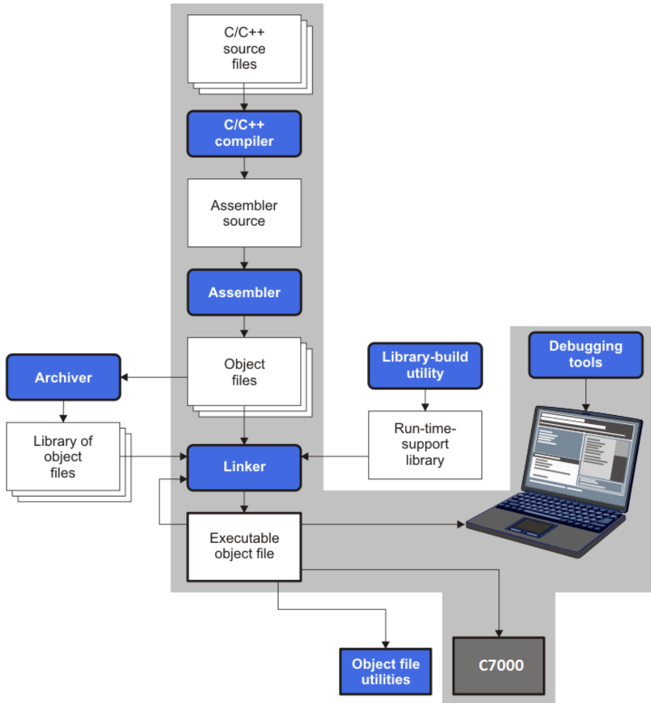
图 1-1. C7000 软件开发流程
