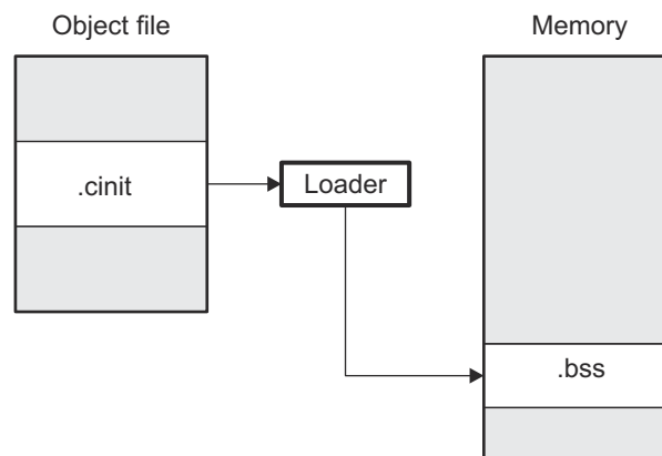
图 9-2. 加载时初始化
