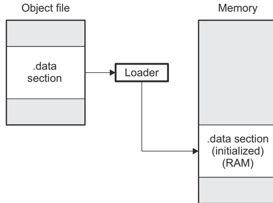
图 6-8. 加载时初始化
