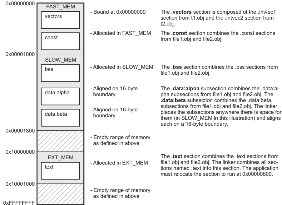
图 12-2. 由 SECTIONS 指令定义的段放置示例
