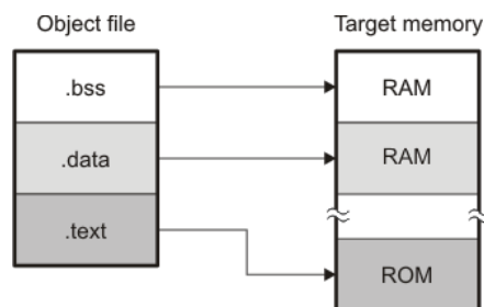
图 8-1. 存储器信息逻辑块分区
