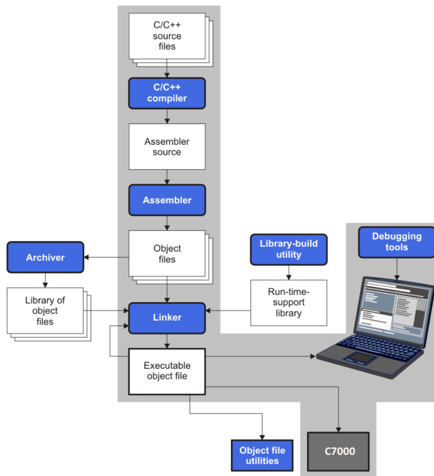
图 12-1. C7000 软件开发流程中的链接器
