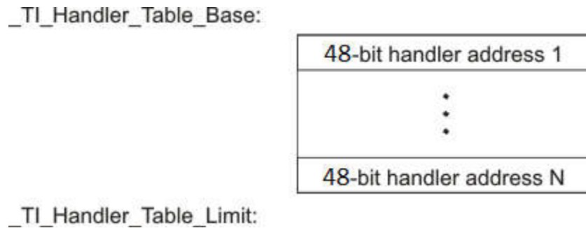
图 12-5. 处理程序表
