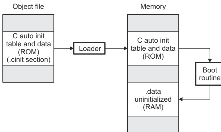
图 6-7. 运行时自动初始化
