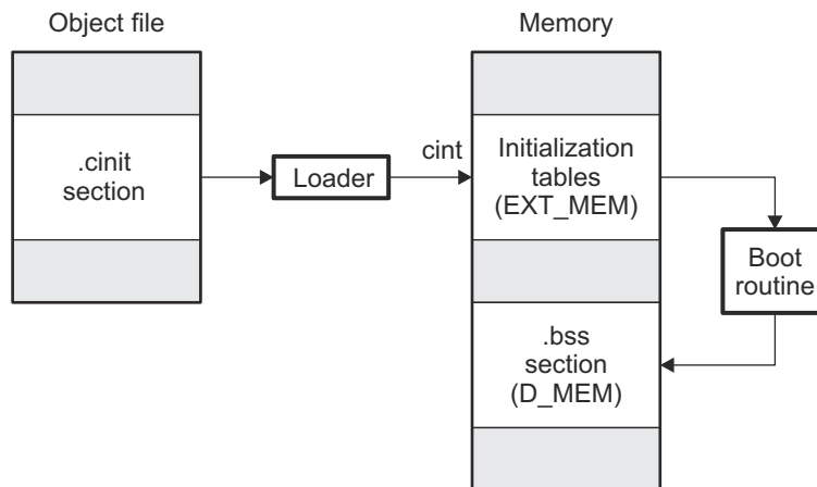
图 9-1. 运行时自动初始化
