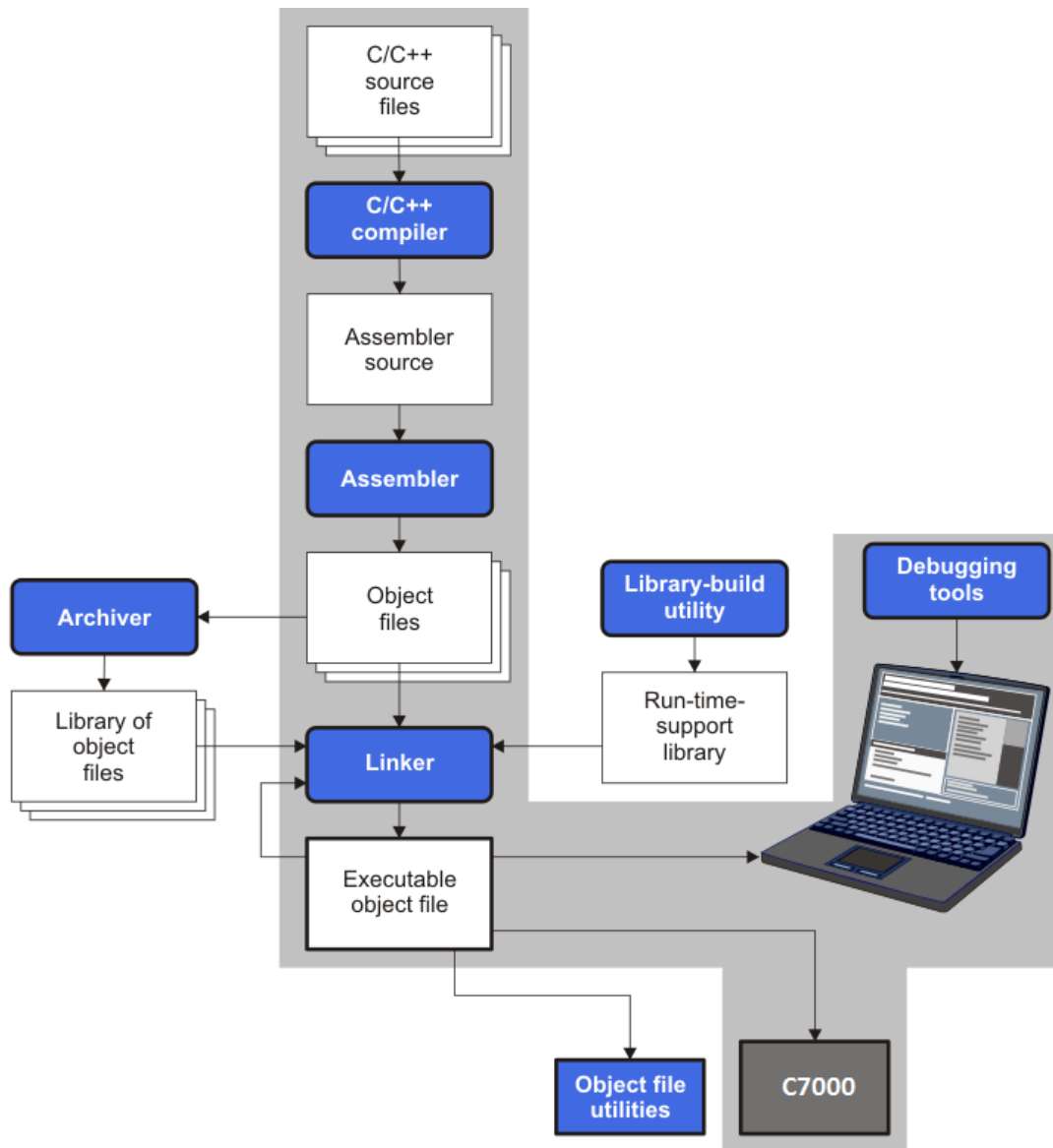
图 10-1. C7000 软件开发流程中的归档器
