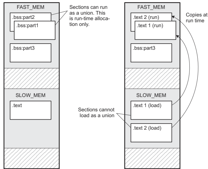
图 12-3. 存储器分配如 UNION 语句和 UNION 段的单独加载地址 所示
