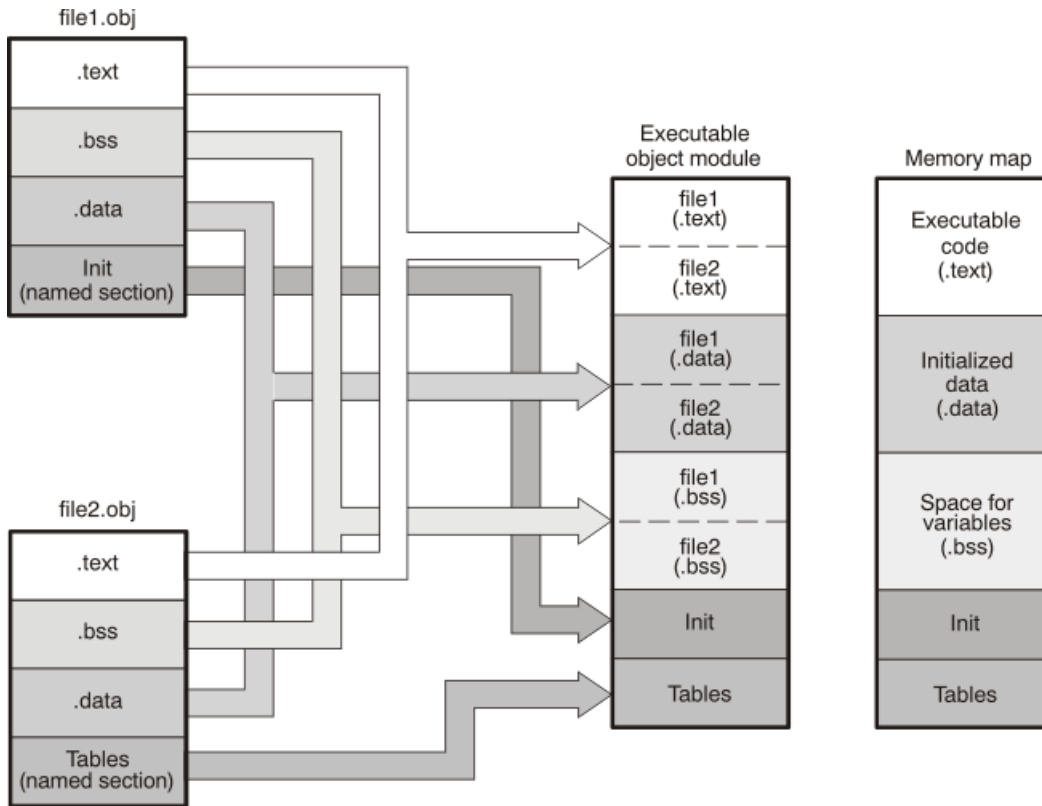
图 8-2. 组合输入段以构成可执行对象模块
