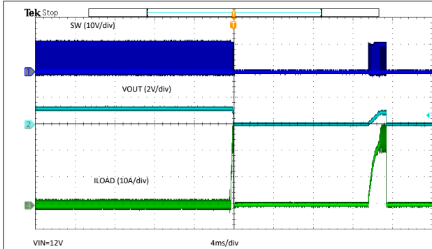
图 3-27. U1 输出过流保护 - 过载
