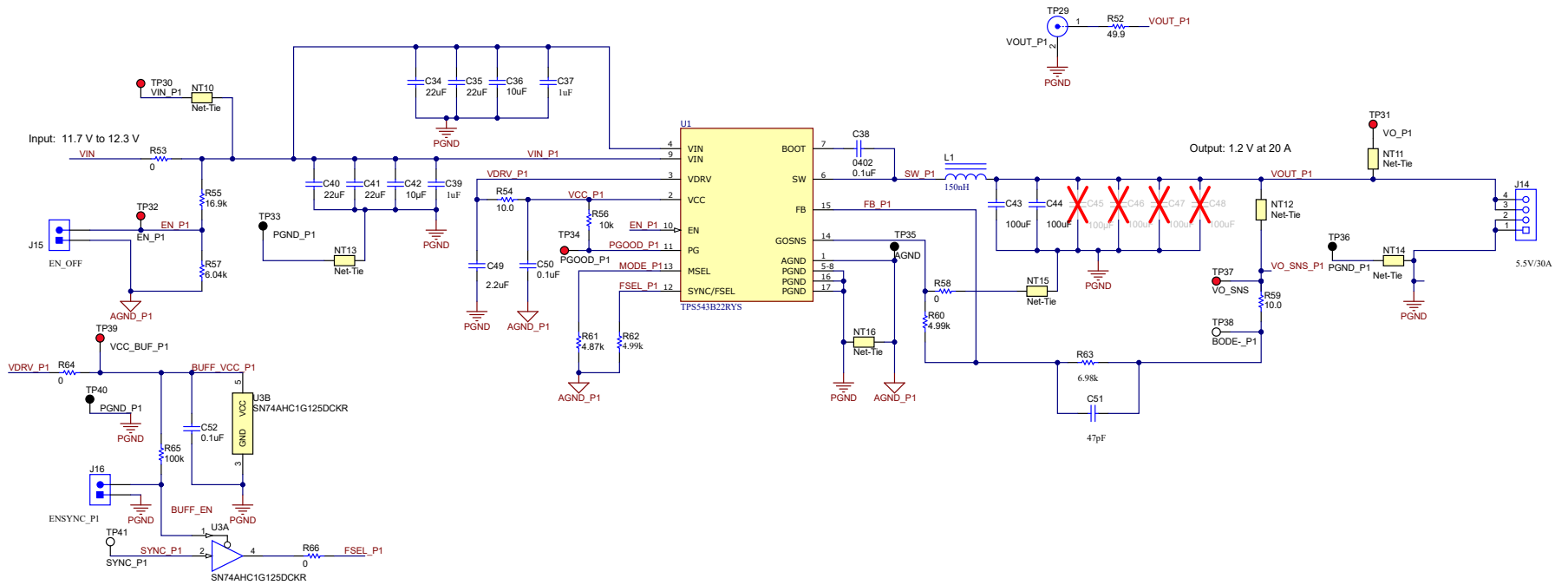
图 5-1. U1 原理图
