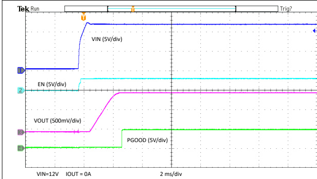
图 3-24. 通过 VIN 启动 U2
