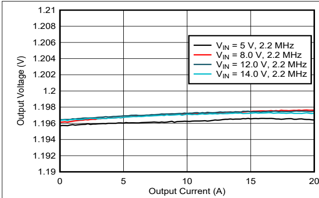
图 3-3. U1 负载调整率
