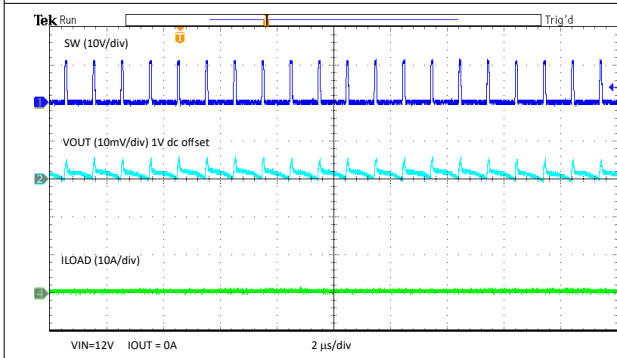
图 3-13. U2 输出纹波，空载
