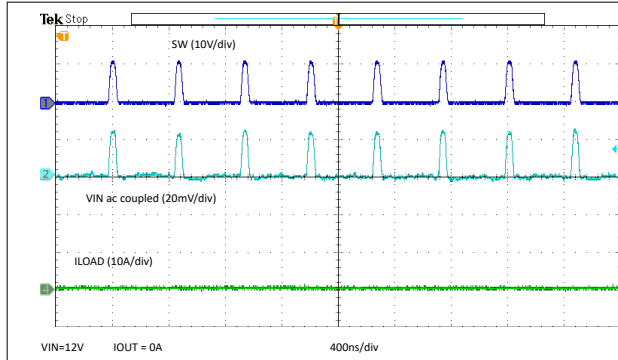
图 3-15. U1 输入纹波，空载
