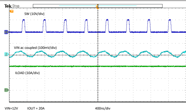
图 3-16. U1 输入纹波 - 20A 负载
