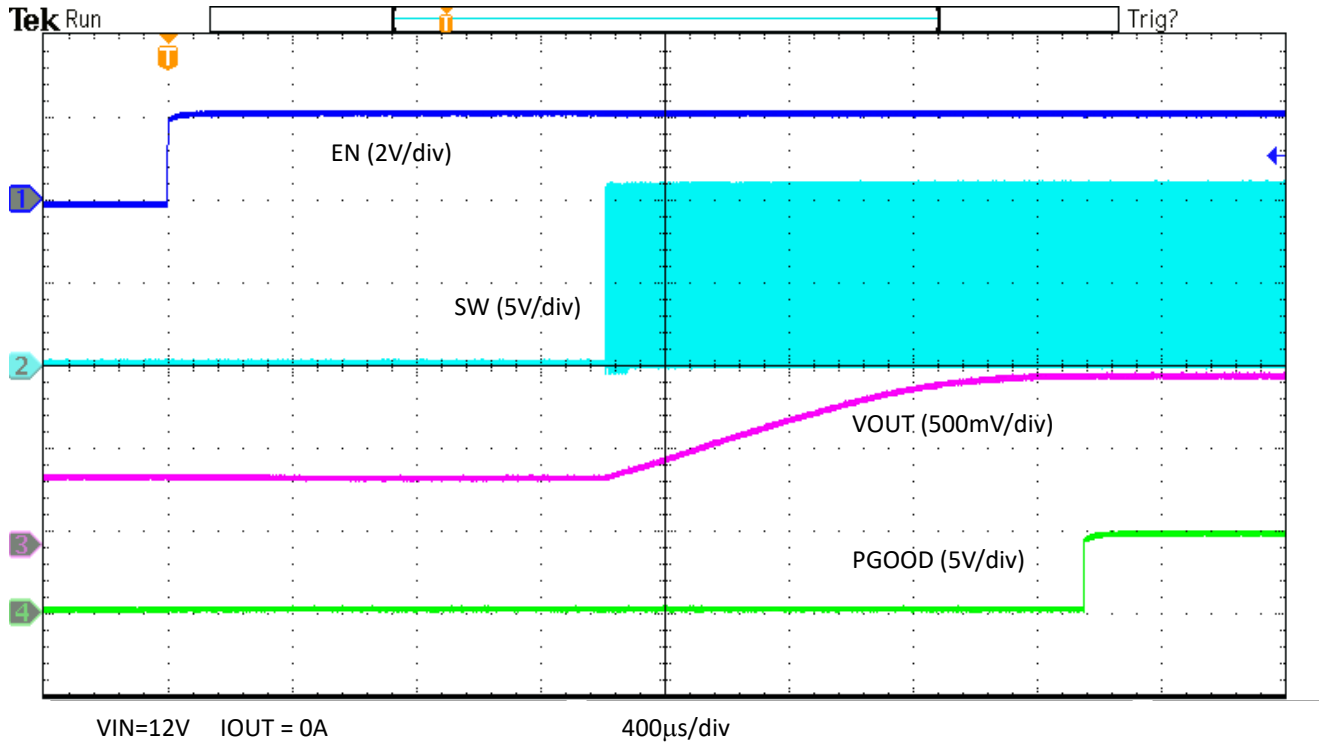
图 3-26. U2 启动至 0.5V 预偏置
