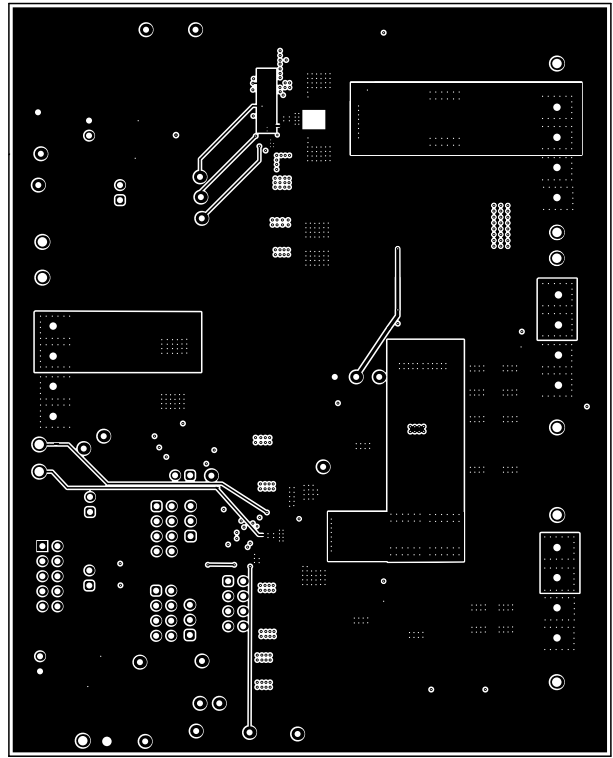
图 4-4. 信号 1
