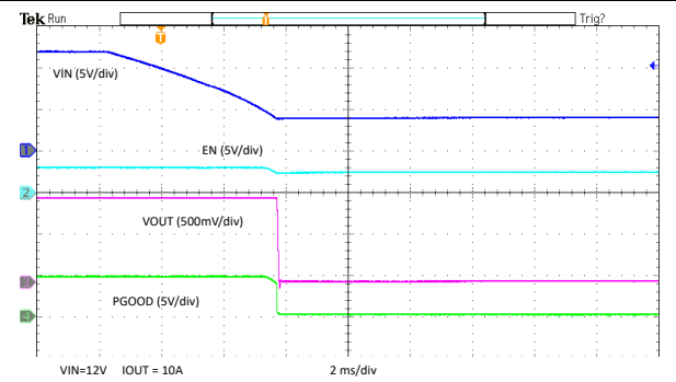
图 3-25. 通过 VIN 关断 U2
