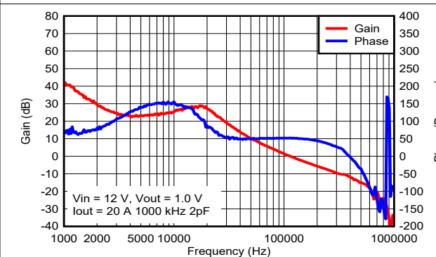
图 3-10. U2 波特图
