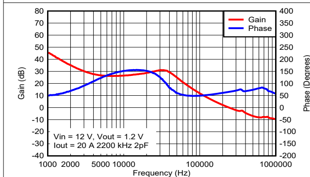
图 3-9. U1 波特图
