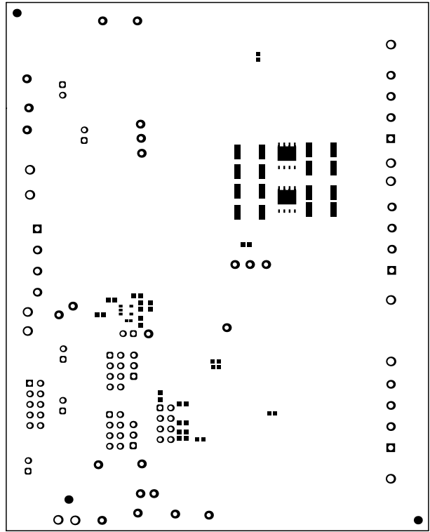
图 4-8. 底部阻焊层
