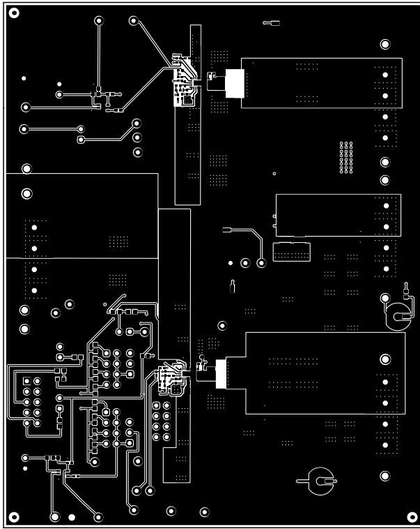
图 4-3. 顶层
