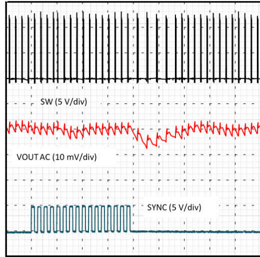
图 3-20. U2 时钟同步转换
