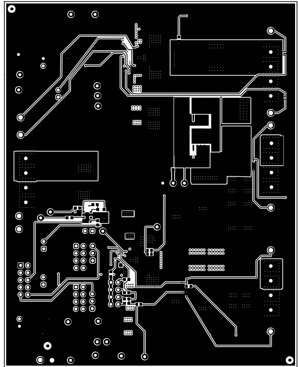
图 4-10. 底层
