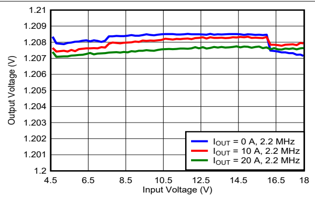
图 3-4. U1 线性调整率
