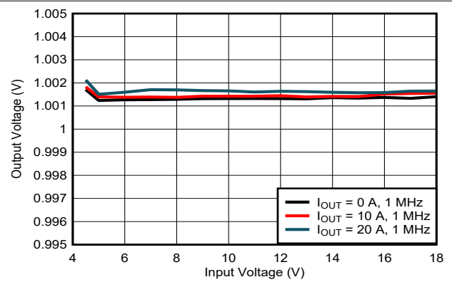
图 3-6. U2 线性调整率
