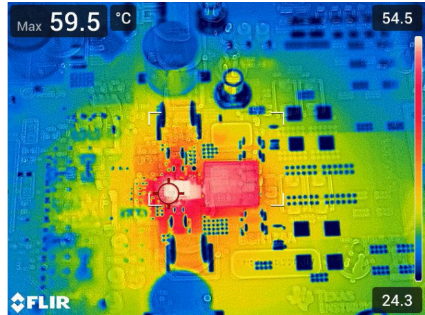
图 3-30. U2 热性能，20A 负载和 U1 关闭
