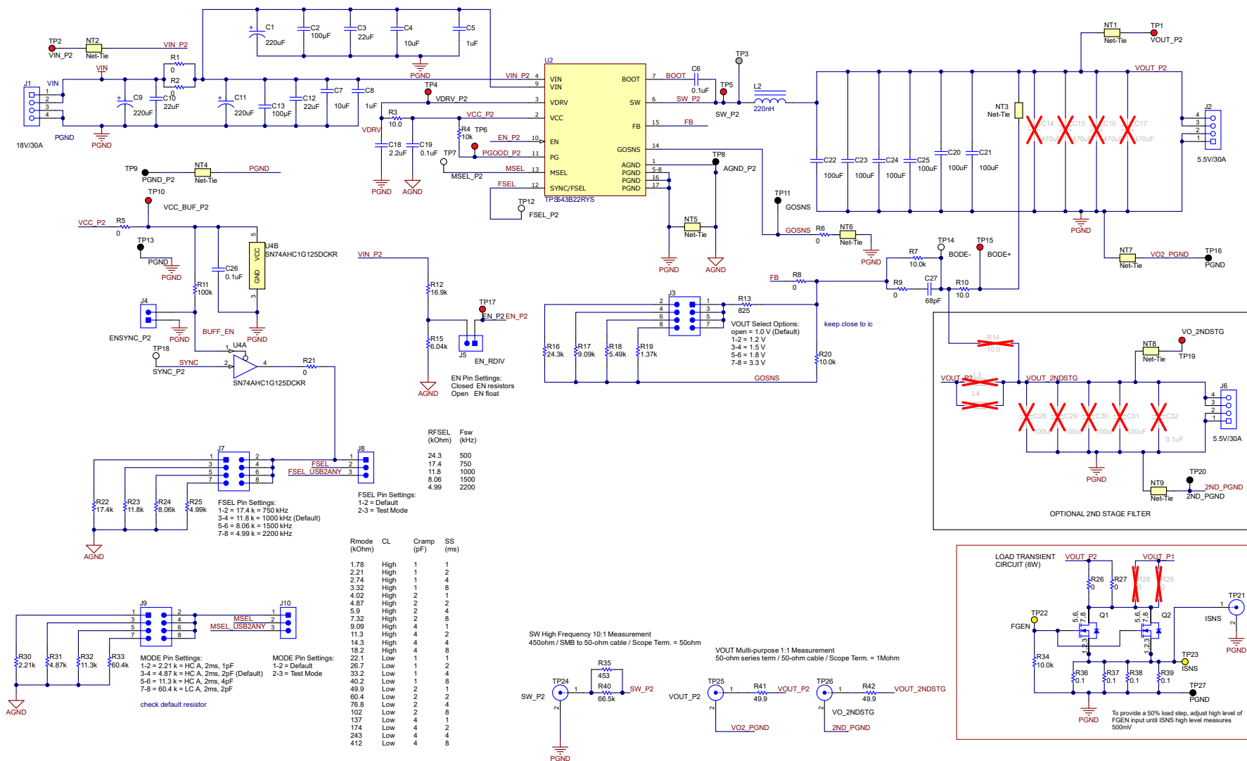
图 5-2. U2 原理图
