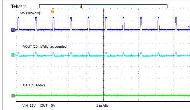
图 3-17. U2 输入纹波，空载
