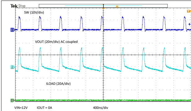
图 3-11. U1 输出纹波，空载
