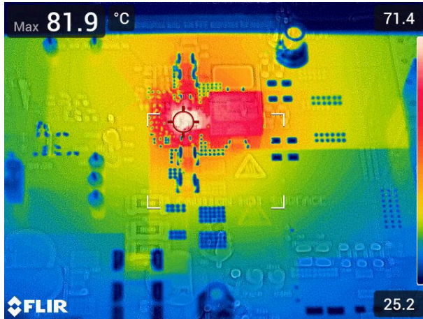
图 3-29. U1 热性能，20A 负载和 U2 关闭
