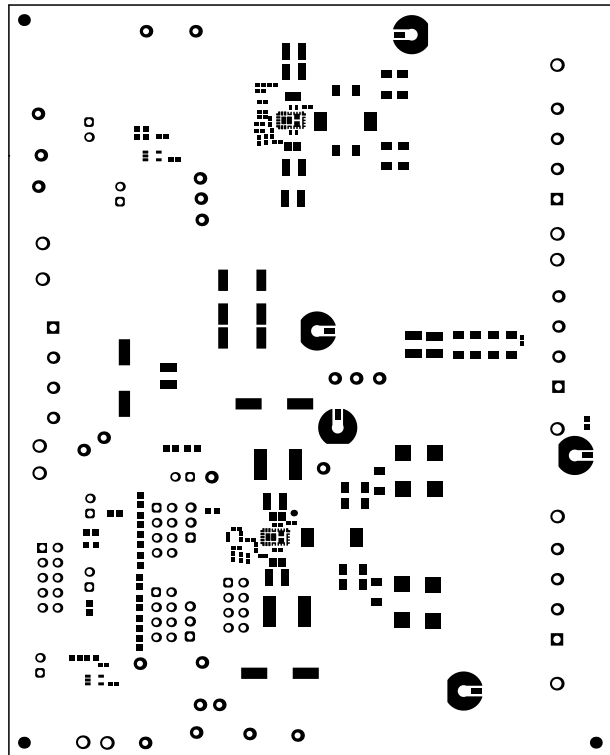
图 4-2. 顶部阻焊层
