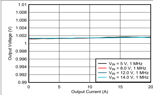
图 3-5. U2 负载调整率
