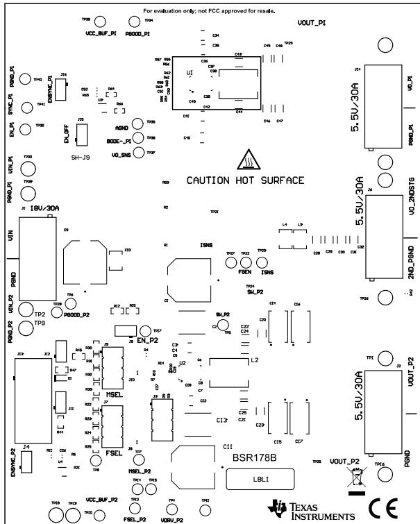
图 4-1. 顶部覆盖层
