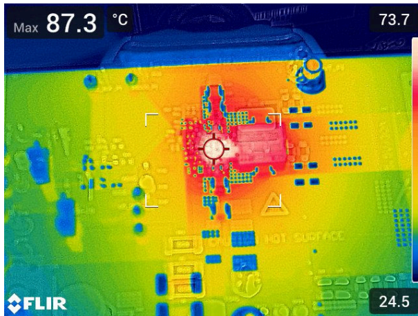
图 3-31. U1 热性能，两个 20A 负载
