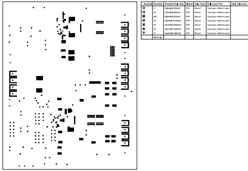
图 4-11. 钻孔图
