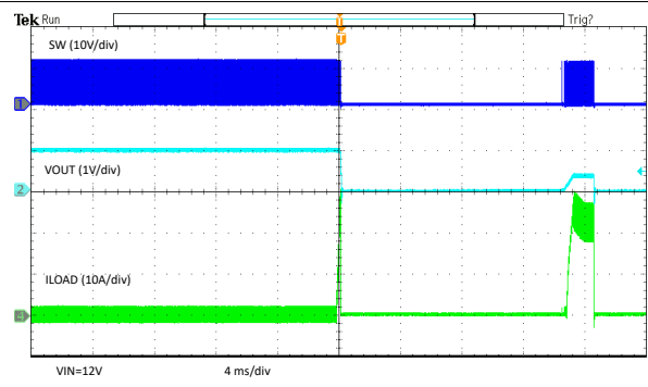
图 3-28. U2 输出过流保护 - 过载
