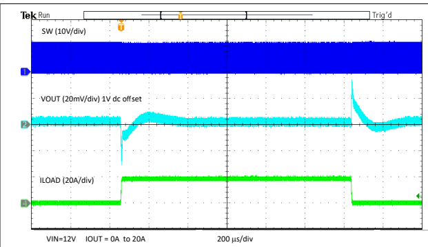
图 3-8. U2 瞬态响应
