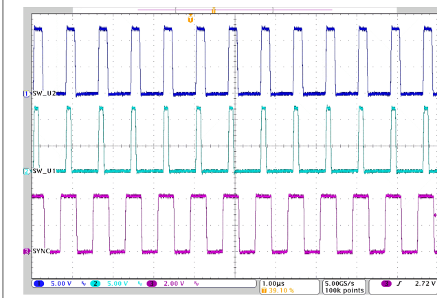
图 3-19. U1 和 U2 同步到时钟
