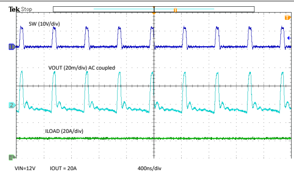
图 3-12. U1 输出纹波 - 20A 负载
