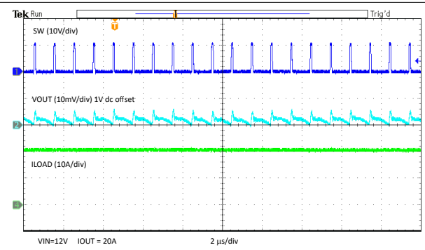
图 3-14. U2 输出纹波 - 20A 负载
