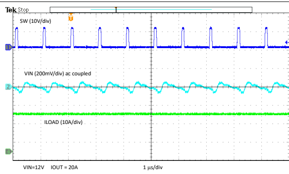
图 3-18. U2 输入纹波 - 20A 负载
