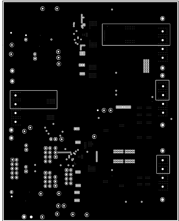
图 4-6. 信号 3
