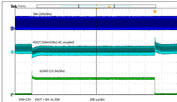
图 3-7. U1 瞬态响应
