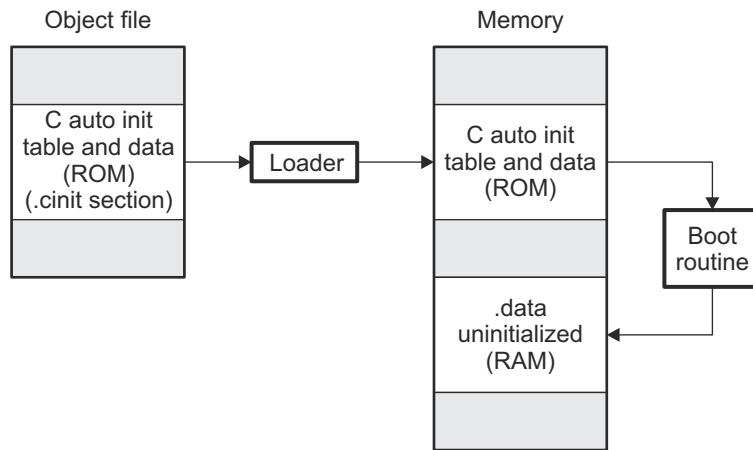
图 8-10. 运行时自动初始化
