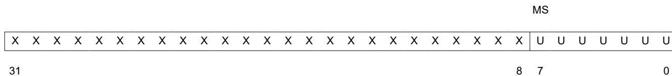
图 8-5. 无符号 40 位 __int40_t
