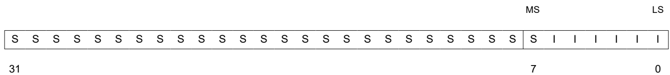
图 8-1. Char 和 Short 数据存储格式
