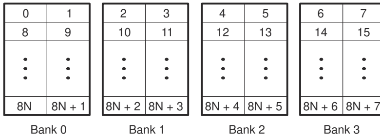
图 5-1. 4 组交错存储器
