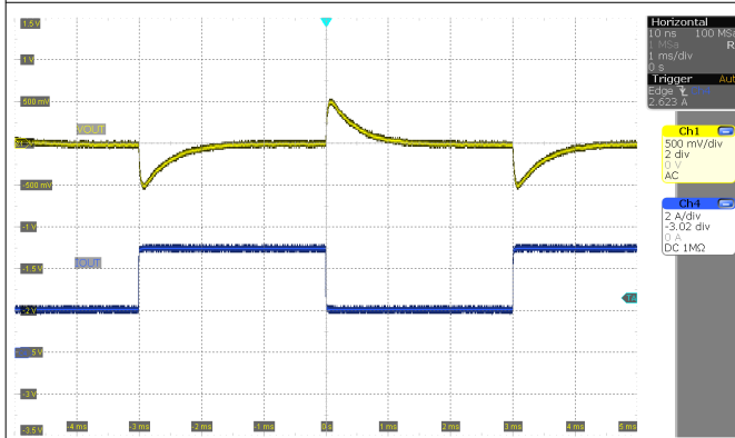
图 3-21. 负载阶跃 ( V_{IN} = 24V , I_{OUT} = 2A 至 5A )
