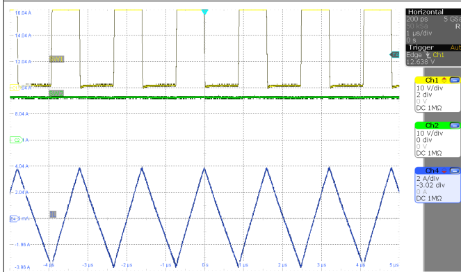
图 3-15. SW1、SW2、 I_L ( V_{IN} = 36V , I_{OUT} = 0A )
