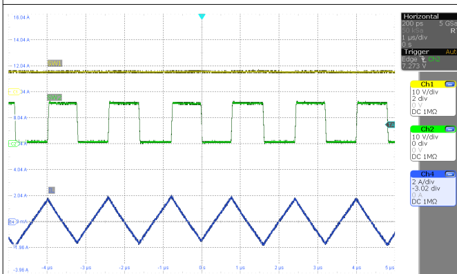
图 3-5. SW1、SW2、 I_L ( V_{IN} = 6V , I_{OUT} = 0A )
