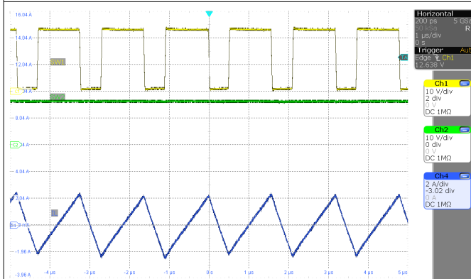
图 3-13. SW1、SW2、 I_L ( V_{IN} = 24V , I_{OUT} = 0A )
