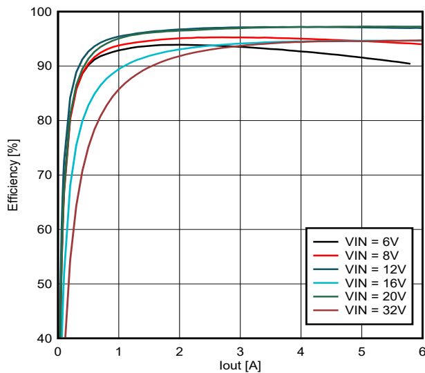
图 3-3. 效率与输出电流间的关系
