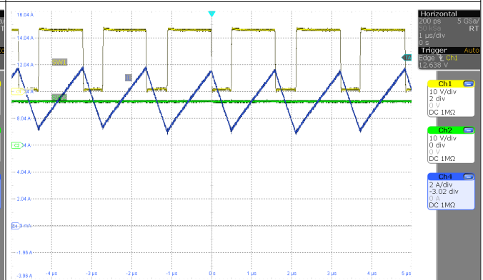
图 3-14. SW1、SW2、 I_L ( V_{IN} = 24V , I_{OUT} = 9.4A )
