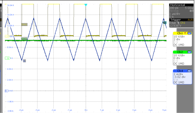
图 3-16. SW1、SW2、 I_L ( V_{IN} = 36V , I_{OUT} = 9.4A )
