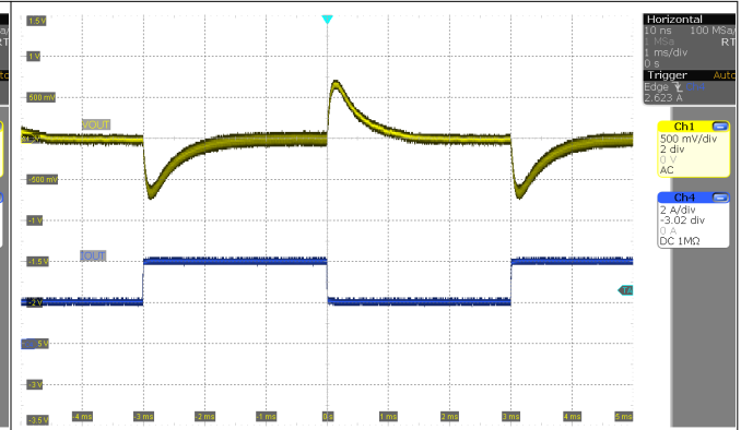
图 3-18. 负载阶跃 ( V_{IN} = 8V , I_{OUT} = 2A 至 4A )
