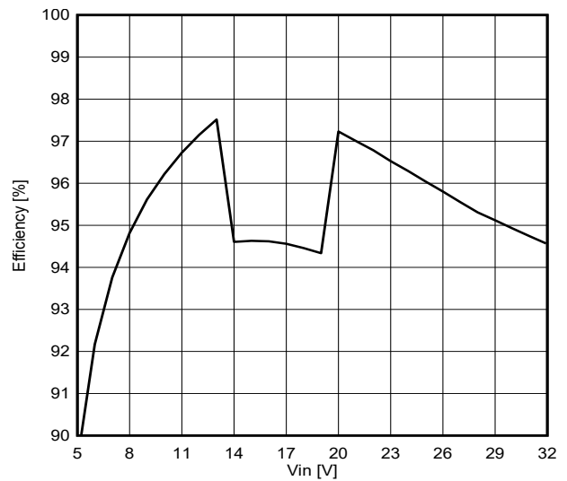
图 3-4. 效率与输入电压间的关系 ( I_{OUT} = 4.5A )
