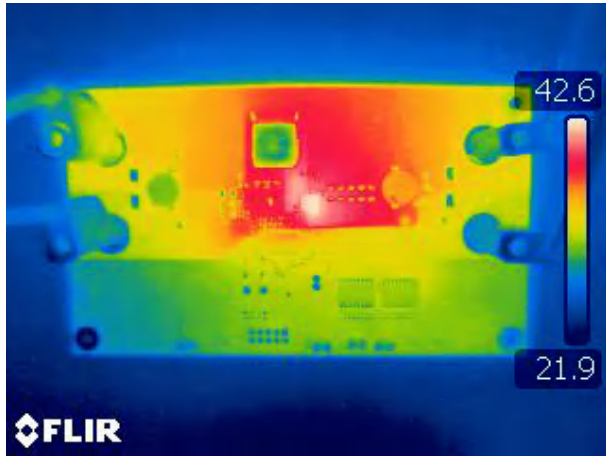
图 3-1. 热像图 : V_{IN} = 4.2V , I_{OUT} = 2.2A , 无强制空气冷却
