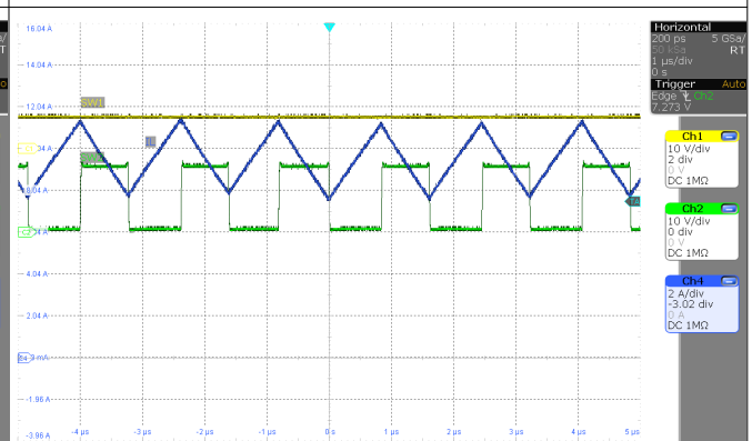
图 3-6. SW1、SW2、 I_L ( V_{IN} = 6V , I_{OUT} = 2A )
