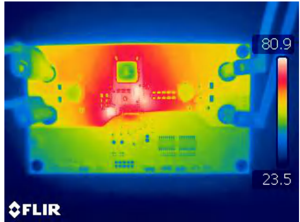
图 3-2. 热像图 : V_{IN} = 16V , I_{OUT} = 9.4A , 无强制空气冷却
