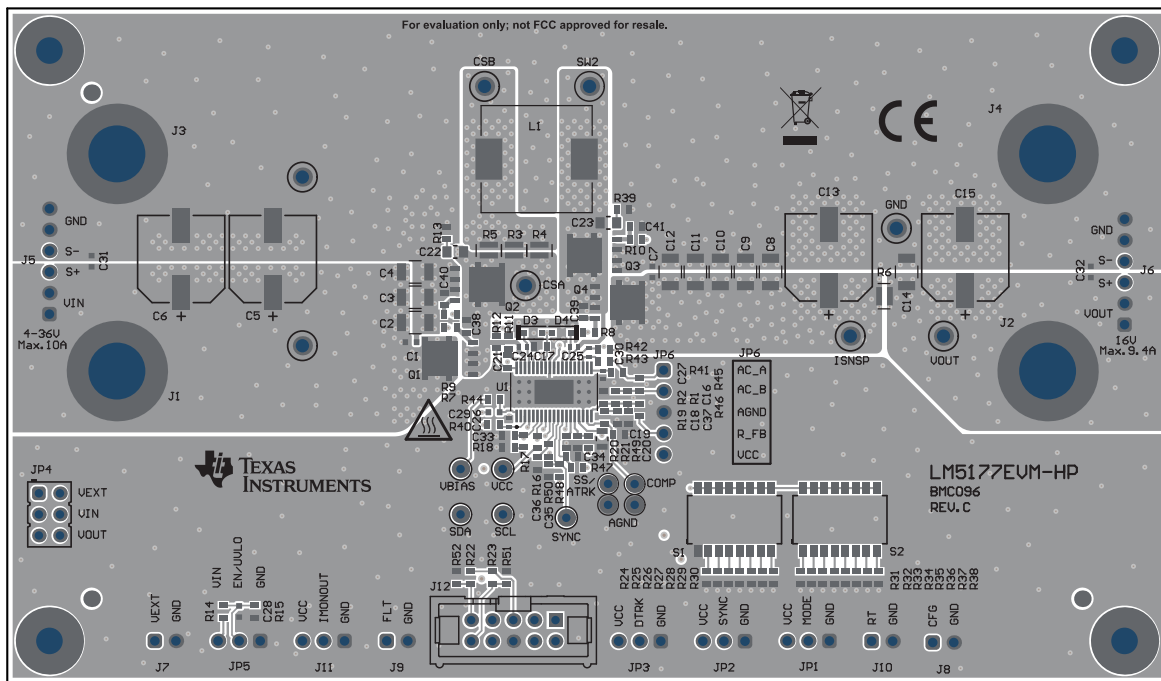
图 4-2. 顶部丝印
