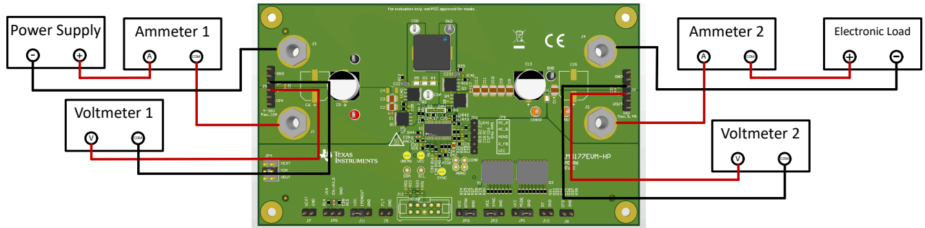
图 2-4. 典型的 EVM 连接图
