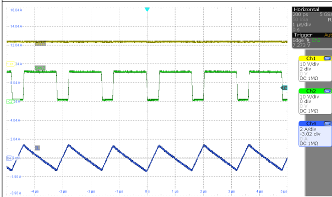
图 3-9. SW1、SW2、 I_L ( V_{IN} = 12V , I_{OUT} = 0A )
