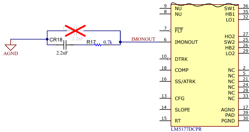
图 2-2. 用于电流限制的 IMONOUT 组件
