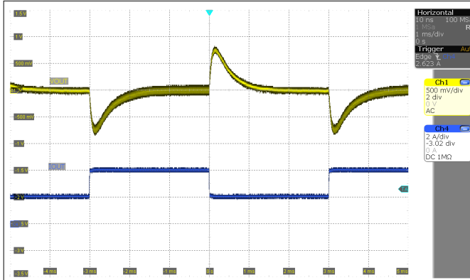
图 3-17. 负载阶跃 ( V_{IN} = 7V , I_{OUT} = 2A 至 4A )
