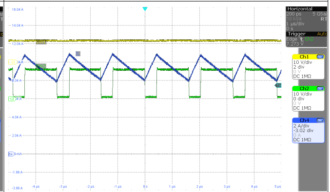
图 3-10. SW1、SW2、 I_L ( V_{IN} = 12V , I_{OUT} = 6.8A )
