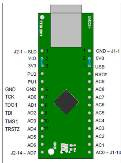
图 3-27. UM232H 模块
