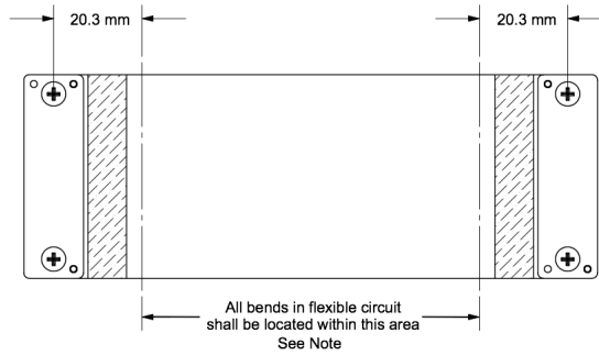
图 1-7. 柔性电缆图
