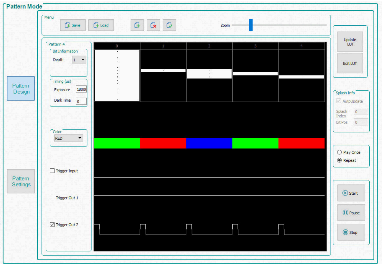
图 3-15. DMD 块加载图形序列
