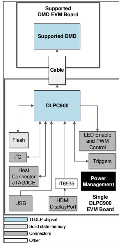
图 1-1. DLP LightCrafter 单 DLPC900 硬件元件
