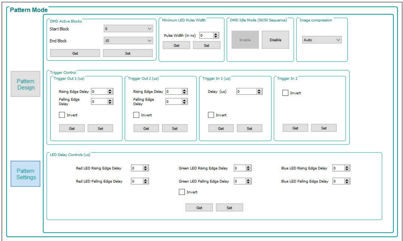
图 3-16. 模式设置面板
