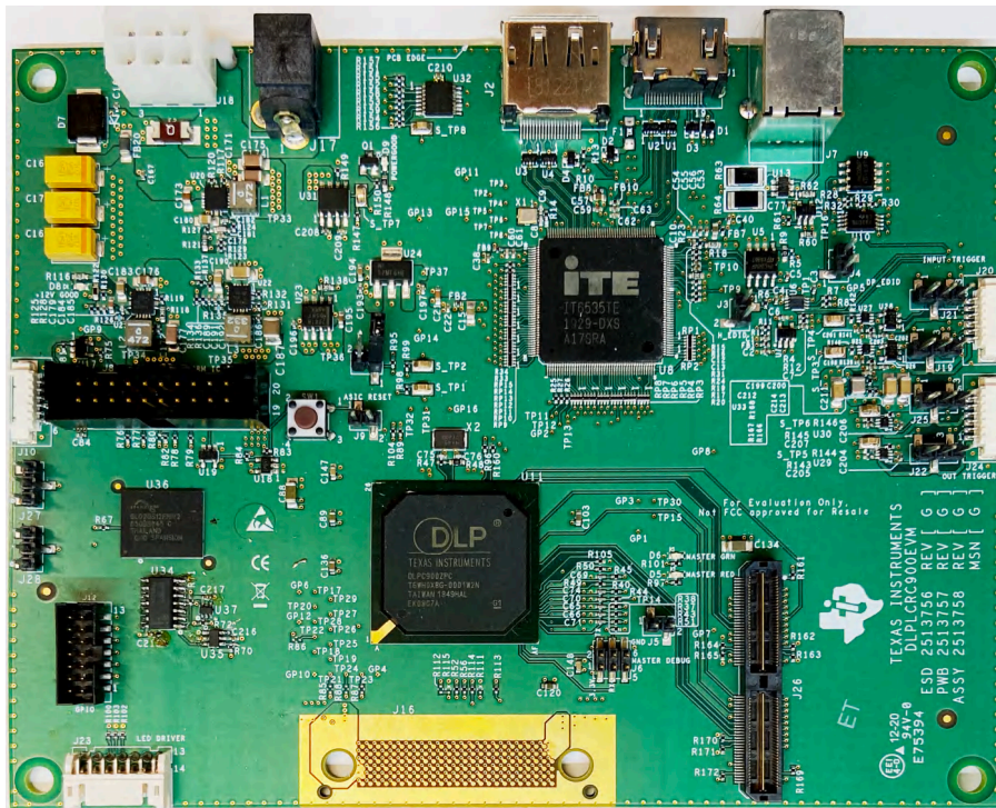
图 1-1. DLP LightCrafter 单 DLPC900 评估模块
