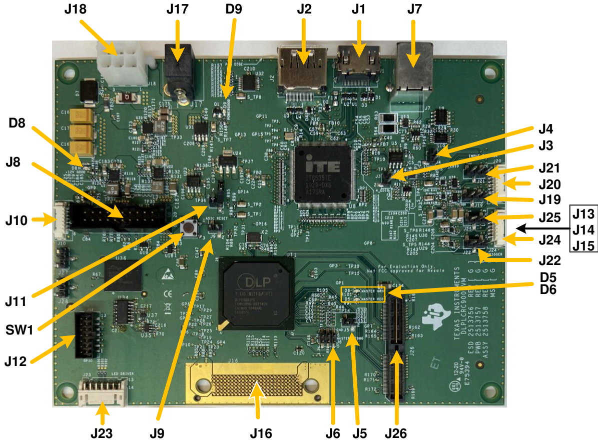
图 1-3. DLP LightCrafter 单 DLPC900 EVM 连接器 (顶视图)
