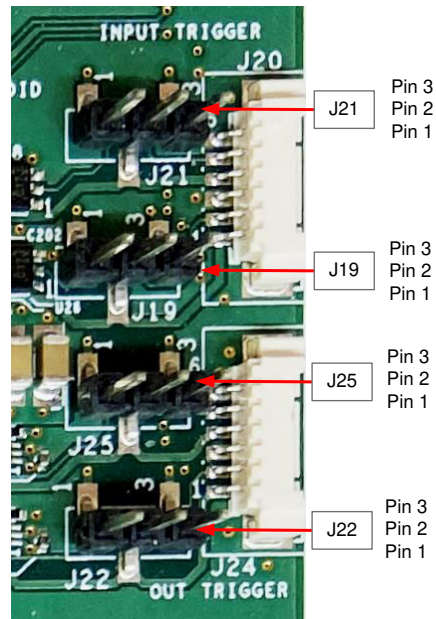
图 1-6. DLP LightCrafter 单 DLPC900 EVM 触发电压电平选择器
