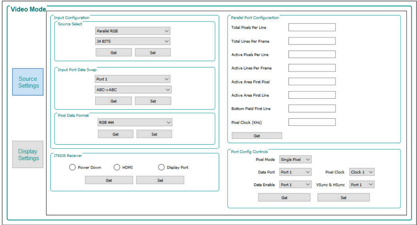
图 3-4. 视频模式面板 - 源设置选项卡
