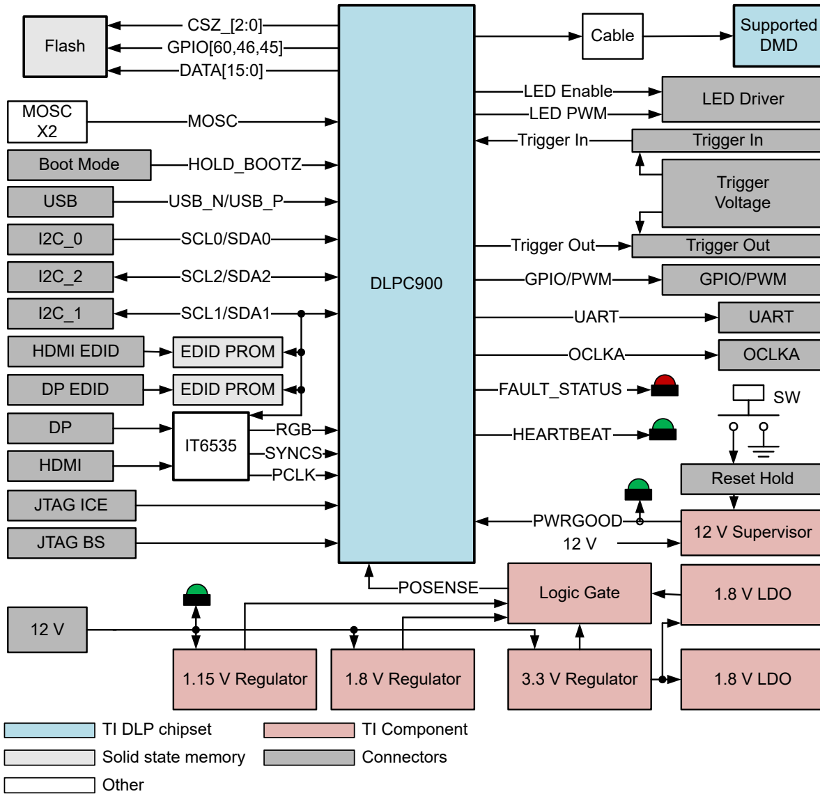
图 1-2. DLP LightCrafter 单 DLPC900 EVM 方框图
