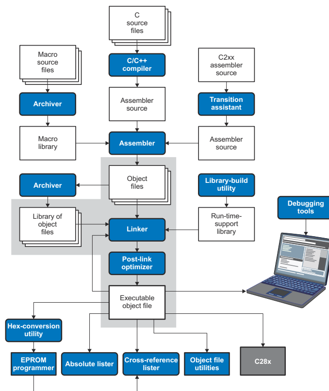
图 8-1. TMS320C28x 软件开发流程中的链接器
