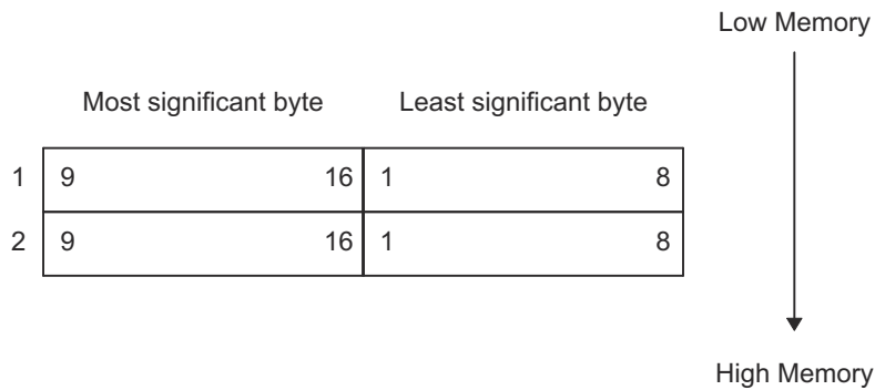
图 8-11. CRC 数据流示例
