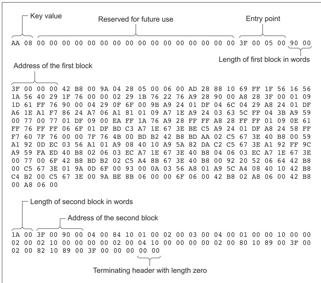
图 12-8. 从 8 位 SCI Boot 引导的示例性十六进制转换器输出文件
