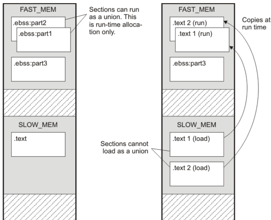
图 8-5. 存储器分配如 UNION 语句和 UNION 段的单独加载地址 所示
