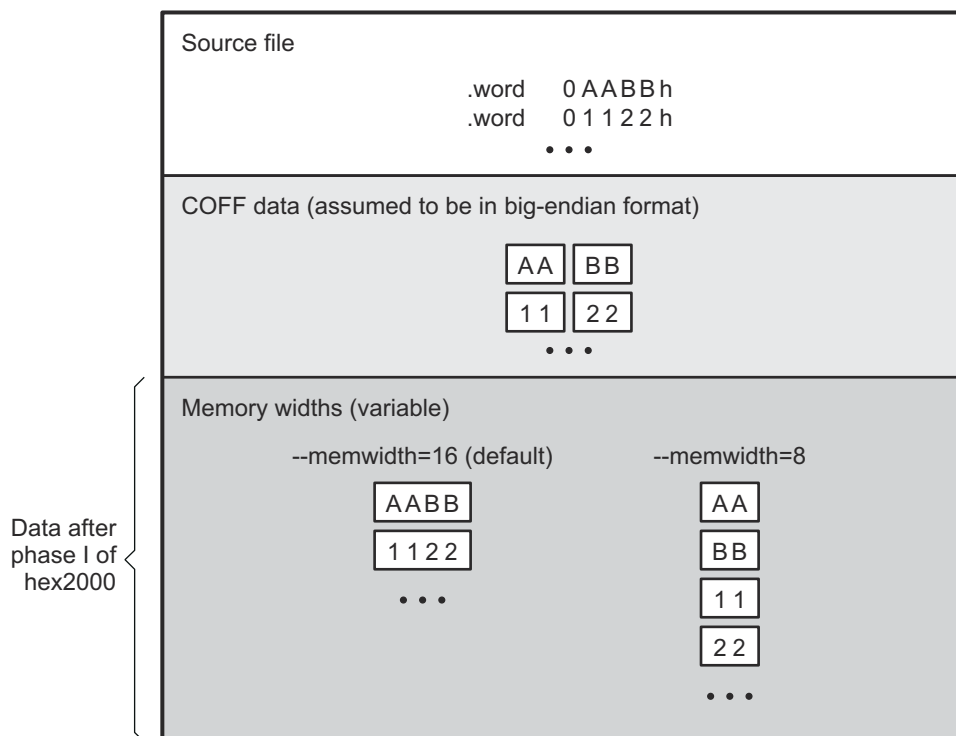
图 12-3. 目标文件数据与存储器宽度
