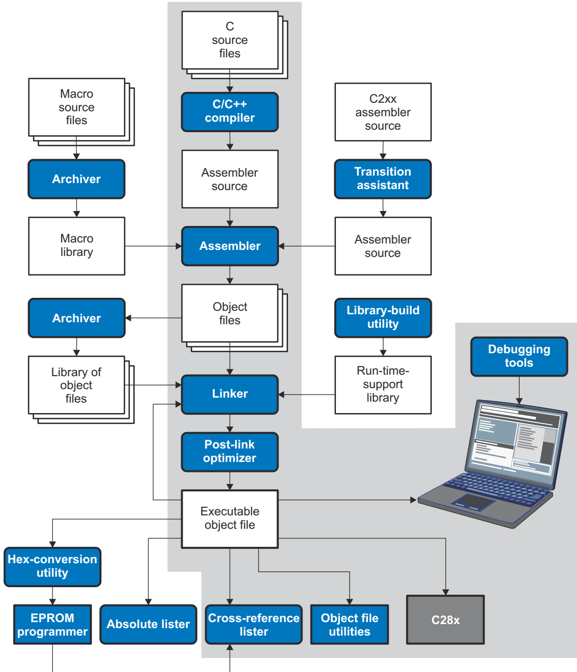
图 4-1. TMS320C28x 软件开发流程中的汇编器
