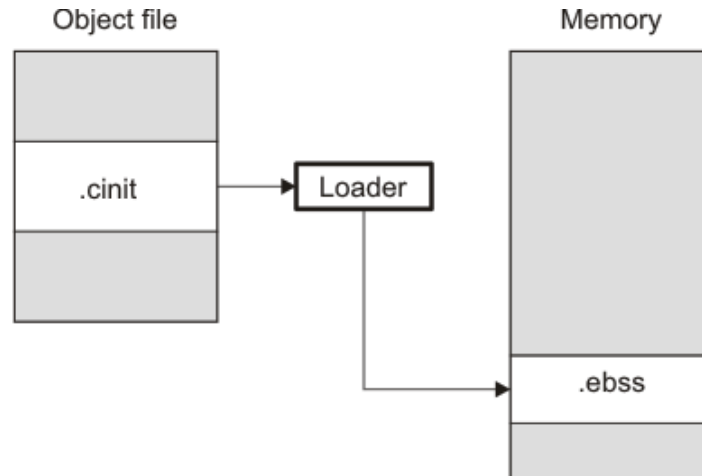
图 3-4. 加载时初始化
