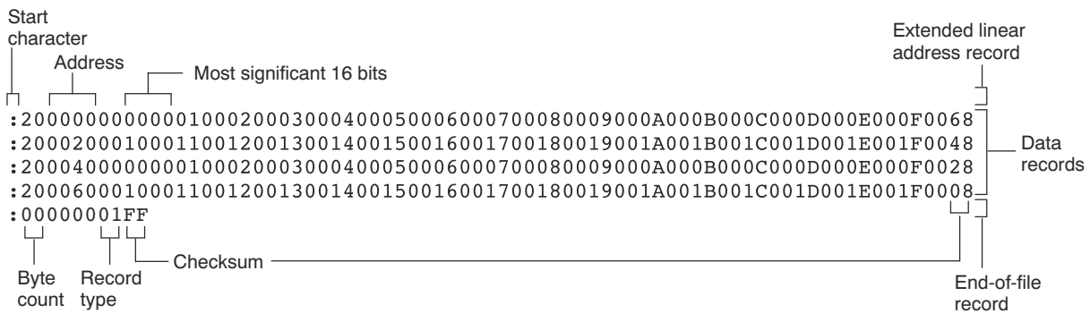
图 12-10. Intel 十六进制目标格式
