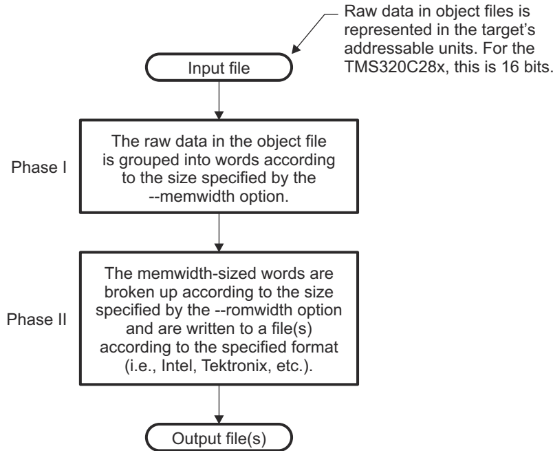
图 12-2. 十六进制转换实用程序处理流程
