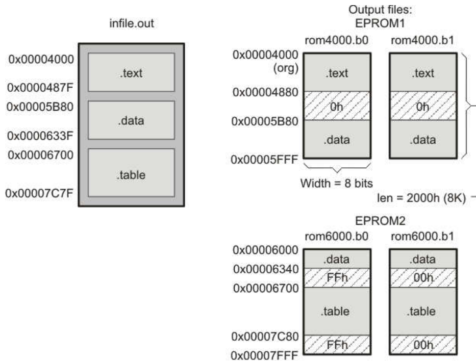
图 12-5. infile.out 文件分区为四个输出文件
