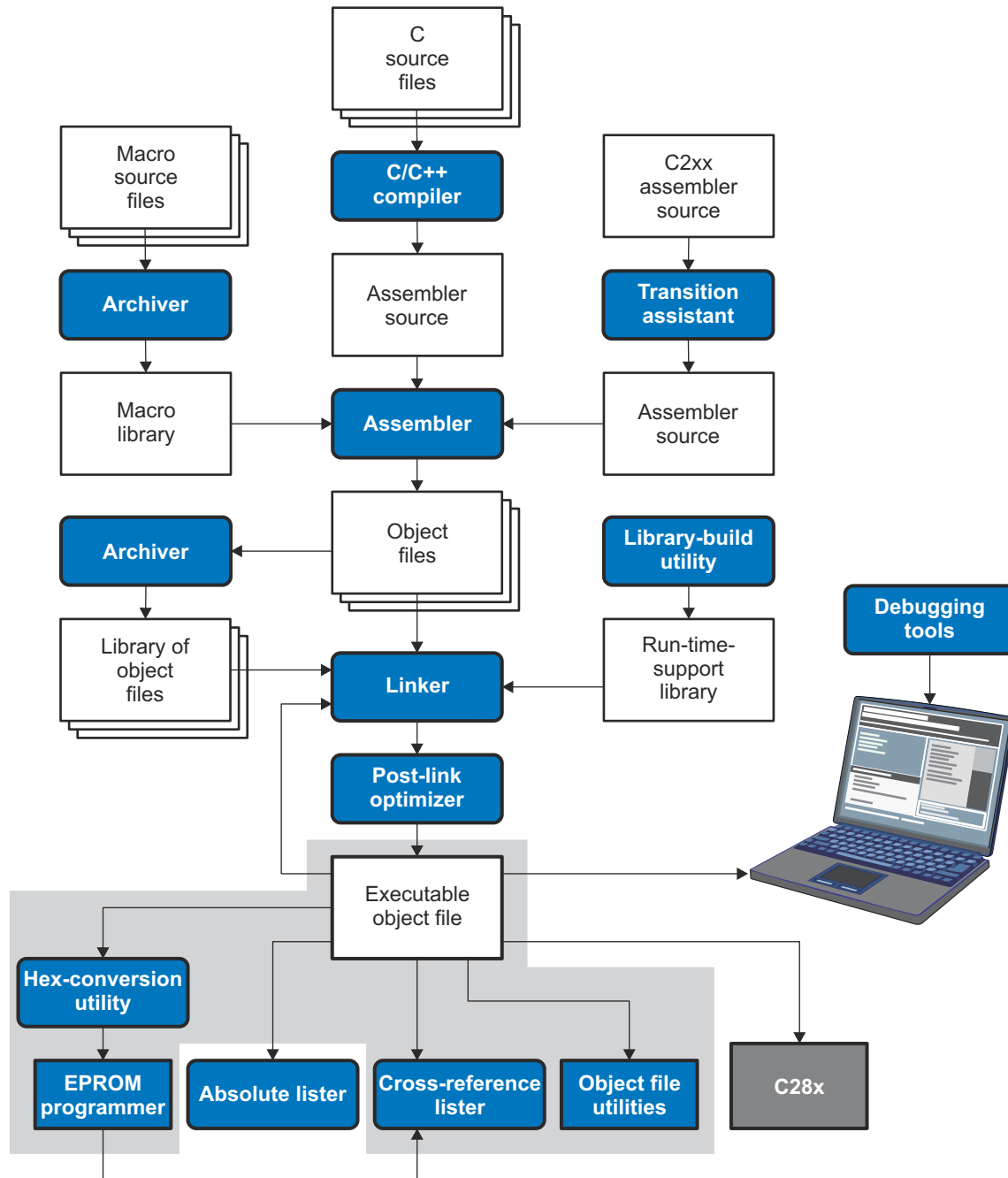
图 12-1. TMS320C28x 软件开发流程中的十六进制转换实用程序
