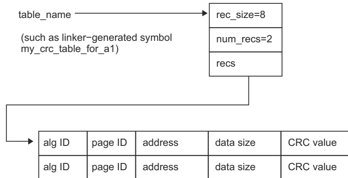
图 8-9. CRC_TABLE 概念模型
