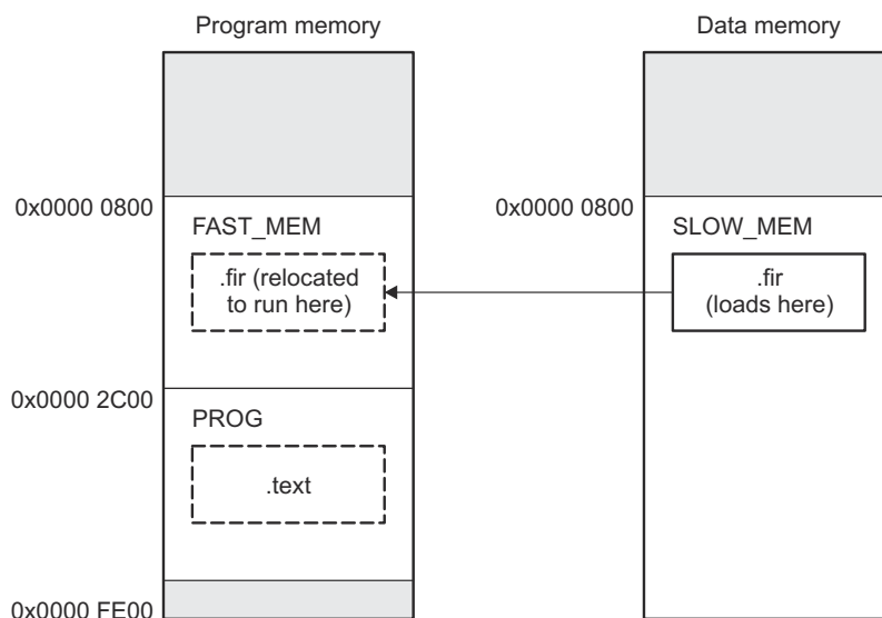
图 8-4. 在运行时将一个函数从慢速存储器移动到快速存储器 的运行时执行
