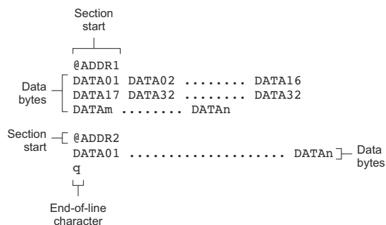
图 12-14. TI-TXT 目标格式
