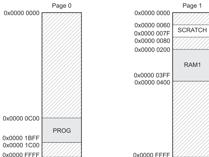
图 8-2. MEMORY 指令中定义的存储器映射
