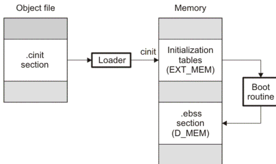
图 3-3. 运行时自动初始化
