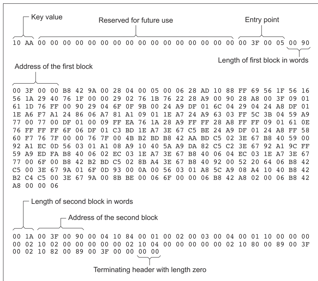
图 12-7. C28x 16 位并行引导 GP I/O 的示例十六进制转换器输出文件
