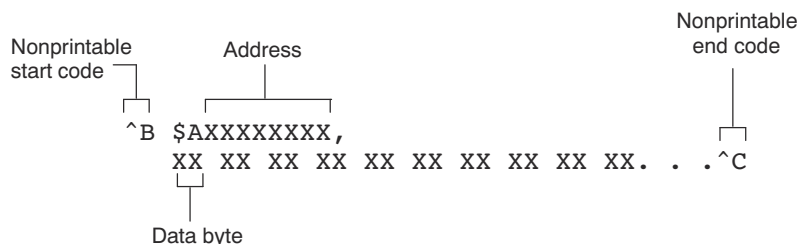
图 12-9. ASCII 十六进制对象格式
