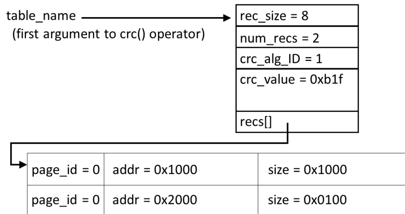
图 8-10. 存储器范围的 CRC 存储格式
