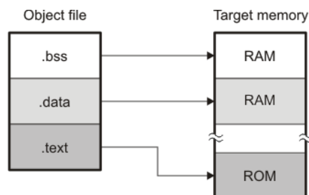
图 2-1. 存储器信息逻辑块分区
