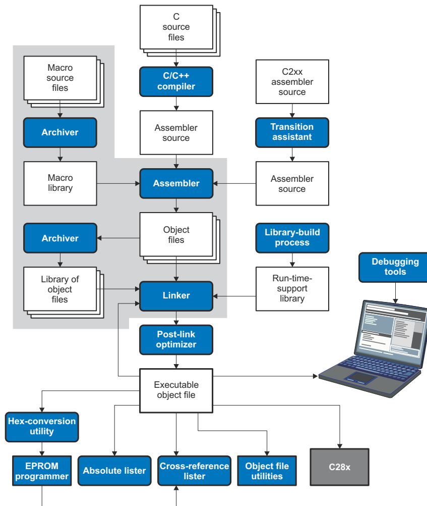
图 7-1. TMS320C28x 软件开发流程中的归档器
