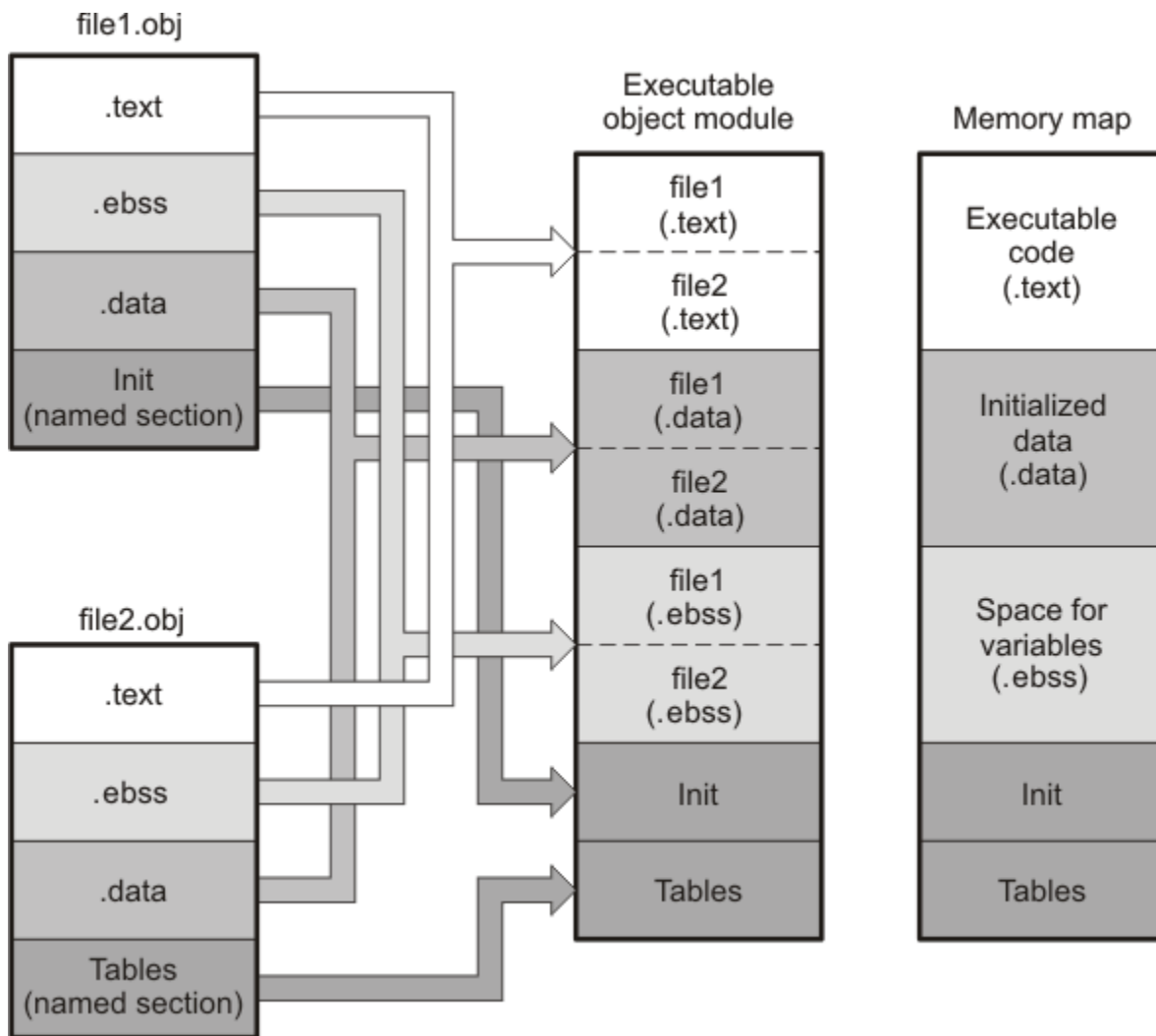
图 2-4. 组合输入段以构成可执行对象模块
