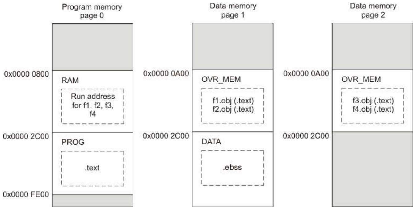
图 8-6. 示例 8-5 和 示例 8-6 中定义的重叠页
