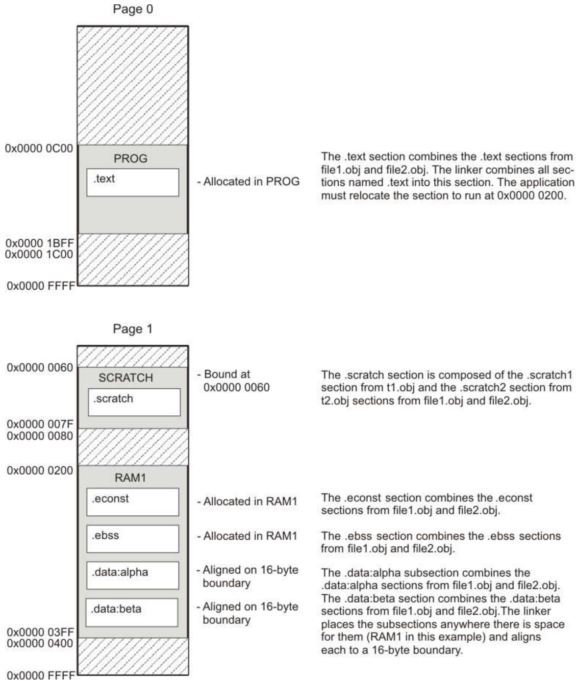
图 8-3. 由 SECTIONS 指令定义的段放置示例
