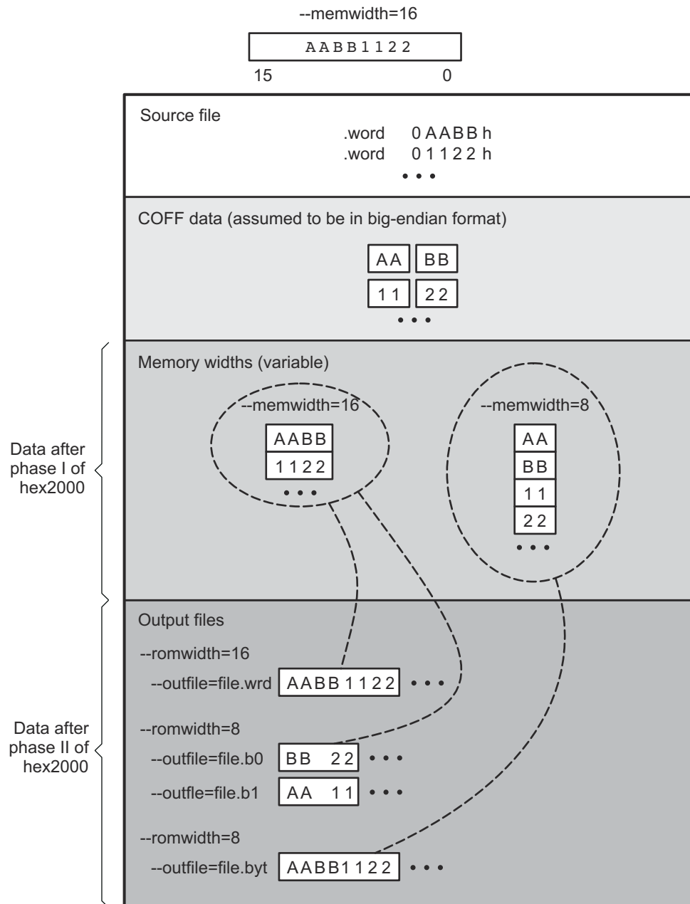
图 12-4. 数据、存储器和 ROM 宽度
