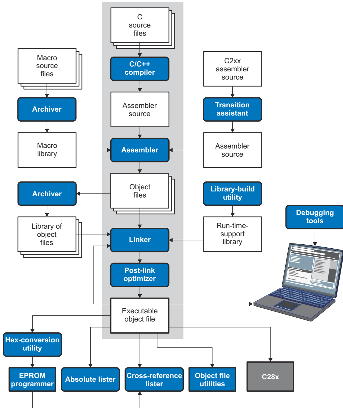
图 1-1. TMS320C28x 软件开发流程
