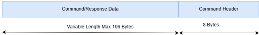
图 5-11. SPI 命令格式
