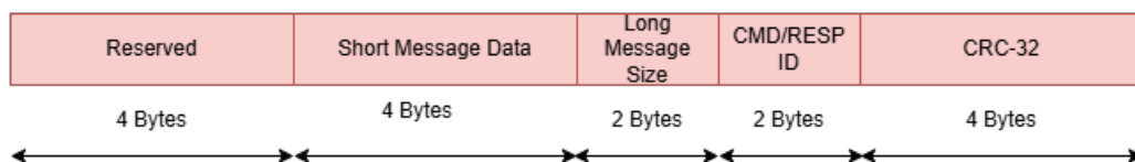
图 5-10. SPI 帧头格式
