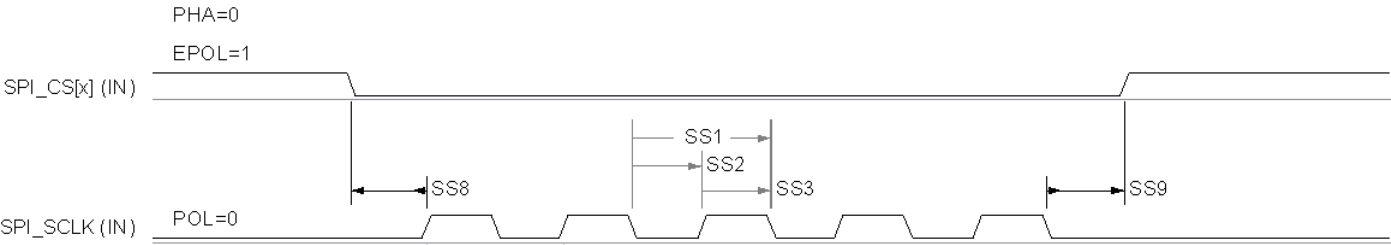
图 5-7. SPI 时序 — 外设模式接收
