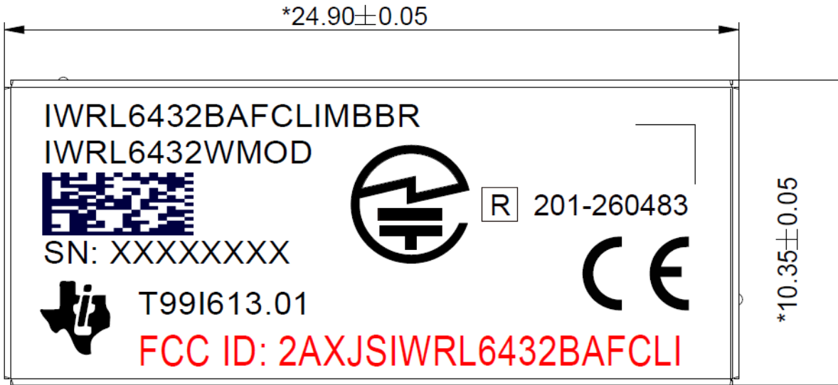
图 9-3. 器件产品标识示例
