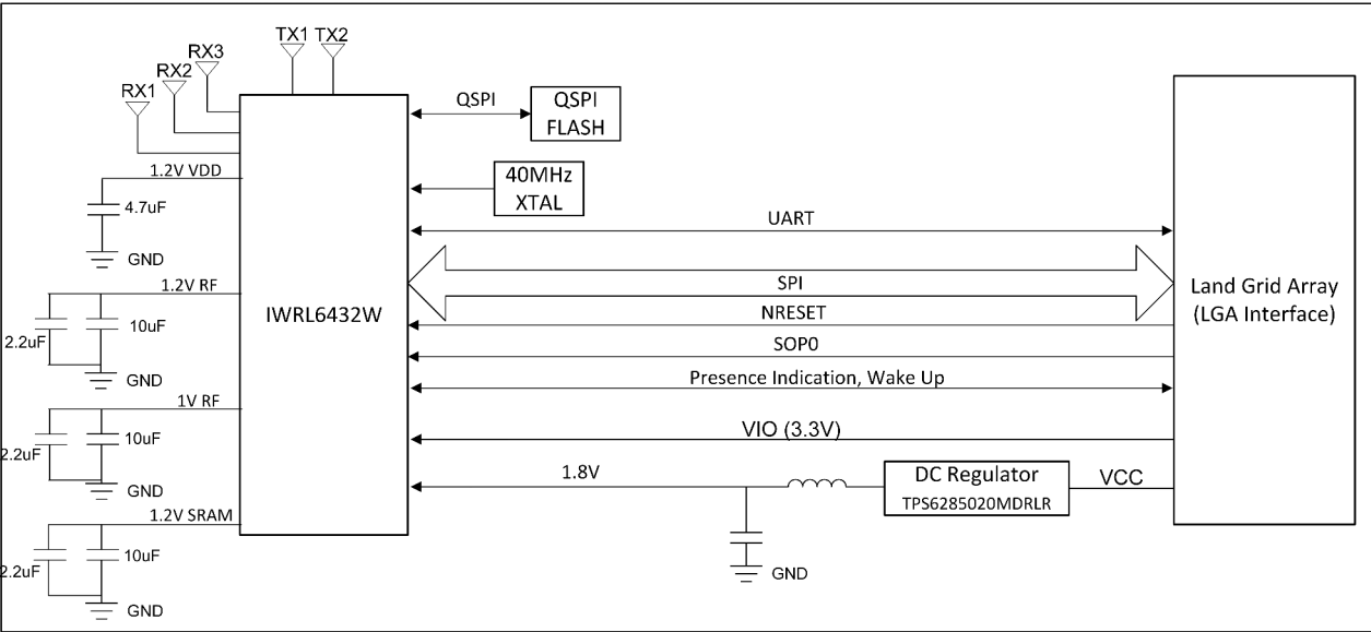
IWRL6432WMOD
