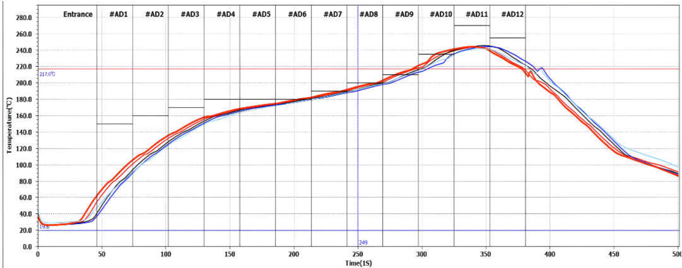
图 10-1. 模块回流焊曲线
