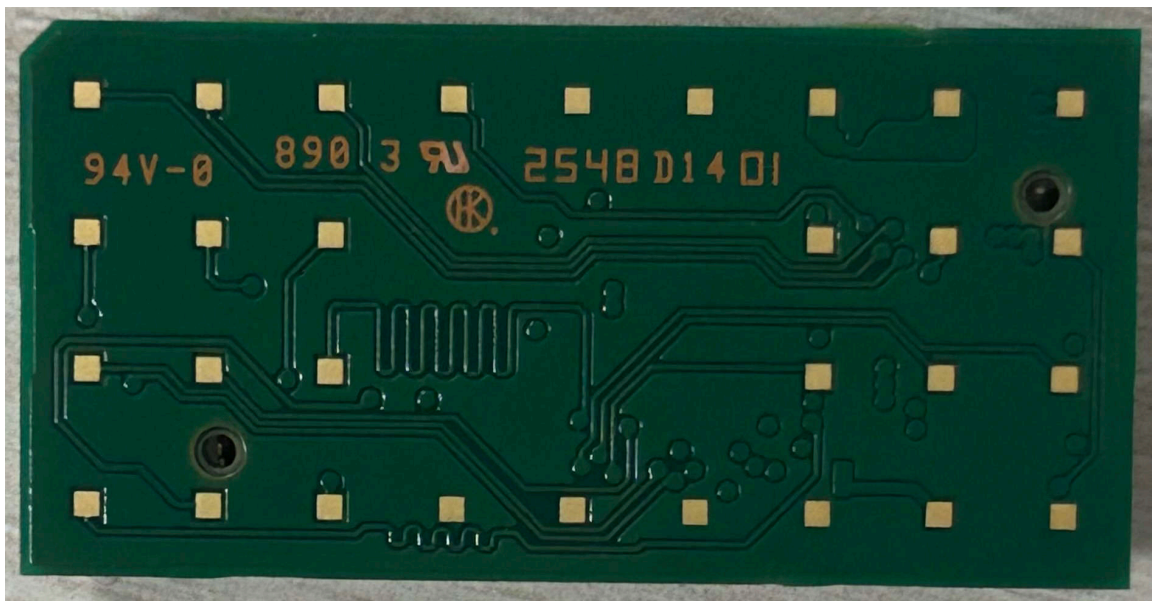
图 6-2. 模块底部
