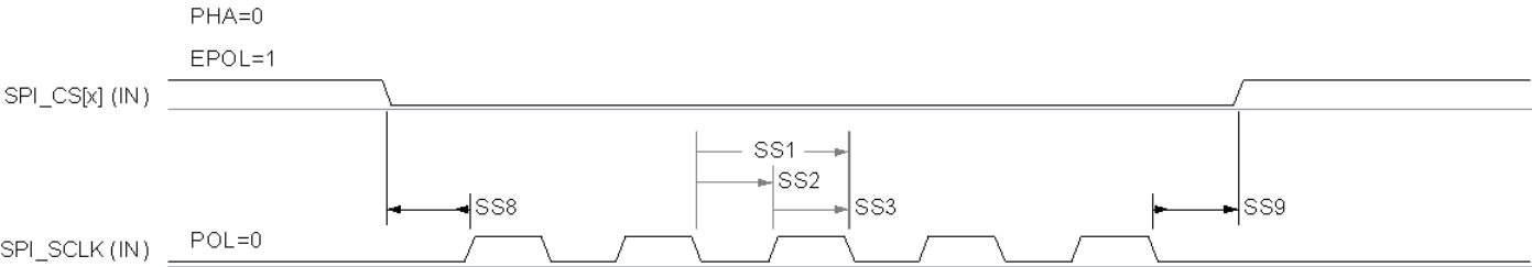
图 5-7. SPI 时序 — 外设模式接收
