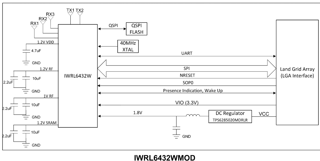
图 6-3. 功能方框图
