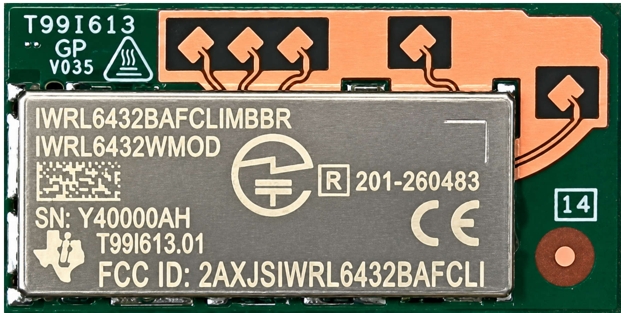
图 6-1. 模块顶部
