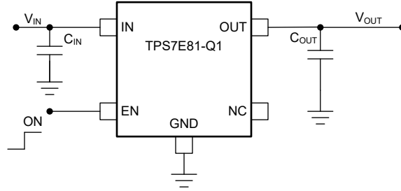
图 7-5. 典型应用电路 (固定电压版本)
