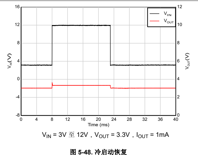
图 5-48. 冷启动恢复
