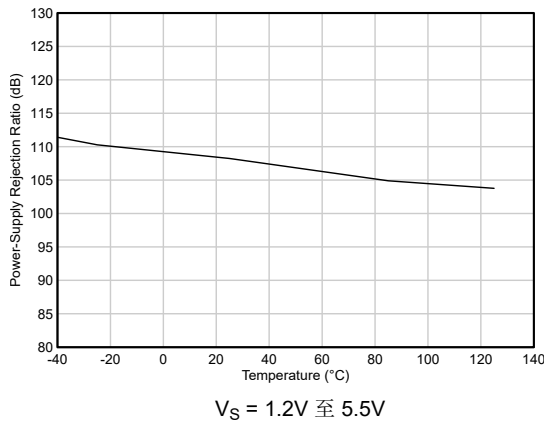
图 5-17. 直流 PSRR 与温度间的关系
