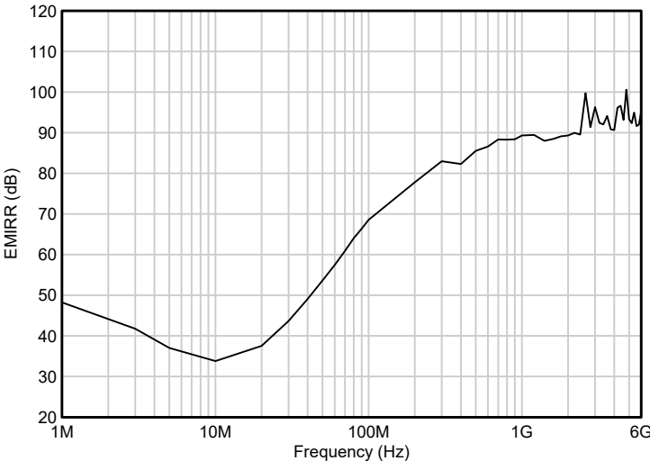
图 6-5. EMIRR 测试
