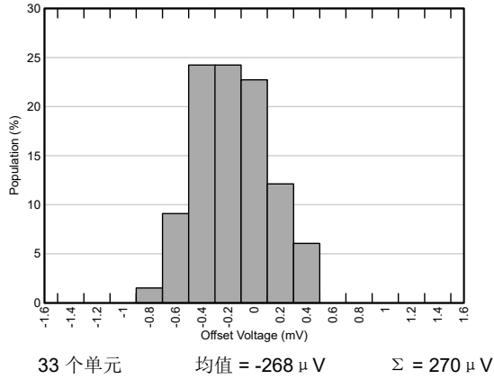
图 5-1. 失调电压分布直方图
