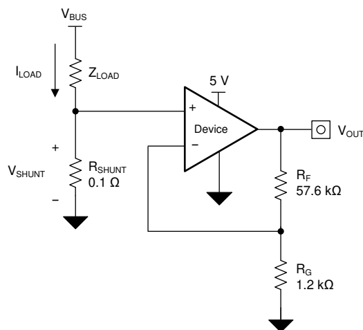
图 7-1. 低侧电流检测应用中的 TLV904xD
