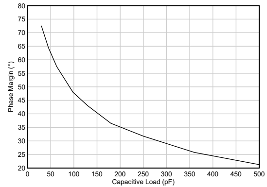
图 5-26. 相位裕度与容性负载间的关系
