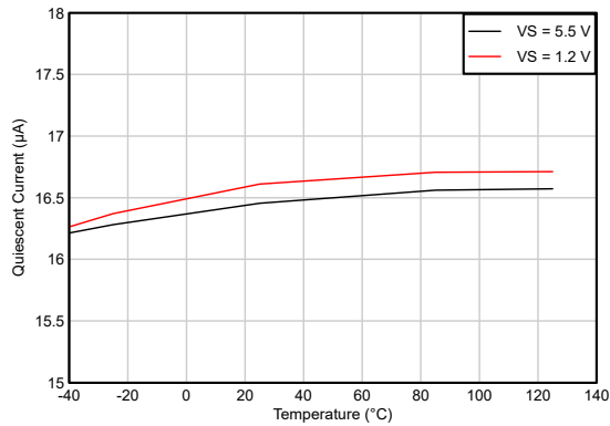
图 5-25. 静态电流与温度间的关系
