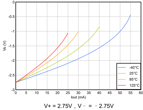
图 5-13. 输出电压与输出电流间的关系 (爪形)
