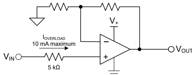
图 6-7. 输入电流保护
