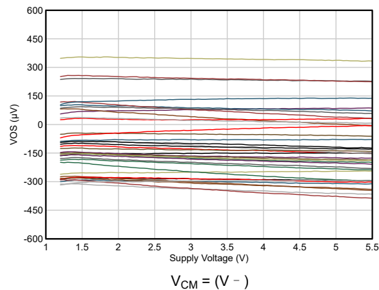
图 5-5. 偏移电压与电源电压间的关系
