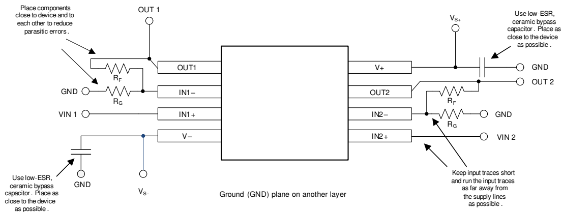
图 7-12. 布局示例
