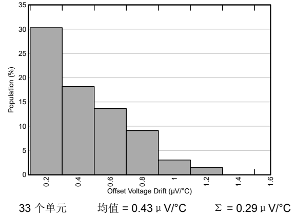
图 5-2. 失调电压漂移分布直方图
