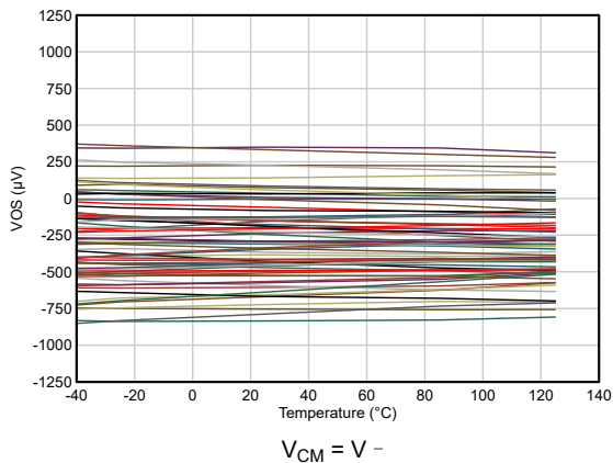
图 5-3. 输入失调电压与温度间的关系
