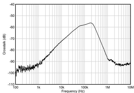
图 5-35. 通道隔离
