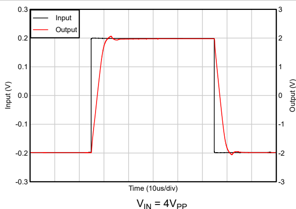
图 5-32. 大信号阶跃响应 (TLV9042D)
