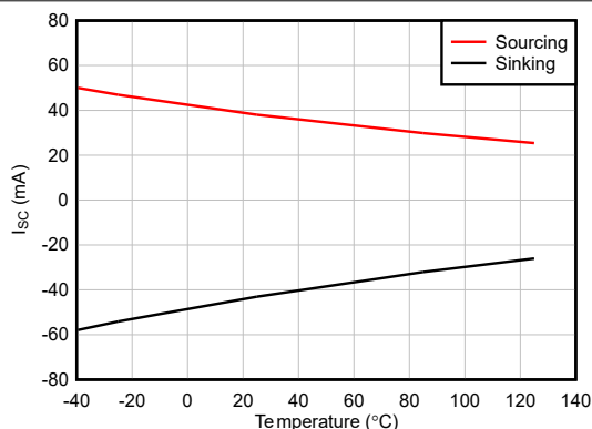
图 5-33. 短路电流与温度间的关系
