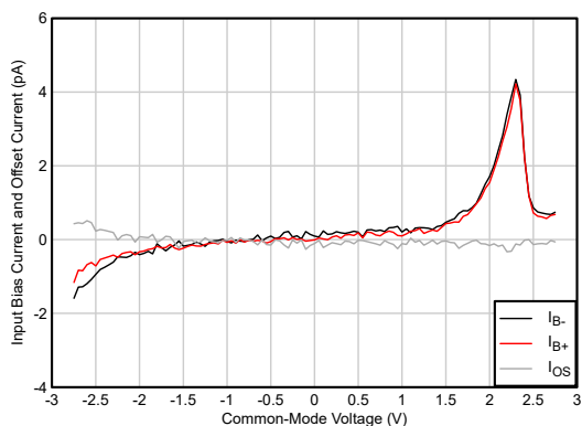
图 5-7. I_B 和 I_{OS} 与共模电压间的关系
