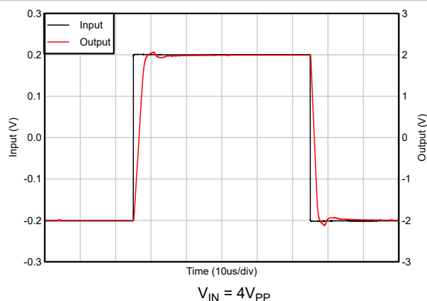
图 5-31. 大信号阶跃响应 (TLV9041D)
