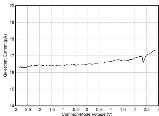
图 5-23. 静态电流与共模间的关系
