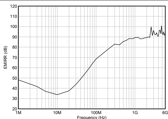
图 5-34. 以同相输入为基准的电磁干扰抑制比 (EMIRR+) 与频率间的关系
