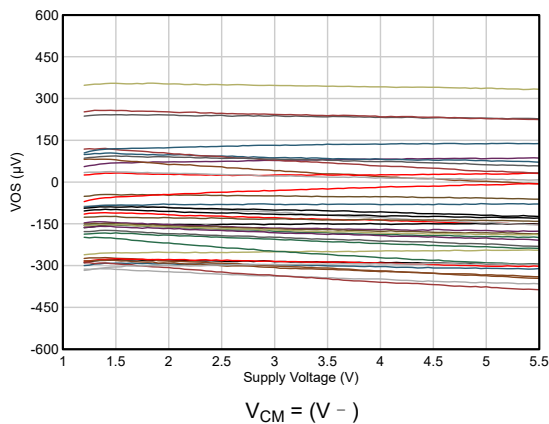
图 5-5. 偏移电压与电源电压间的关系
