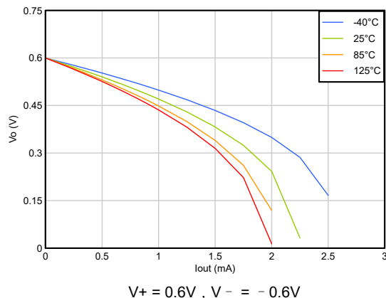
图 5-14. 输出电压与输出电流间的关系 (爪形)
