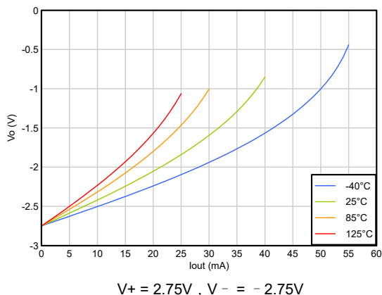
图 5-13. 输出电压与输出电流间的关系 (爪形)
