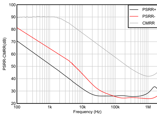
图 5-16. CMRR 和 PSRR 与频率间的关系
