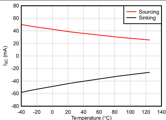
图 5-33. 短路电流与温度间的关系
