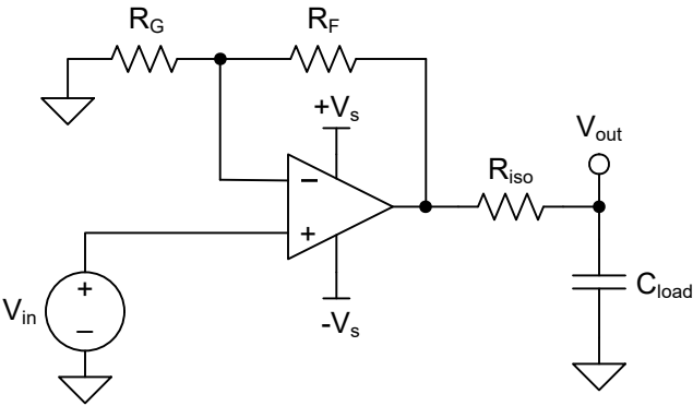
图 6-4. 增强容性负载驱动能力
