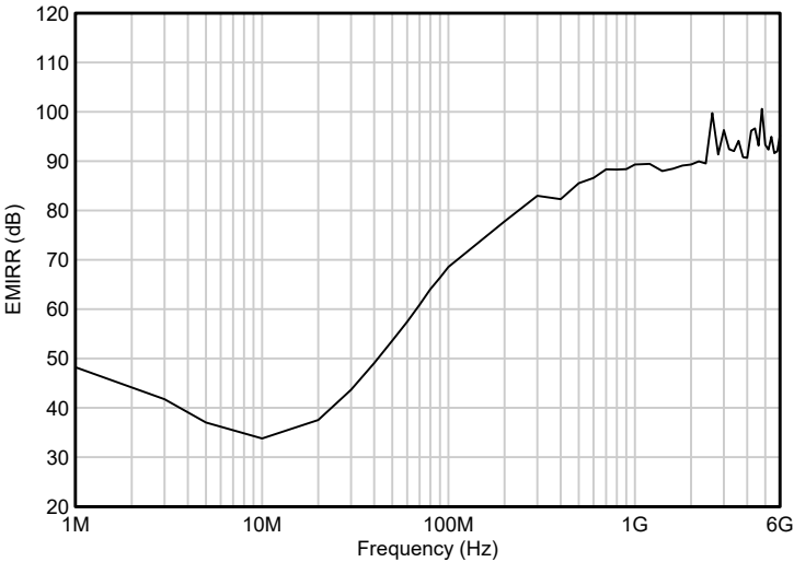
图 6-5. EMIRR 测试
