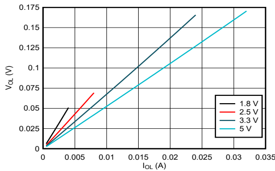
图 5-3. 低电平状态下输出电压与电流间的关系
