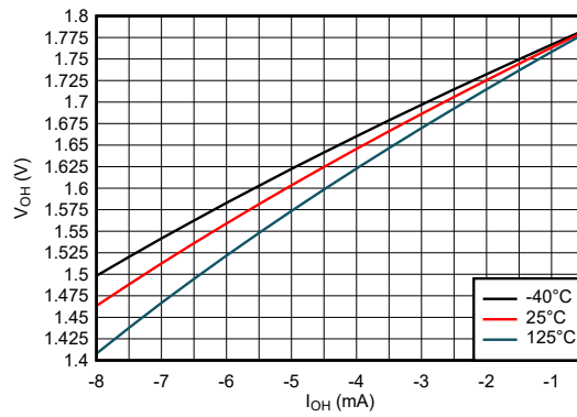
图 5-7. 高电平状态下输出电压与电流间的关系 (1.8V 电源)
