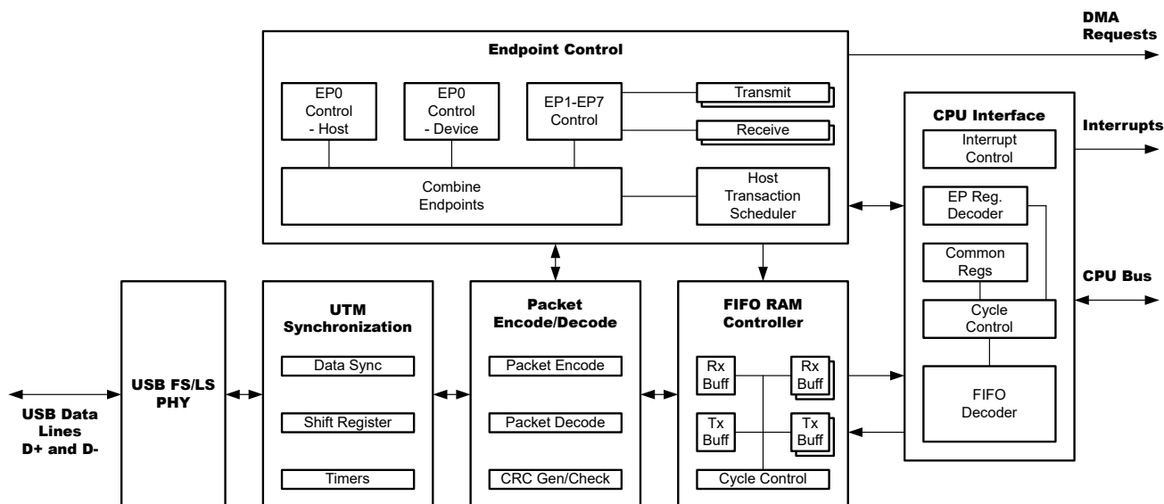
图 8-4. USB 方框图
