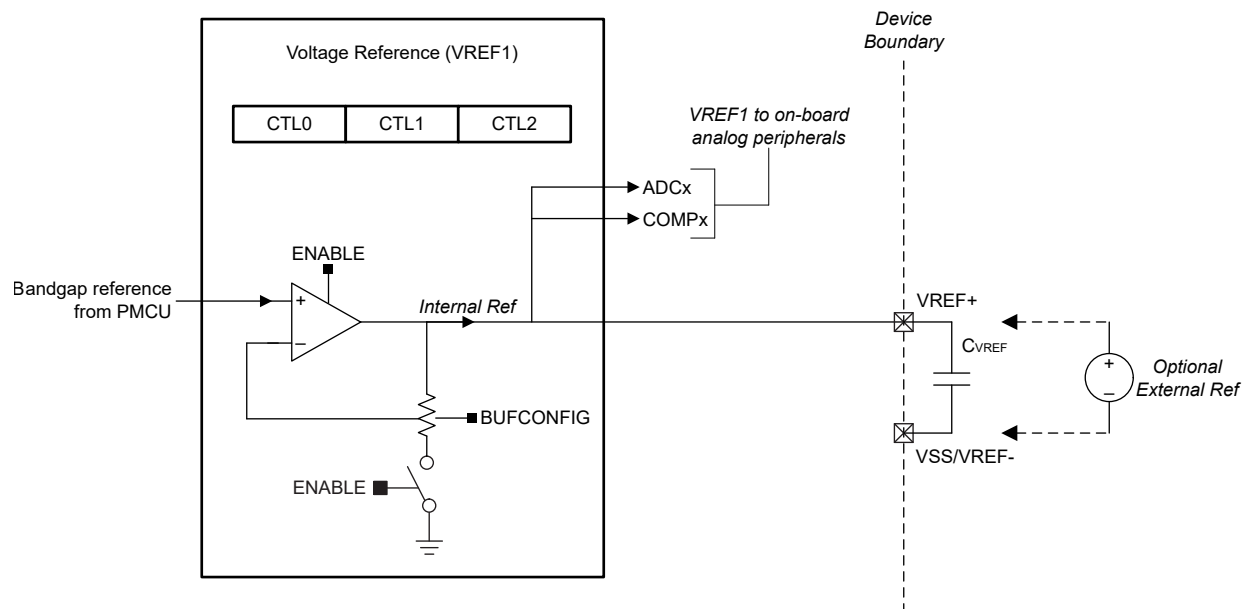
图 8-2. VREF1 模块
