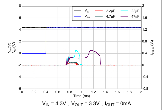
图 5-28. 浪涌电流与 C_{OUT} 间的关系
