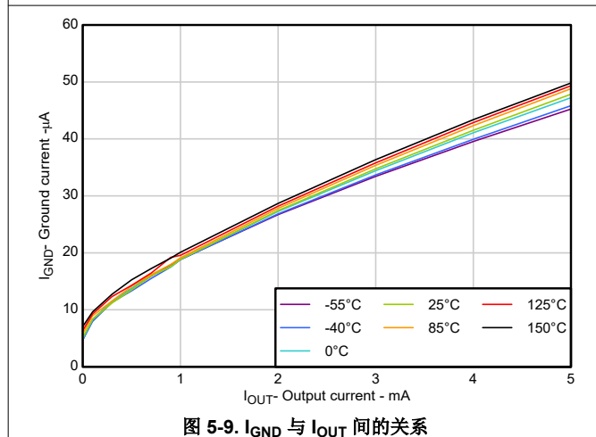
图 5-9. I_{GND} 与 I_{OUT} 间的关系
