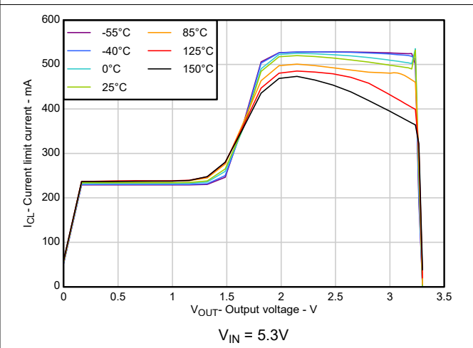
图 5-12. 折返电流限值 I_{CL} 与温度间的关系
