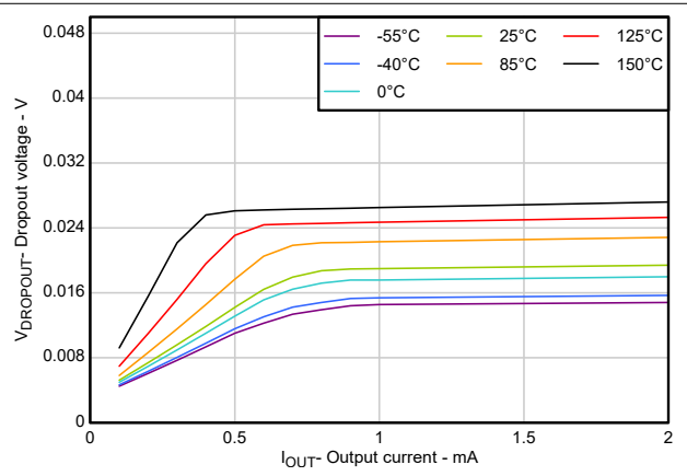
图 5-6. V_{DO} 与 I_{OUT} (mA) 间的关系
