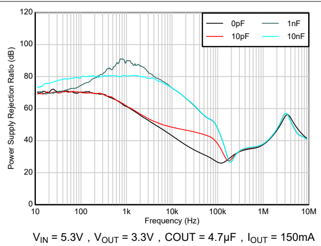
图 5-22. PSRR 与 C_{FF} 间的关系
