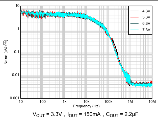
图 5-24. 噪声与 V_{IN} 间的关系
