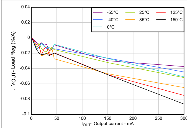
图 5-5. 负载调整率
