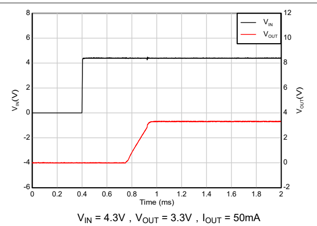
图 5-30. EN 与 V_{IN} 引脚短接启动
