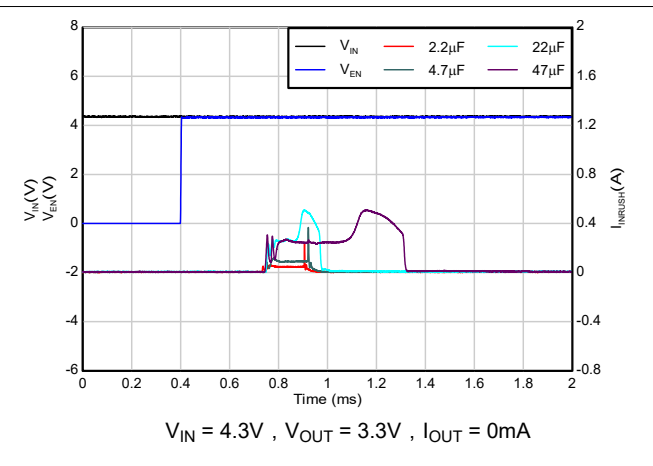
图 5-28. 浪涌电流与 C_{OUT} 间的关系
