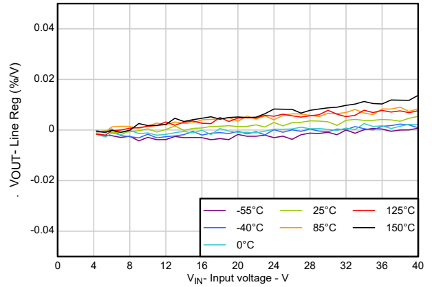
图 5-4. 线路调整率
