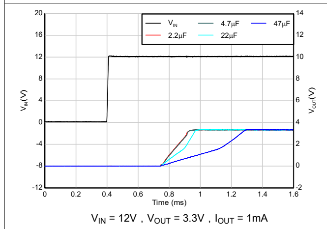
图 5-27. 启动与 C_{OUT} 间的关系
