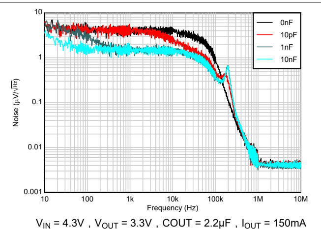
图 5-26. 噪声与 C_{FF} 间的关系
