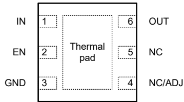
图 4-1. DRV 封装 (固定/ADJ) , 6-引脚 WSON (顶视图)
