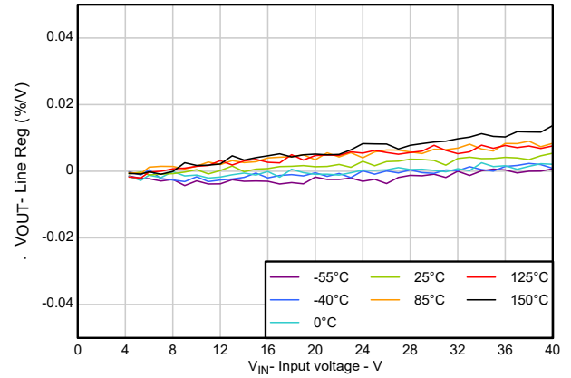
图 5-4. 线路调整率
