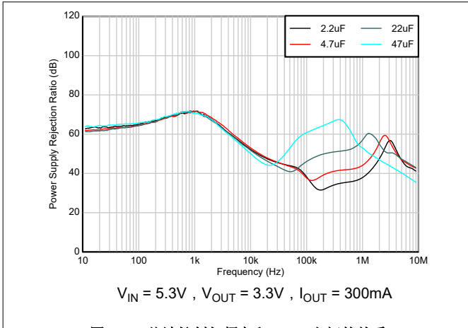
图 5-19. 纹波抑制与频率和 C_{OUT} 之间的关系
