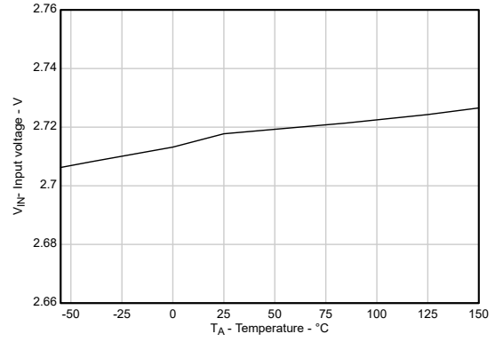
图 5-2. 下降输入电源 UVLO 与温度之间的关系
