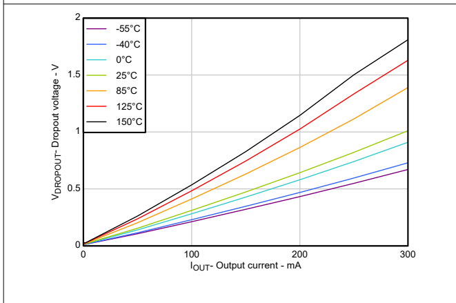
图 5-9. 压降电压与输出电流之间的关系
