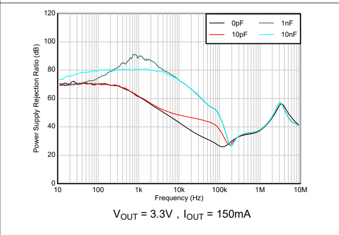
图 5-22. 纹波抑制与频率和 C_{FF} 之间的关系
