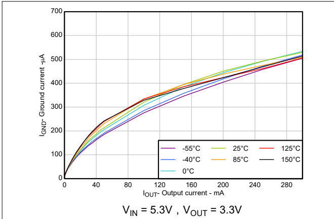
图 5-13. 接地电流与输出电流间的关系
