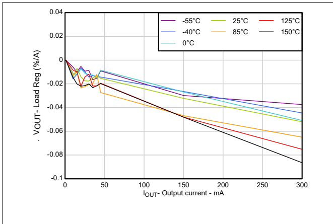
图 5-7. 负载调整率与输出电流之间的关系
