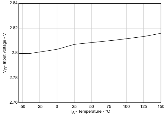
图 5-1. 上升输入电源 UVLO 与温度之间的关系
