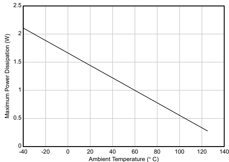
图 7-3. TPS7E81 (DRV) 允许的功率耗散
