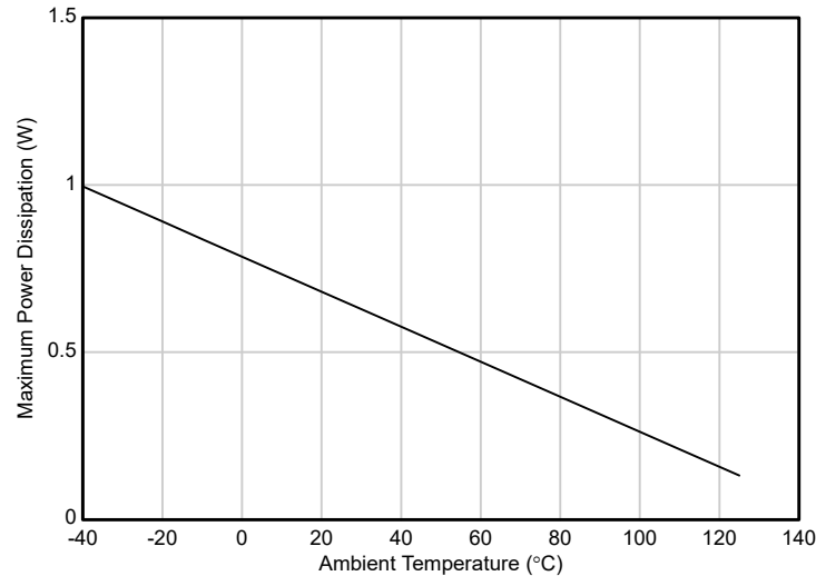
图 7-2. TPS7E81 (DBV) 允许的功率耗散
