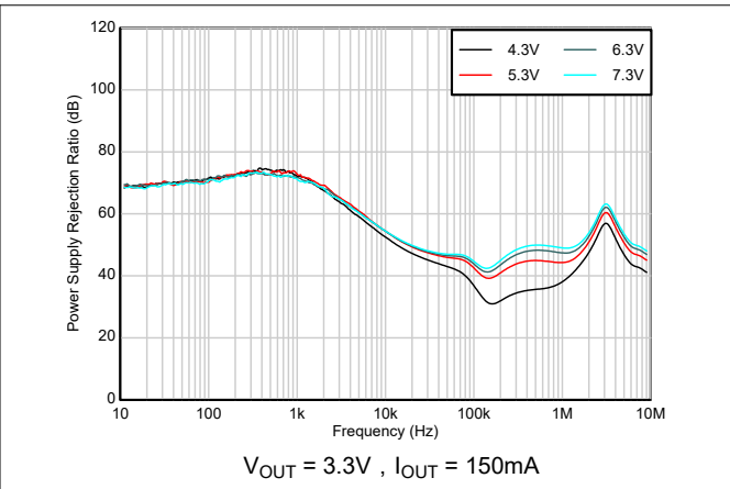
图 5-20. 纹波抑制与频率和输入电压之间的关系
