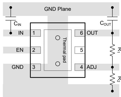
图 7-12. TPS7E81 ( DRV 封装 ) 的布局示例
