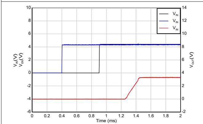
图 5-47. 时序启动 (IN 在 EN 之后)
