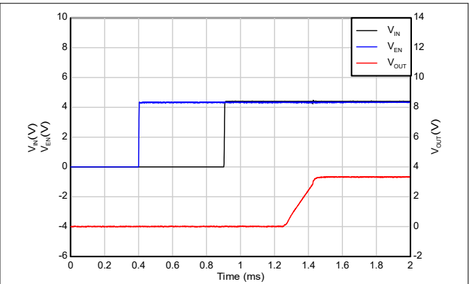
图 5-48. 时序启动 (IN 在 EN 之后)
