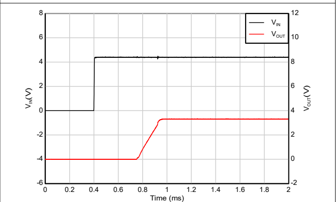
图 5-50. IN 与 EN 引脚短接启动
