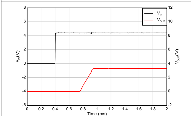
图 5-49. 时序启动 (IN 在 EN 之后)
