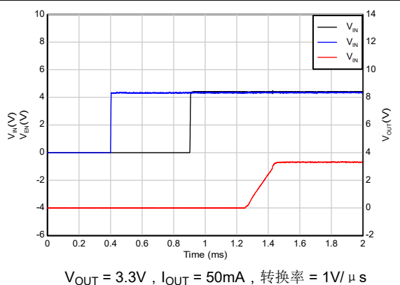
图 7-9. 时序启动 (IN 在 EN 之后)
