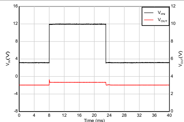
图 5-33. 冷启动恢复
