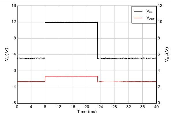
图 5-32. 线路瞬态
