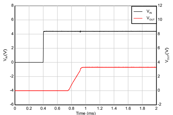
图 5-49. 时序启动 (IN 在 EN 之后)
