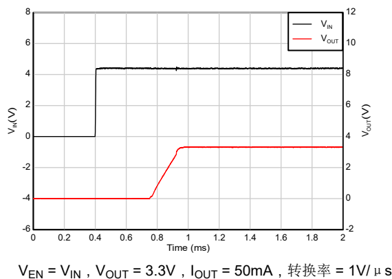
图 7-10. IN 与 EN 引脚短接启动
