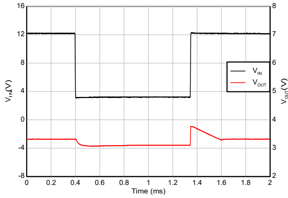
图 5-39. 压降恢复
