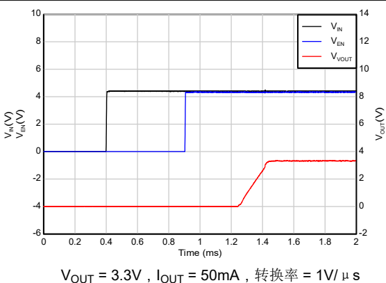
图 7-8. 时序启动 (EN 在 IN 之后)
