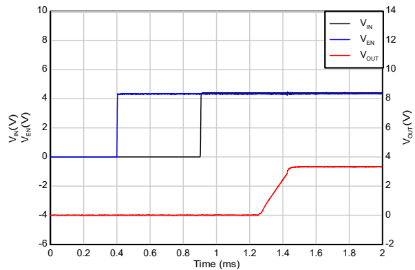
图 5-48. 时序启动 (IN 在 EN 之后)
