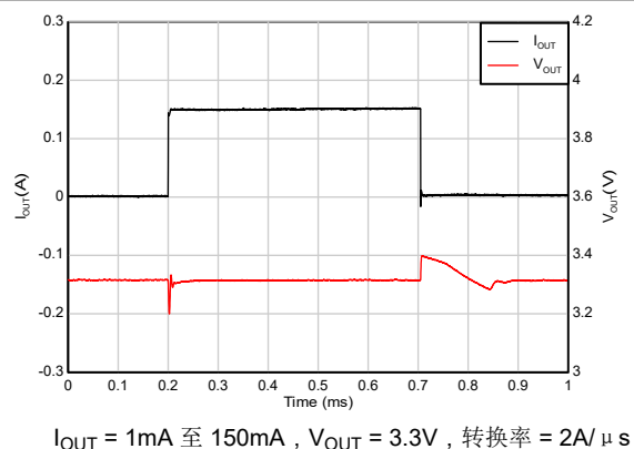
图 7-7. 负载瞬态
