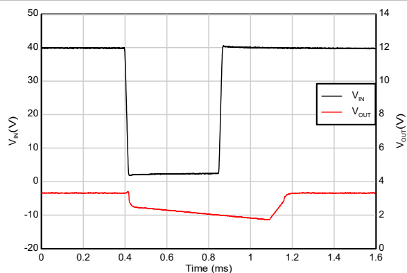
图 5-41. 欠压恢复
