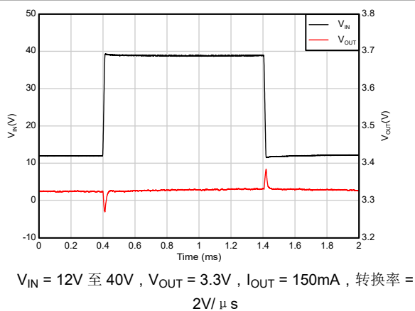
图 7-6. 线路瞬态
