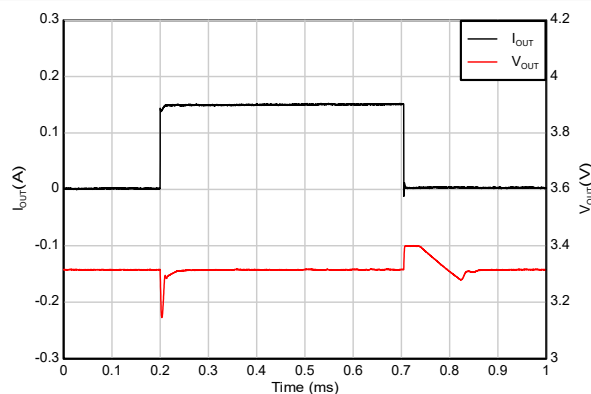
图 5-35. 负载瞬态
