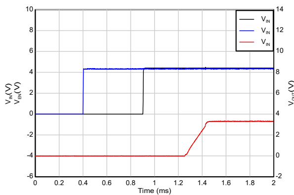
图 5-47. 时序启动 (IN 在 EN 之后)
