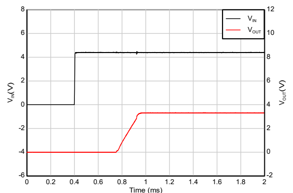
图 5-50. IN 与 EN 引脚短接启动
