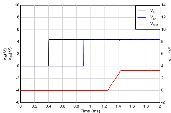
图 5-42. 欠压恢复
