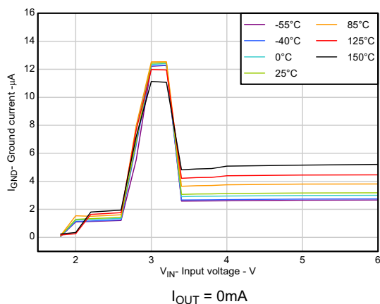
图 5-11. 接地电流与输入电压间的关系
