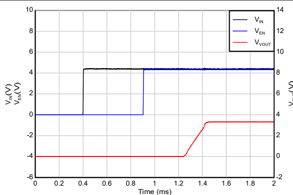
图 5-44. 时序启动 (EN 在 IN 之后)
