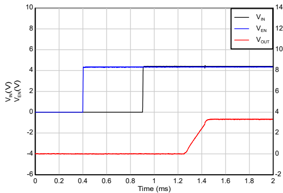
图 5-47. 时序启动 (IN 在 EN 之后)
