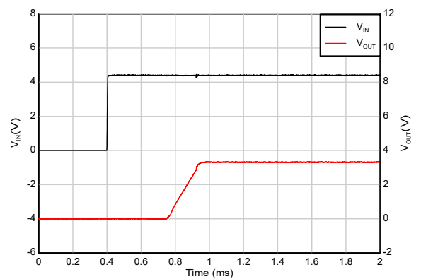
图 5-48. 时序启动 (IN 在 EN 之后)
