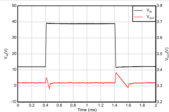
图 5-31. 线路瞬态
