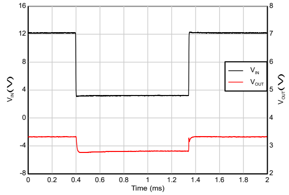
图 5-38. 压降恢复
