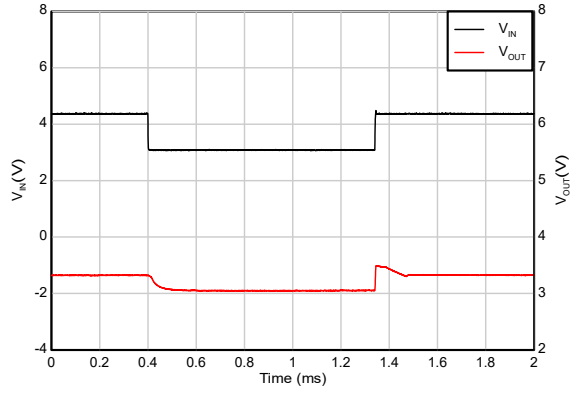
图 5-37. 压降恢复
