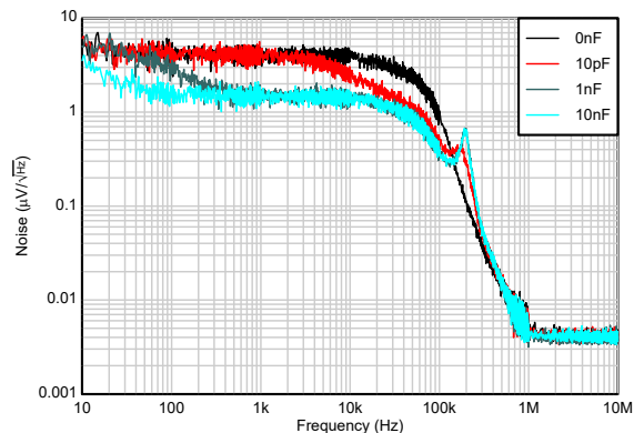
图 5-26. 输出噪声与频率和 C_{FF} 之间的关系
