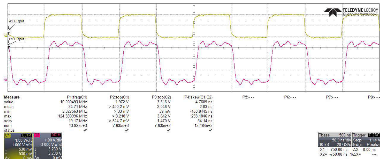
图 8-1. 10MHz 信号的电压转换 ( V_{CCA} = 1.8V , V_{CCB} = 3.6V , C_L = 20 英寸+ 50pF )
