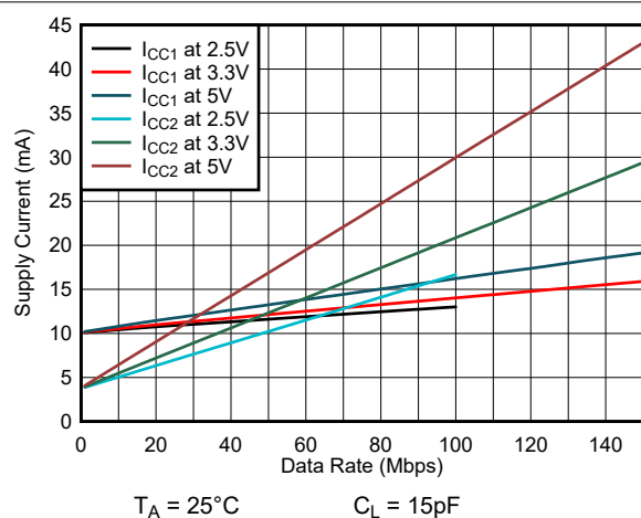
图 6-5. ISO6461 或 ISO6461F 电源电流与数据速率间的关系 (15pF 负载)
