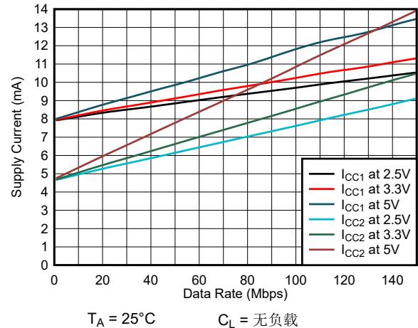
图 6-8. ISO6462 或 ISO6462F 电源电流与数据速率间的关系 (无负载)
