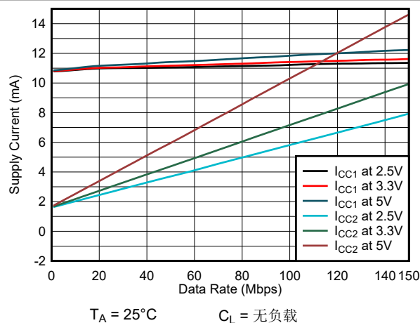
图 6-4. ISO6460 或 ISO6460F 电源电流与数据速率间的关系 (无负载)
