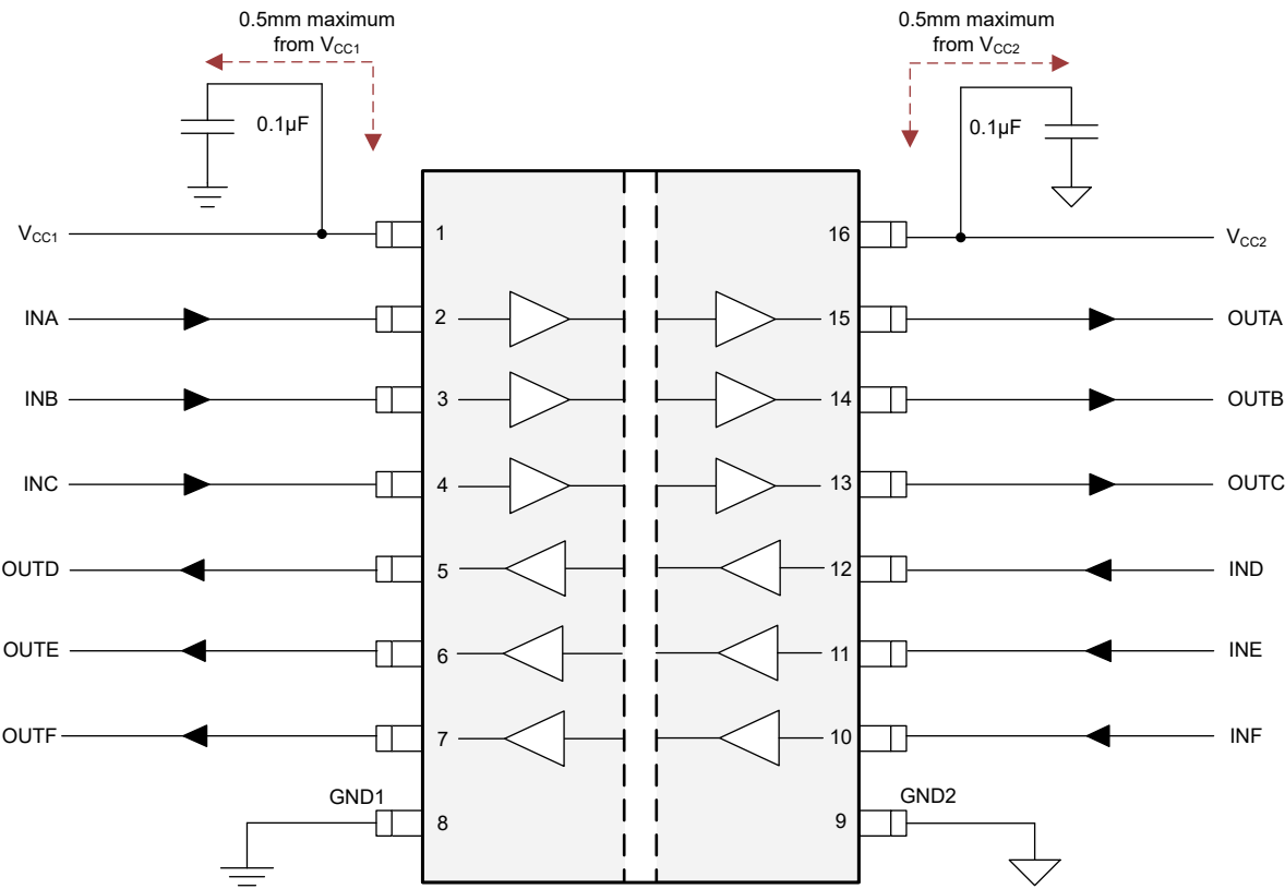
图 9-2. 典型 ISO646x 电路
