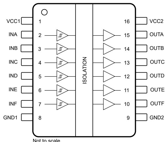
图 5-1. ISO6460 和 ISO6460F 顶视图
