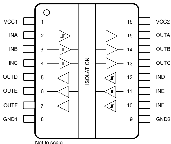
图 5-4. ISO6463 和 ISO6463F 顶视图
