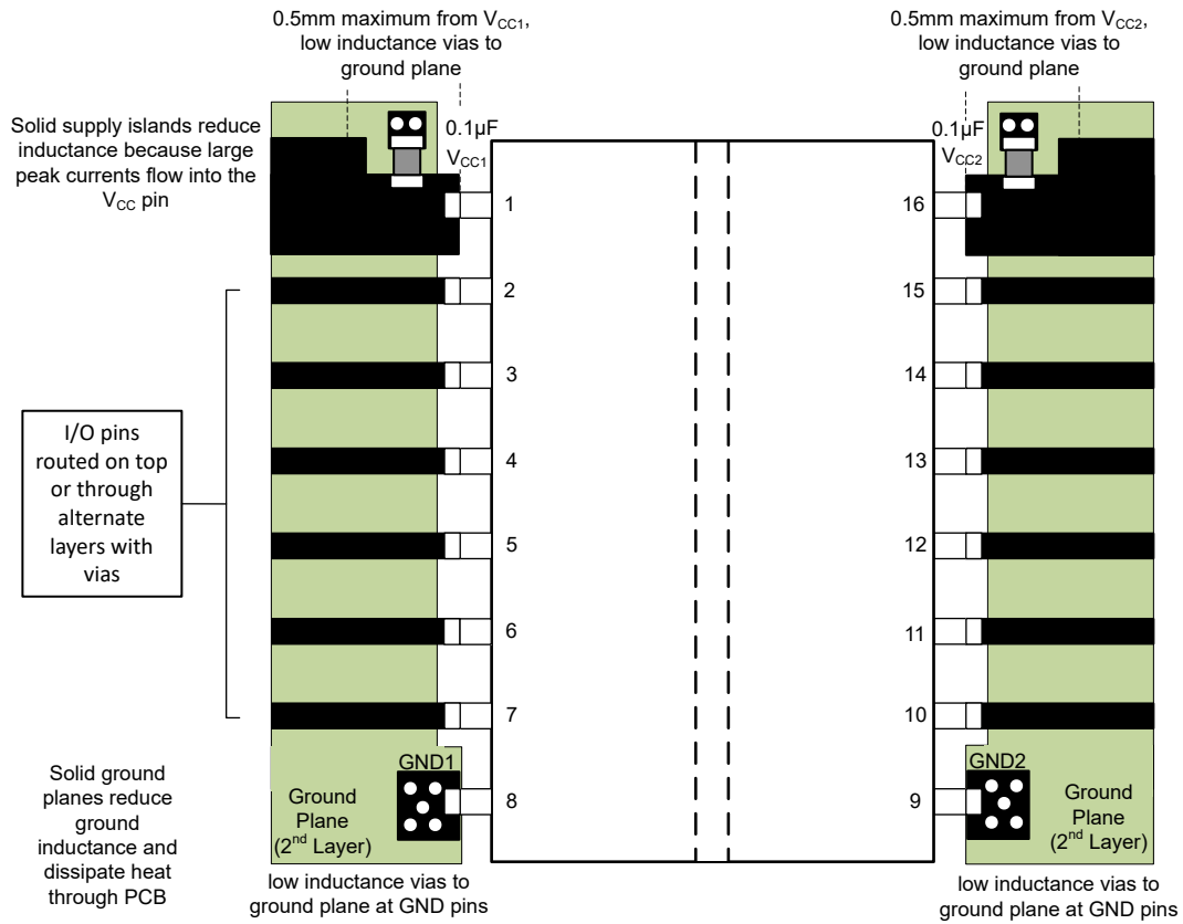
图 9-6. 布局示例
