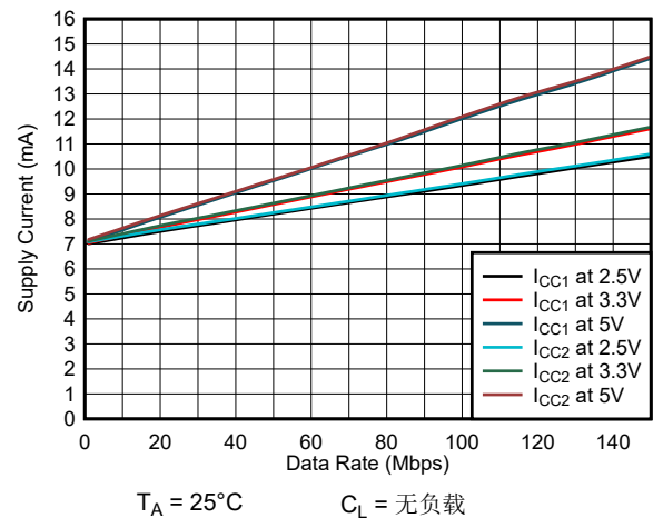
图 6-10. ISO6463 或 ISO6463F 电源电流与数据速率间的关系 (无负载)
