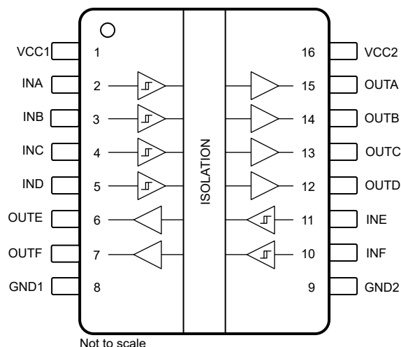
图 5-3. ISO6462 和 ISO6462F 顶视图
