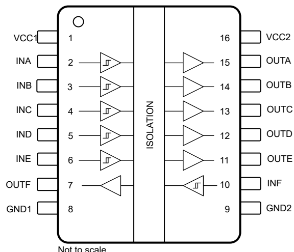
图 5-2. ISO6461 和 ISO6461F 顶视图
