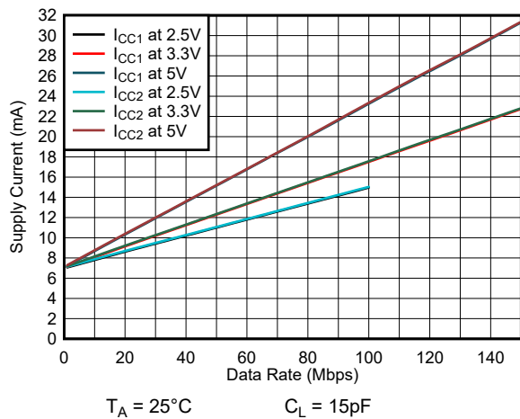
图 6-9. ISO6463 或 ISO6463F 电源电流与数据速率间的关系 (15pF 负载)
