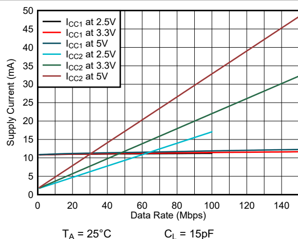
图 6-3. ISO6460 或 ISO6460F 电源电流与数据速率间的关系 (15pF 负载)
