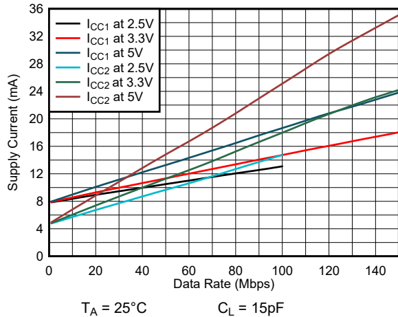
图 6-7. ISO6462 或 ISO6462F 电源电流与数据速率间的关系 (15pF 负载)
