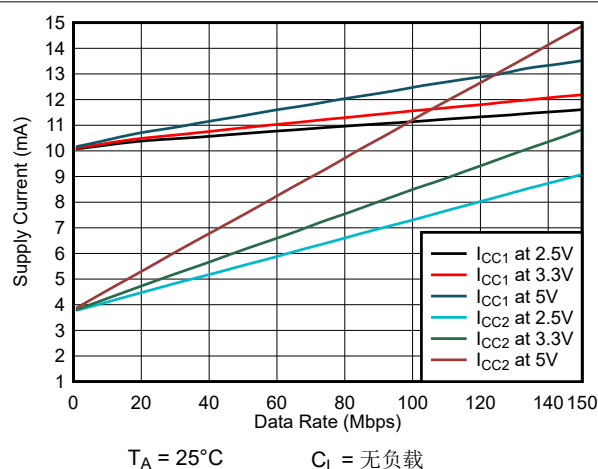
图 6-6. ISO6461 或 ISO6461F 电源电流与数据速率间的关系 (无负载)
