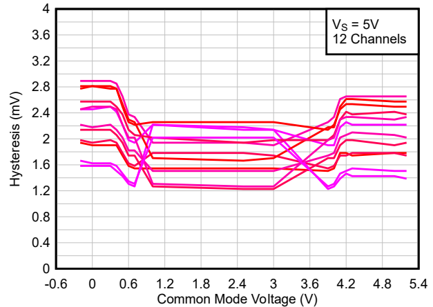
图 5-12. 迟滞与 共模电压间的关系, 5V
