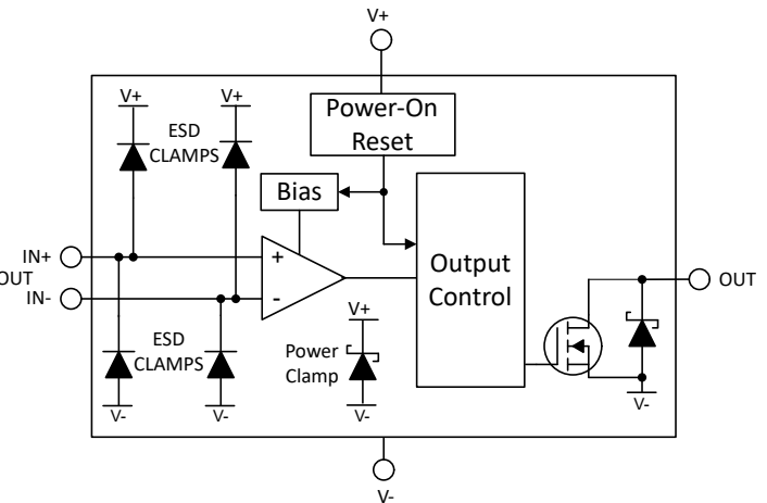
图 6-2. TLV322x 开漏方框图
