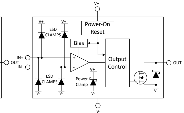
图 6-2. TLV322x 开漏方框图
