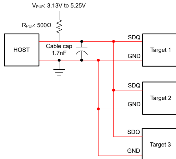
图 6-6. 多目标配置
