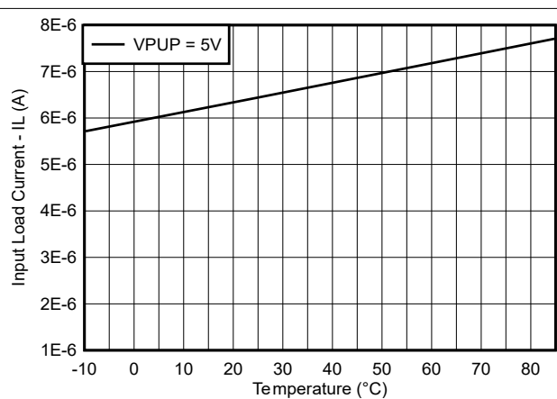
图 7-3. 输入负载电流 ( I_L ) 与温度间的关系 (超速)
