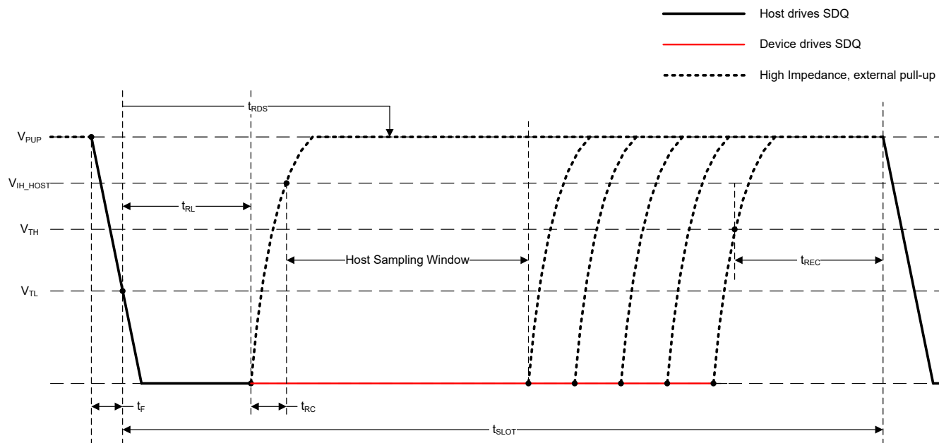
图 6-20. 读取数据时序图
