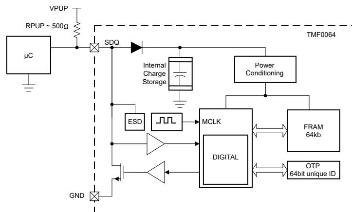
方框图
