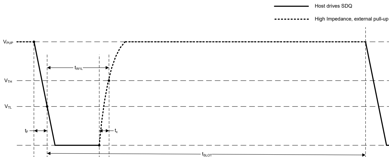
图 6-18. 写入“1”时序图
