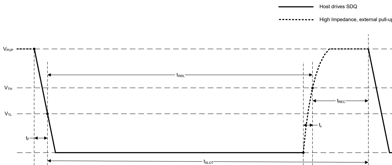
图 6-19. 写入“0”时序图
