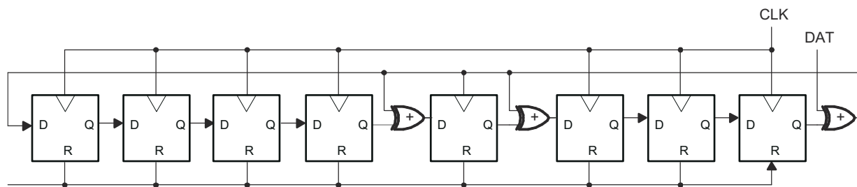
图 6-21. 8 位 CRC 生成器电路 ( X^8 + X^5 + X^4 + 1 )
