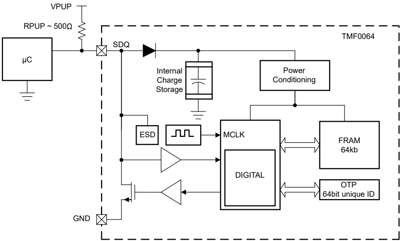
图 6-1. 功能方框图
