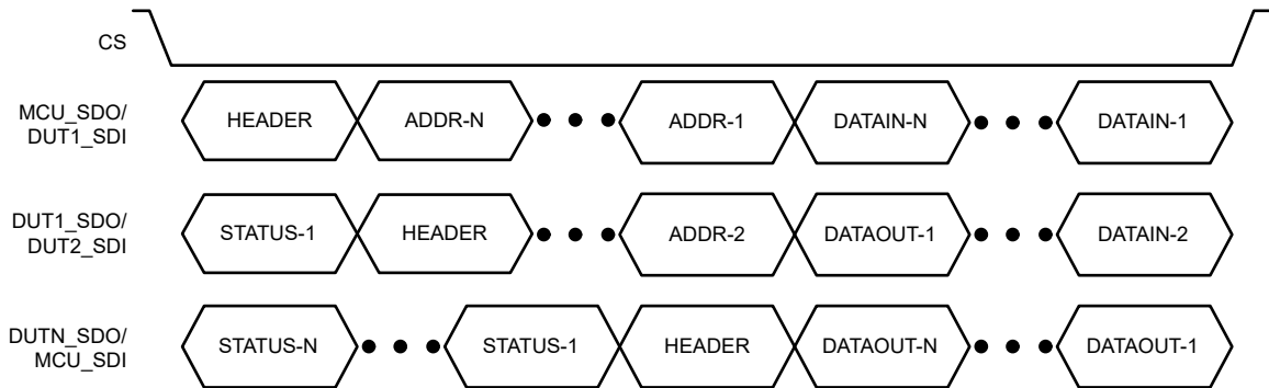
图 7-4. SPI 菊花链数据输出
