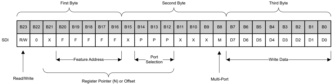
图 7-5. TXE8116 SPI SDI 数据帧格式
