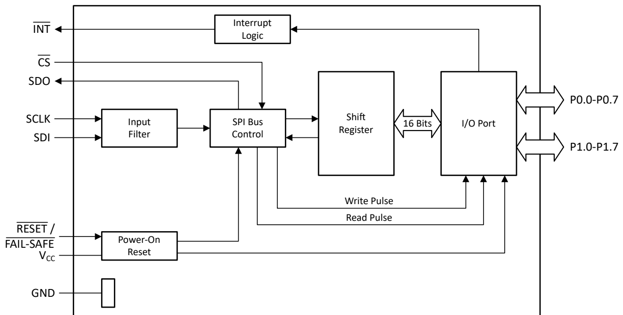
图 7-1. 逻辑图
