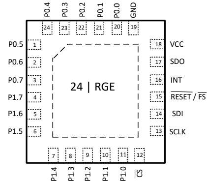
图 4-2. TXE8116 RGE (VQFN) 封装，24 引脚 (顶视图)
