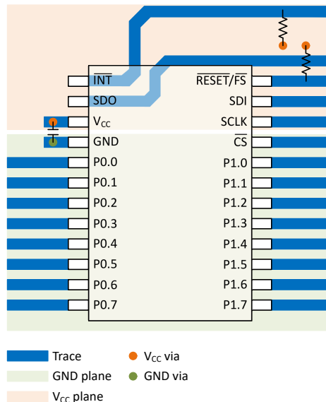
图 8-6. TXE8116 布局
