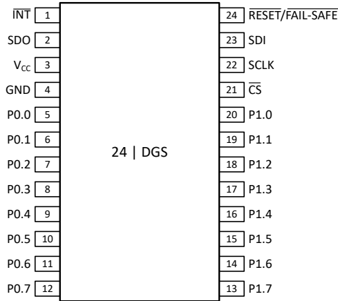
图 4-1. TXE8116 DGS (VSSOP) 封装，24 引脚 (顶视图)
