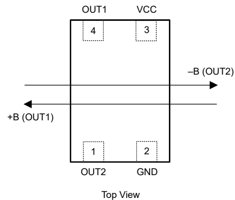
图 7-8. 灵敏度方向
