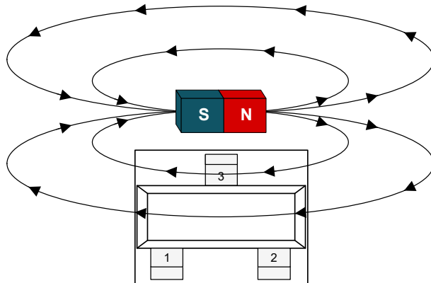
图 7-5. 正磁通密度：磁体偏移
