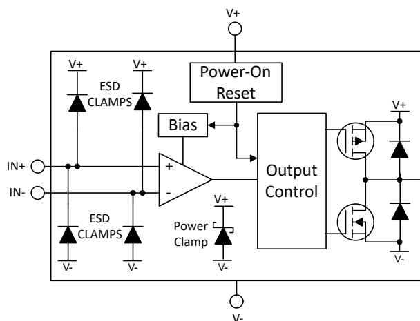
图 6-1. 推挽方框图
