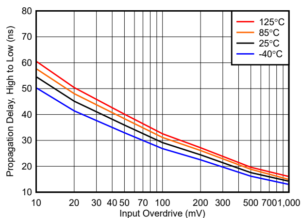
图 5-25. 在 1.8V 时高电平到低电平的传播延迟与过驱间的关系
