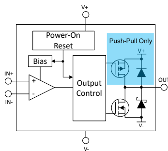
方框图
