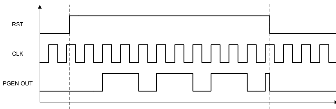
图 8-4. 图形发生器输出计时示意图示例 (SIZE = 3, PATTERN = 011, 低电平 RST)
