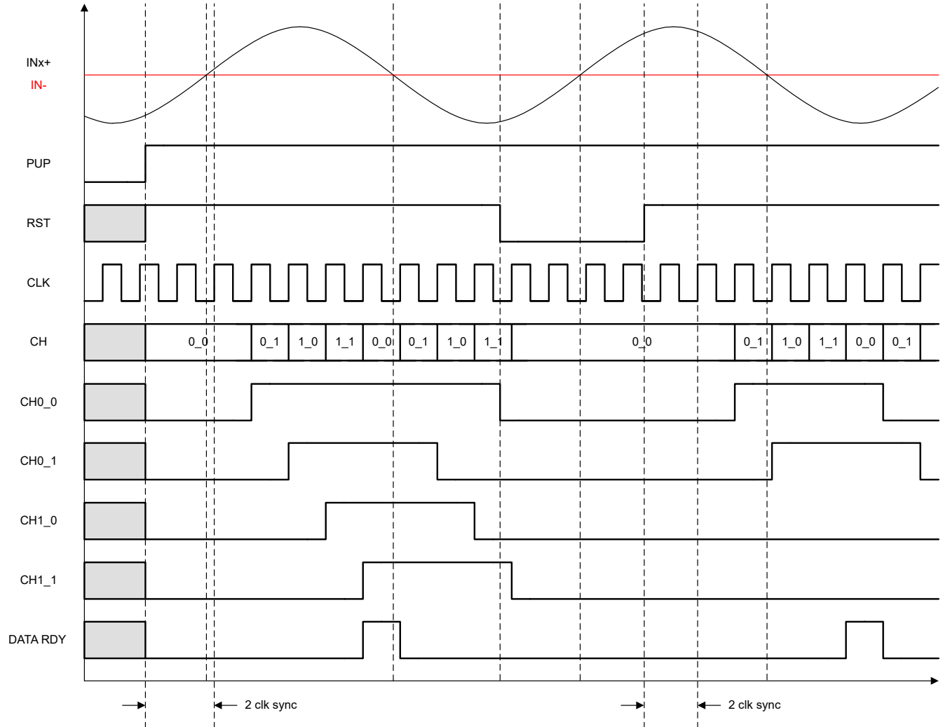
图 8-44. 多通道采样比较器时序示例
