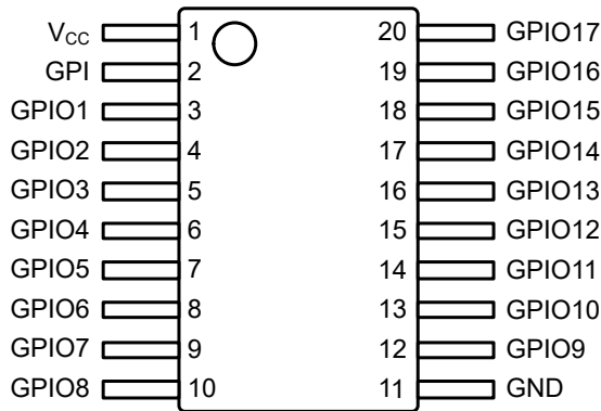
图 4-1. DGS 封装， 20 引脚 VSSOP (俯视图)
