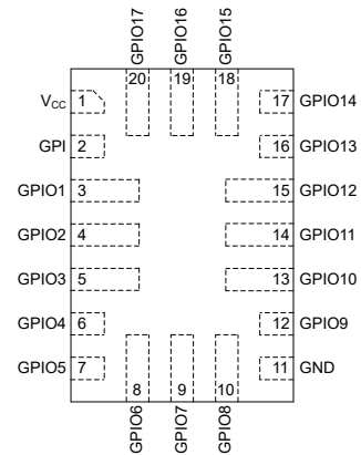
图 4-2. RJY 封装， 20 引脚 UQFN (俯视图)
