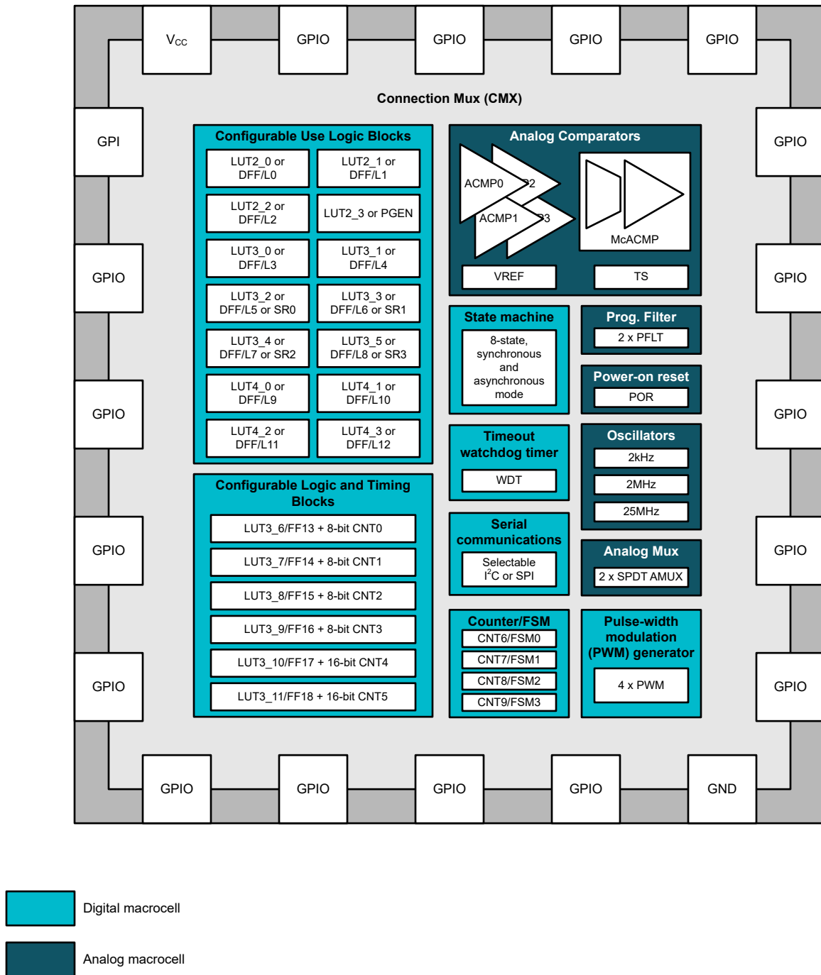
图 8-1. TPLD2001 功能方框图
