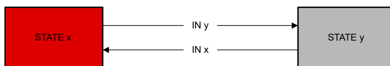
图 8-33. 闭环状态转换
