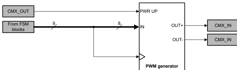
图 8-38. PWM 发生器模块结构图
