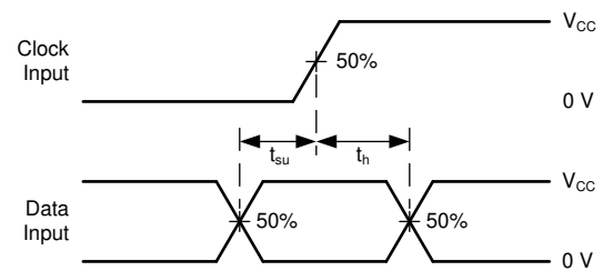
图 7-5. 电压波形，设置和保持时间
