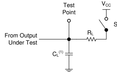
图 7-2. 开漏输出的负载电路
