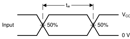
图 7-4. 电压波形，脉冲持续时间
