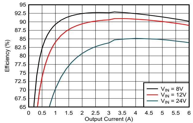
图 8-5. 效率 - FPWM 模式
