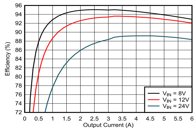
图 8-7. 效率 - FPWM 模式
