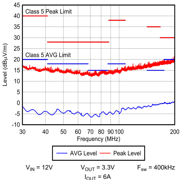
图 8-39. 辐射 EMI (双锥垂直) 与 CISPR 25 限值对比
