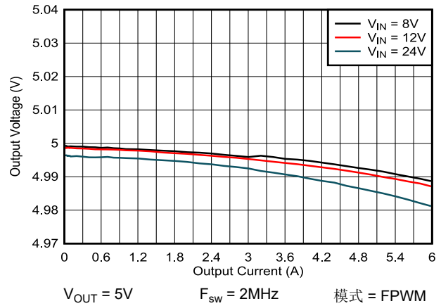
图 8-17. 负载和线路调节 - FPWM 模式
