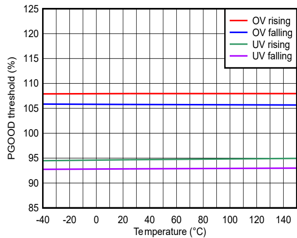
图 6-10. PGOOD 阈值
