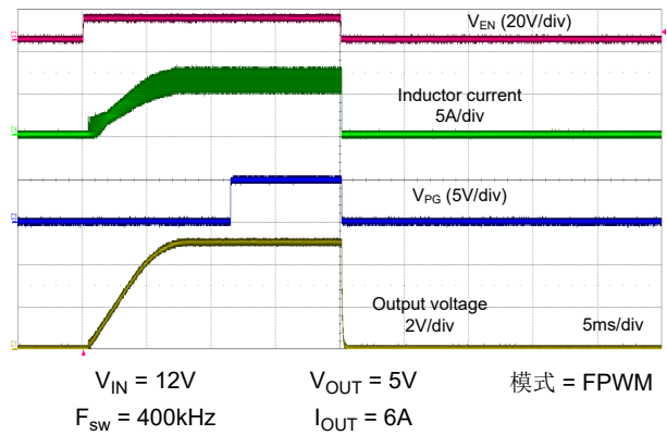
图 8-31. 在 6A 负载条件下实现启动和关断控制
