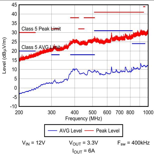
图 8-41. 辐射 EMI (对数周期垂直) 与 CISPR 25 限值对比
