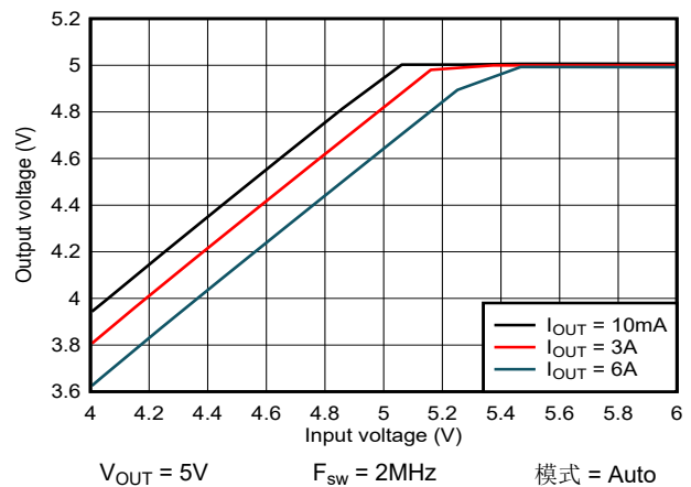
图 8-21. 压降曲线
