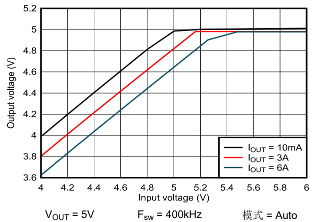
图 8-19. 压降曲线
