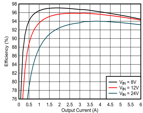
图 8-5. 效率 - FPWM 模式
