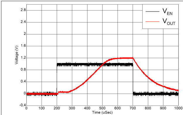
图 7-2. 启动
