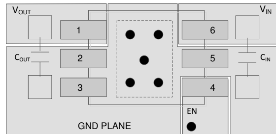
图 7-4. DBV 封装 (SOT-23) 典型布局
