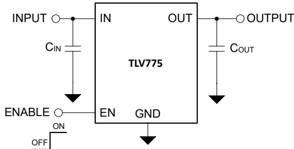
图 7-1. TLV775 典型应用
