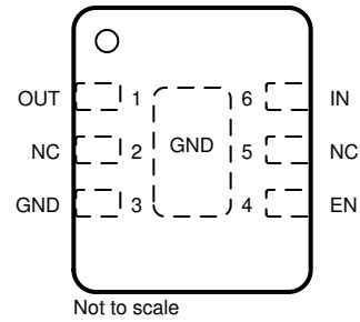
图 4-2. DRV 封装，6 引脚 WSON (俯视图)
