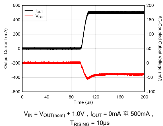
图 5-12. 负载瞬态
