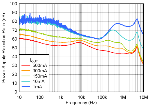
图 7-3. PSRR
