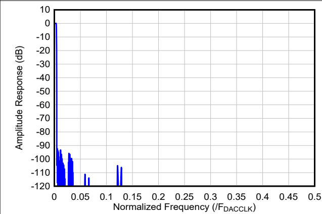
图 7-31. 128 倍内插滤波器响应
