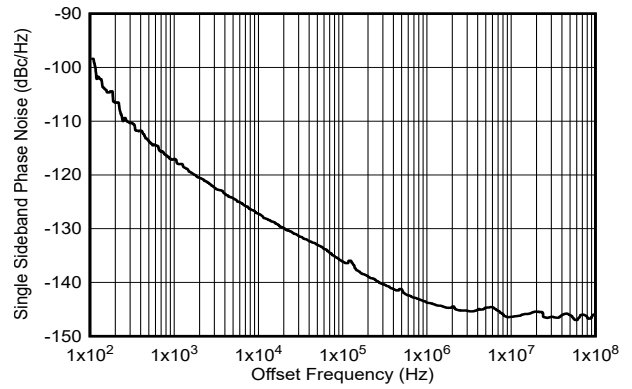
图 9-8. 16.2GHz 频率下的 DAC 附加相位噪声
