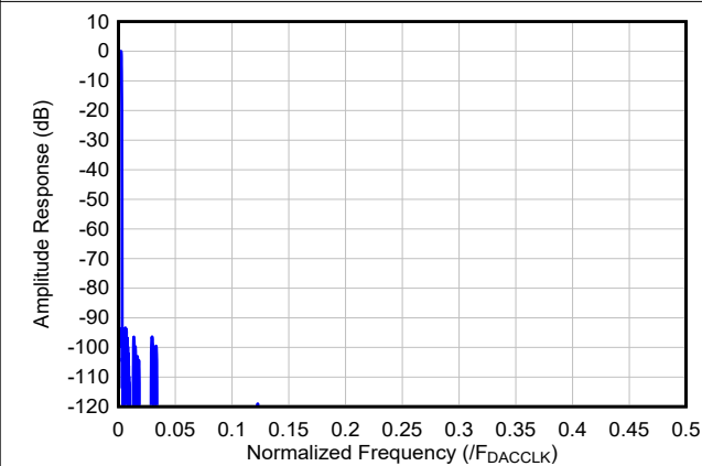
图 7-33. 192 倍内插滤波器响应
