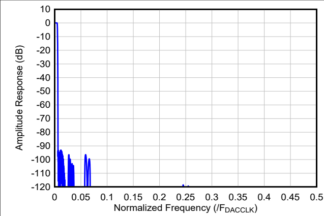
图 7-29. 96 倍内插滤波器响应
