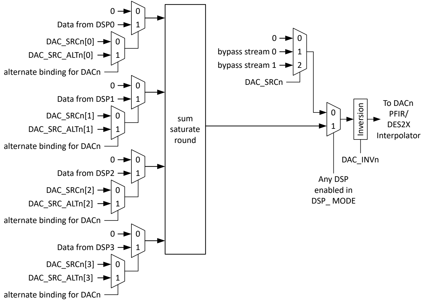
图 7-45. DAC 通道 n 的通道接合器方框图
