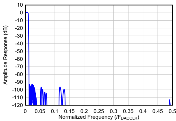
图 7-25. 48 倍内插滤波器响应
