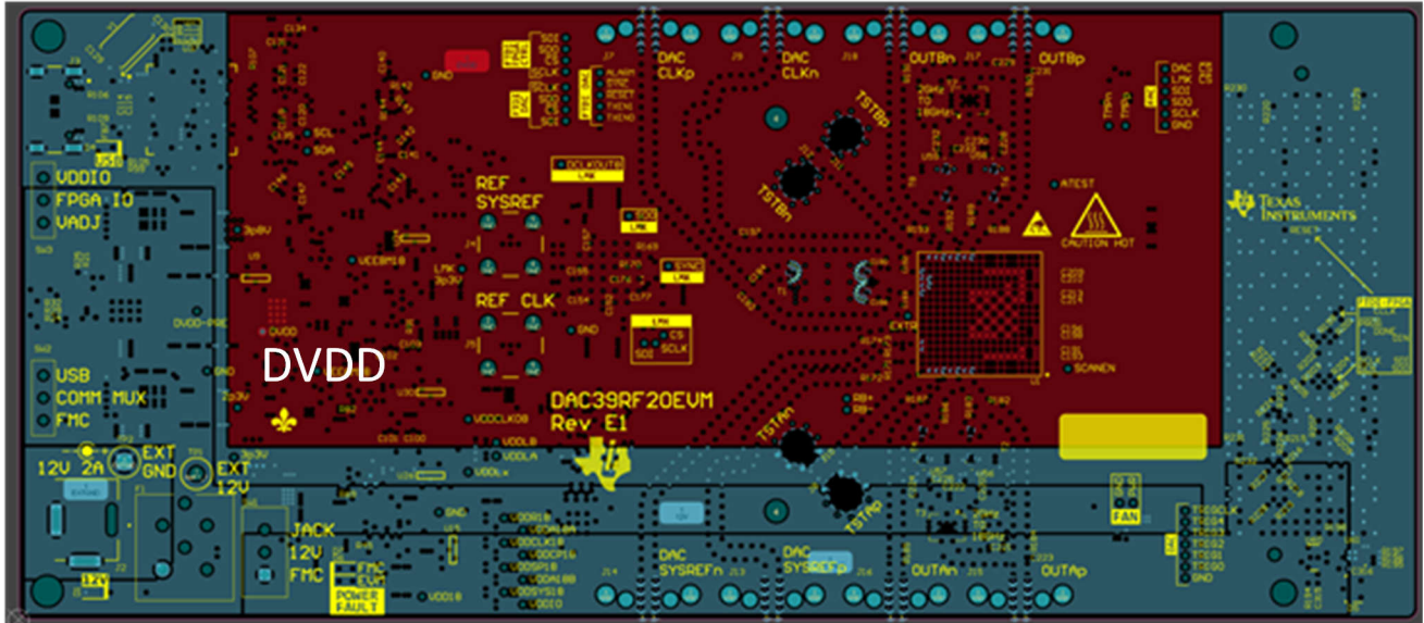
图 9-15. 第 3 层的电源平面布局
