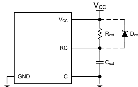
图 8-2. 外部保护二极管连接
