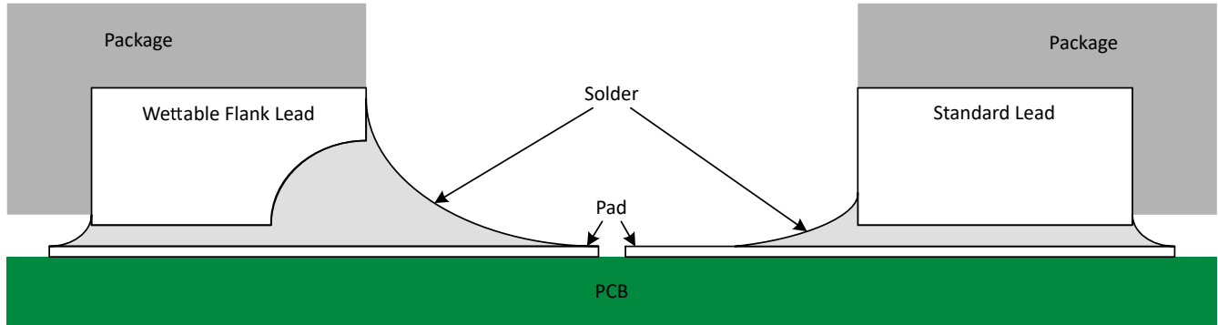
图 7-5. 焊接后具有可润湿侧翼的 QFN 封装和标准 QFN 封装的简化剖面图
