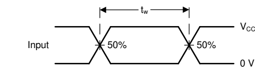
图 6-2. 电压波形，脉冲持续时间
