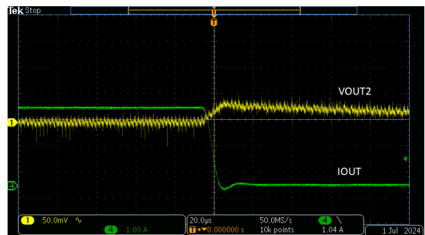
图 9-6. V_{OUT2} 满负载阶跃下降
