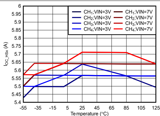
图 6-70. 高侧开关过流阈值与温度间的关系
