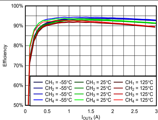
图 6-37. VIN = 7V, VOUTx = 3.3V, fSW = 500kHz 时, 效率与负载间的关系
