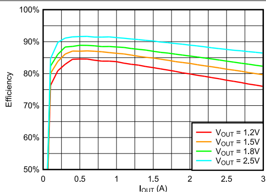
图 6-43. 在 V_{IN} = 3.3V , f_{sw} = 1MHz , 温度 = 25^{\circ}C 条件下, 通道 1 在不同 V_{OUT} 下的效率与负载间的关系
