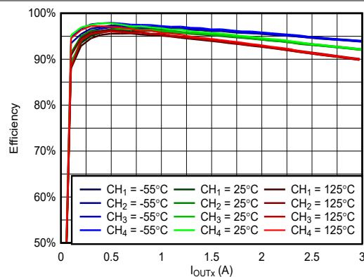
图 6-12. VIN = 5V, VOUTx = 3.3V, fSW = 100kHz 时, 效率与负载间的关系
