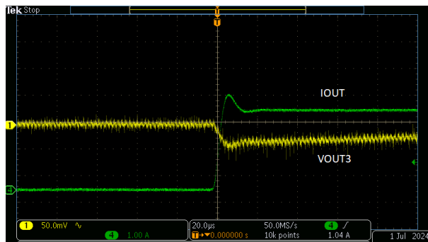
图 9-7. V_{OUT3} 满负载阶跃上升
