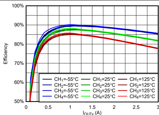
图 6-2. VIN = 3.3V, VOUTX = 1.2V, fSW = 100kHz 时, 效率与负载间的关系
