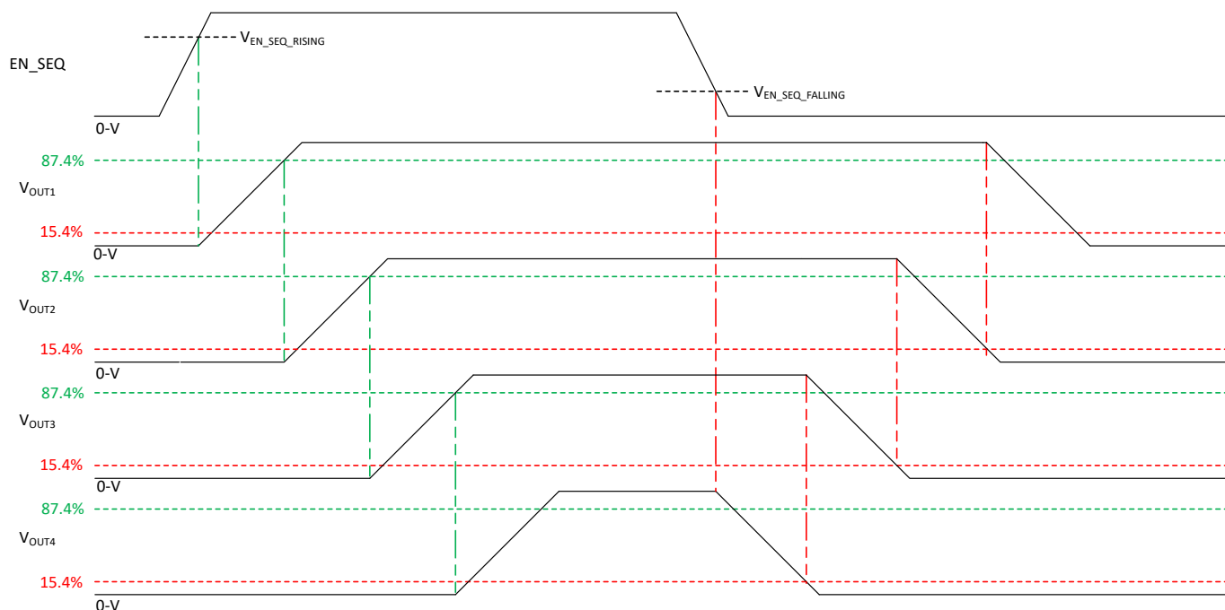
图 8-3. 序列上升/下降
