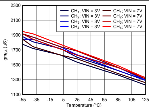
图 6-68. 误差放大器跨导与温度间的关系
