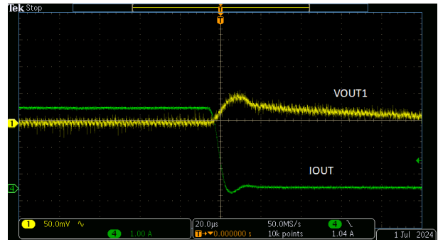
图 9-4. V_{OUT1} 满负载阶跃下降
