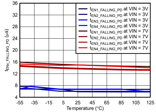
图 6-62. EN 下降电压传播延迟与温度之间的关系
