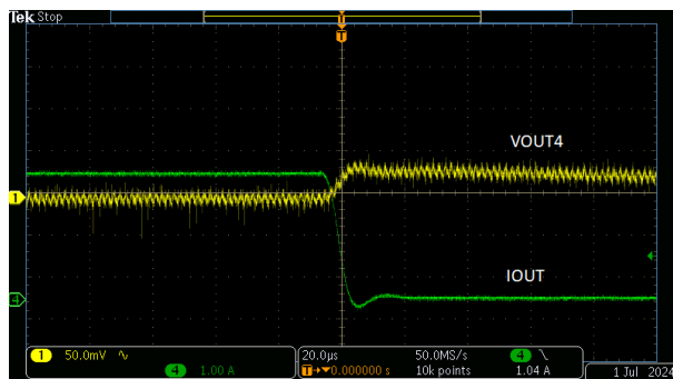
图 9-10. V_{OUT4} 满负载阶跃下降
