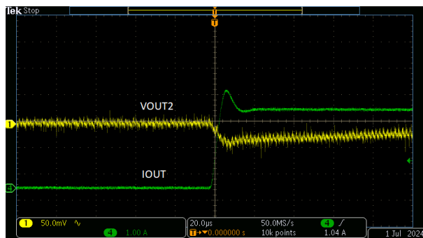
图 9-5. V_{OUT2} 满负载阶跃上升
