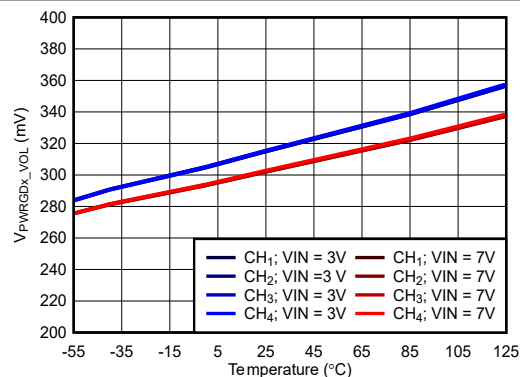
图 6-82. 电源正常输出低电压与温度间的关系
