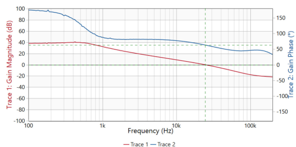
图 9-12. V_{OUT2} 完整环路波德图
