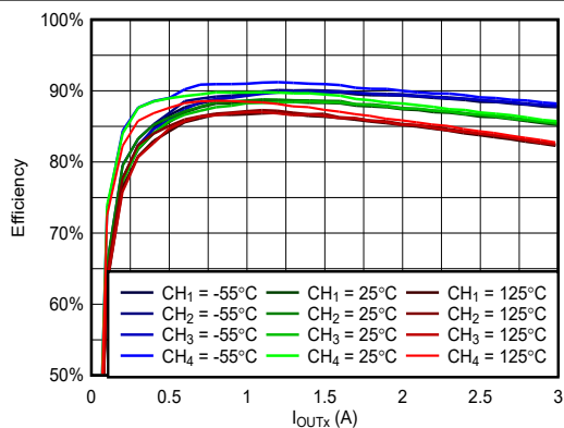
图 6-35. VIN = 7V, VOUTx = 1.8V, fSW = 500kHz 时, 效率与负载间的关系
