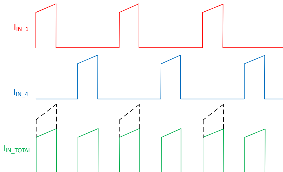
图 9-19. SW1 及 SW4 并联的输入电流波形
