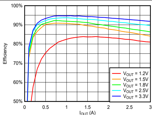
图 6-19. 在 V_{IN} = 7V , f_{SW} = 100kHz , 温度 = 25^{\circ}C 条件下, 通道 1 在不同 V_{OUT} 下的效率与负载间的关系
