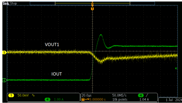
图 9-3. V_{OUT1} 满负载阶跃上升
