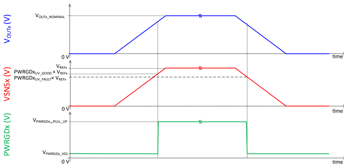
图 8-5. PWRGDx 欠压 (UV) 阈值
