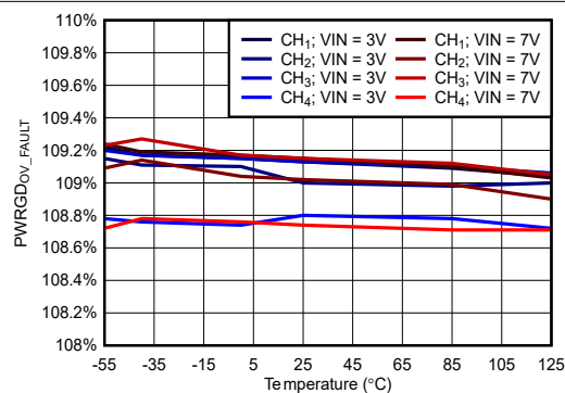
图 6-80. PWRGD 故障状态下 VSNSx 上升阈值与温度间的关系
