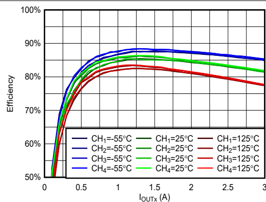
图 6-8. VIN = 5V, VOUTx = 1.2V, fSW = 100kHz 时, 效率与负载间的关系
