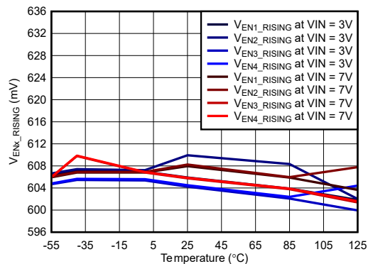
图 6-58. EN 上升阈值与温度之间的关系
