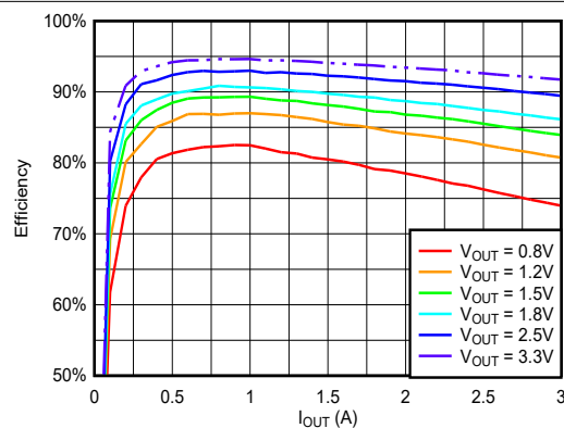
图 6-32. 在 VIN = 5V, fSW = 500kHz, 温度 = 25°C 条件下, 通道 1 在不同 VOUT 下的效率与负载间的关系
