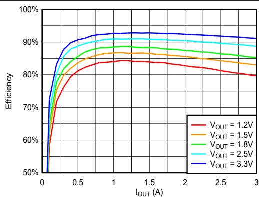
图 6-38. 在 VIN = 7V, fSW = 500kHz, 温度 = 25°C 条件下, 通道 1 在不同 VOUT 下的效率与负载间的关系
