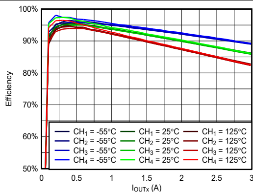
图 6-4. VIN = 3.3V, VOUTX = 1.8V, fSW = 100kHz 时, 效率与负载间的关系
