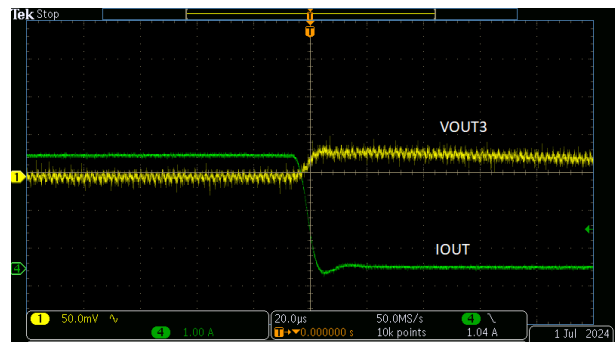
图 9-8. V_{OUT3} 满负载阶跃下降
