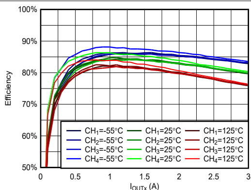
图 6-33. VIN = 7V, VOUTx = 1.2V, fSW = 500kHz 时, 效率与负载间的关系
