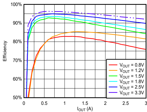
图 6-13. 在 VIN = 5V, f SW = 100kHz, 温度 = 25°C 条件下, 通道 1 在不同 V OUT 下的效率与负载间的关系
