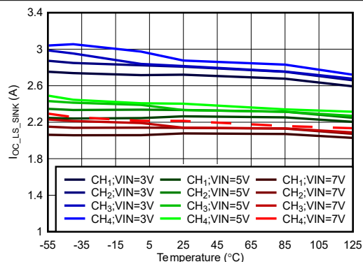
图 6-72. 低侧灌电流开关过流阈值与温度间的关系
