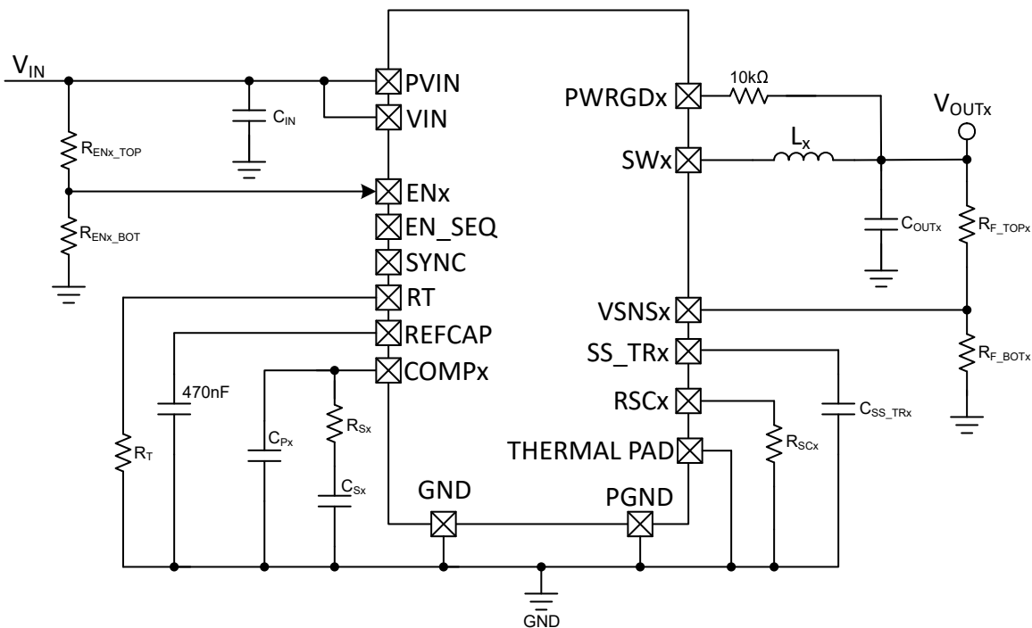
图 9-1. 典型应用原理图
