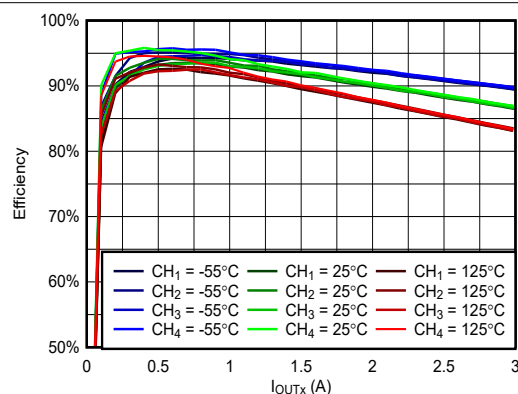
图 6-10. VIN = 5V, VOUTx = 1.8V, fSW = 100kHz 时, 效率与负载间的关系
