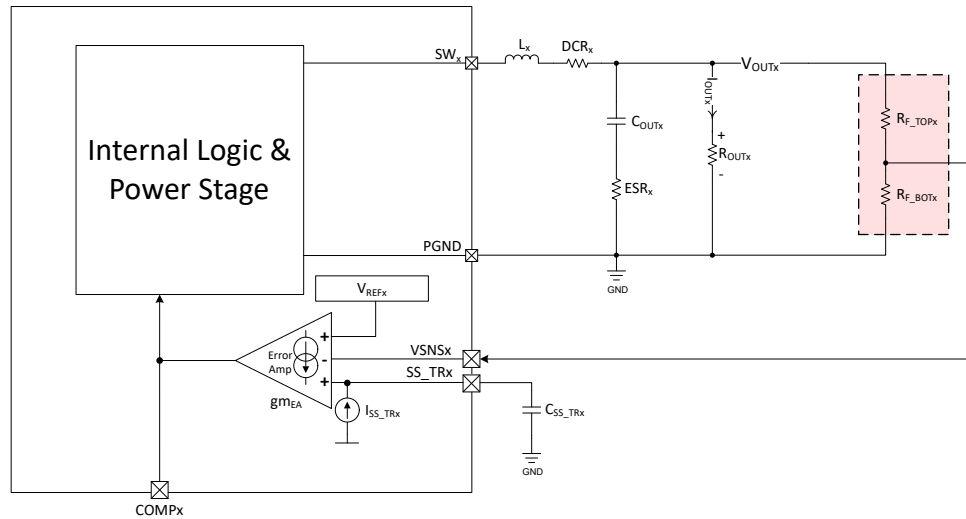
图 8-1. 利用电阻分压器进行 V_{OUTX} 编程
