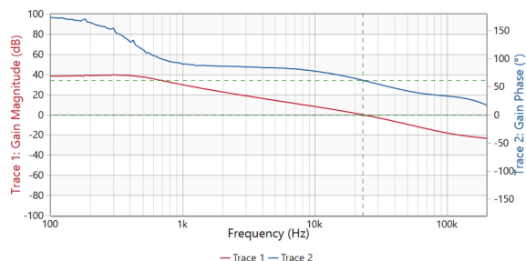
图 9-14. V_{OUT4} 完整环路波德图
