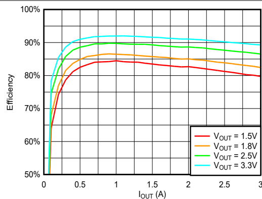
图 6-48. 在 V_{IN} = 5V , f_{sw} = 1MHz , 温度 = 25^{\circ}C 条件下, 通道 1 在不同 V_{OUT} 下的效率与负载间的关系
