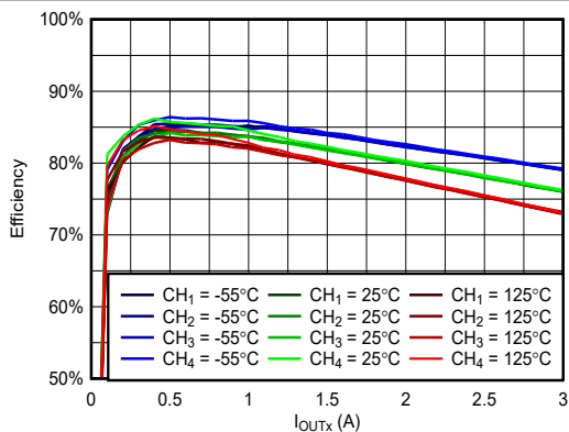
图 6-39. VIN = 3.3V, VOUTx = 1.2V, fSW = 1MHz 时, 效率与负载间的关系
