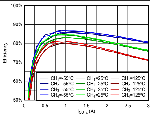
图 6-7. VIN = 5V, VOUTx = 0.8V, fSW = 100kHz 时, 效率与负载间的关系
