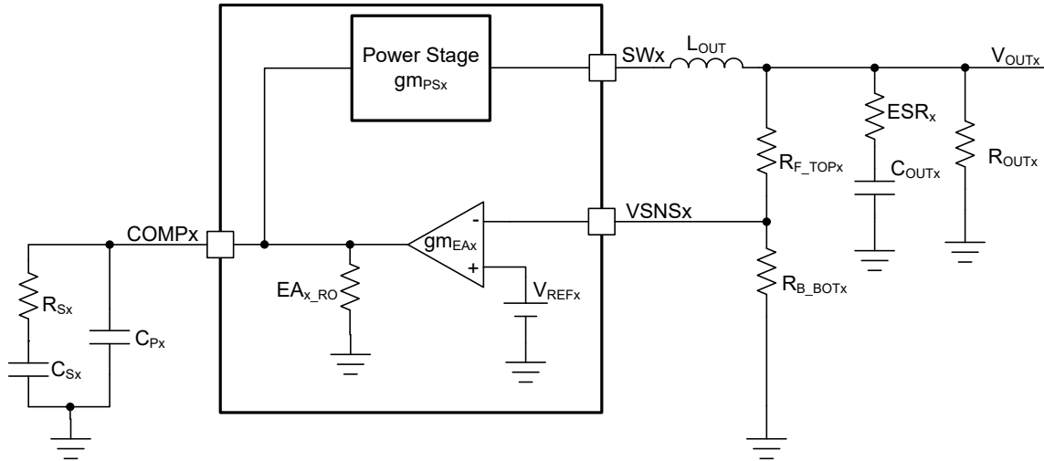
图 8-17. 闭环响应的简化小信号模型
