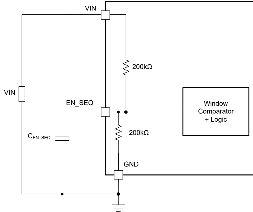
图 8-4. EN_SEQ 上的内部标称阻抗
