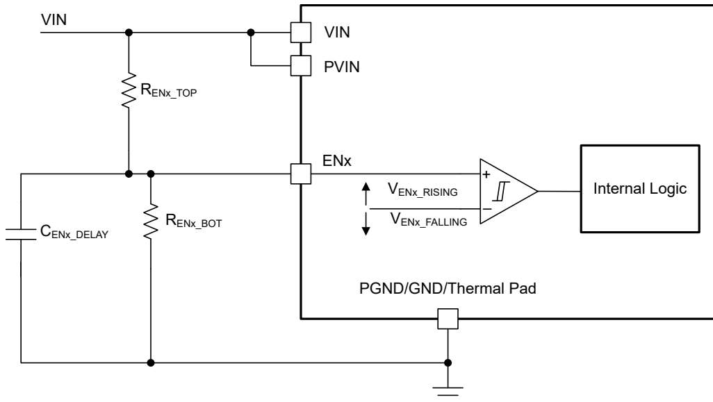
图 8-2. 利用 ENx 与电阻分压器进行外部 UVLO
