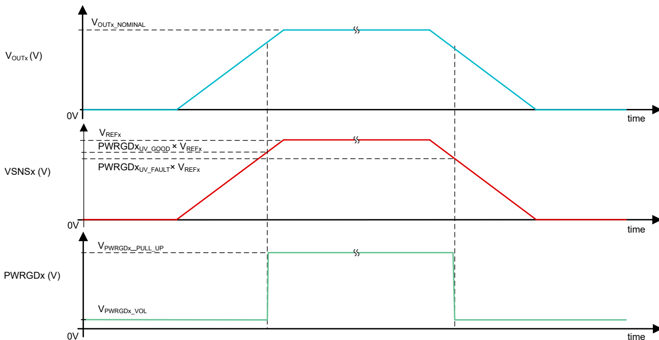
图 8-5. PWRGDx 欠压 (UV) 阈值
