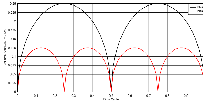
图 9-20. i_{\text{CIN\_RMS\_PARALLEL\_FACTOR}} 与占空比之间的关系
