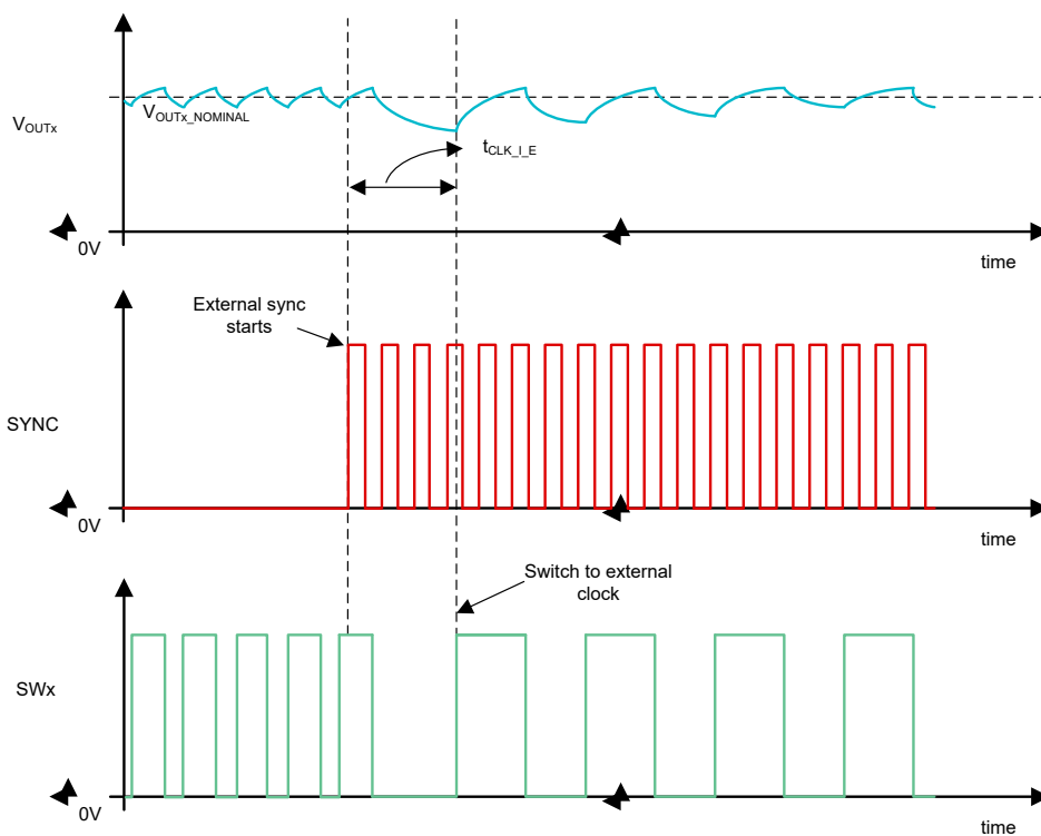
图 8-9. 内部至外部时钟转换
