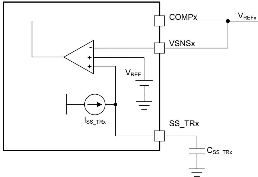
图 7-1. 基准电压测量 ( V_{REFx} )
