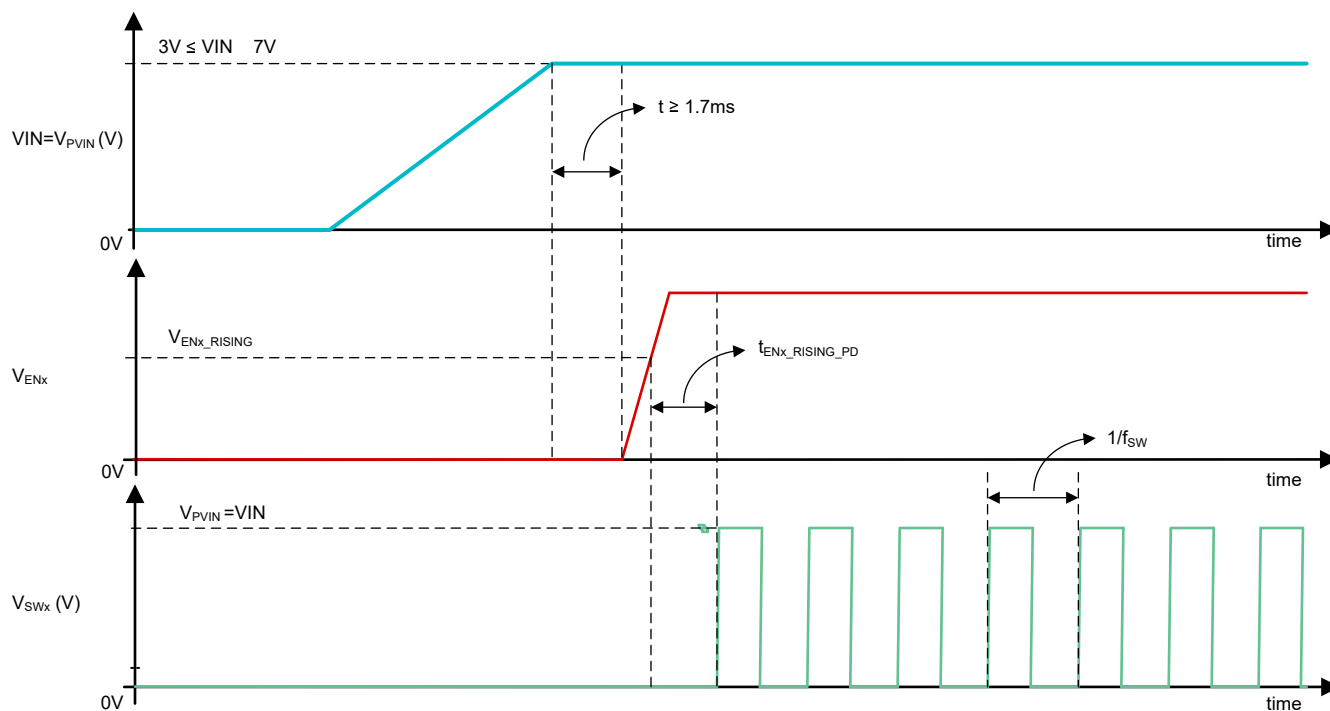
图 7-3. ENx 独立于 PVIN = VIN 驱动时的上升使能传播延迟 ( t_{ENx\_RISING\_PD} )
