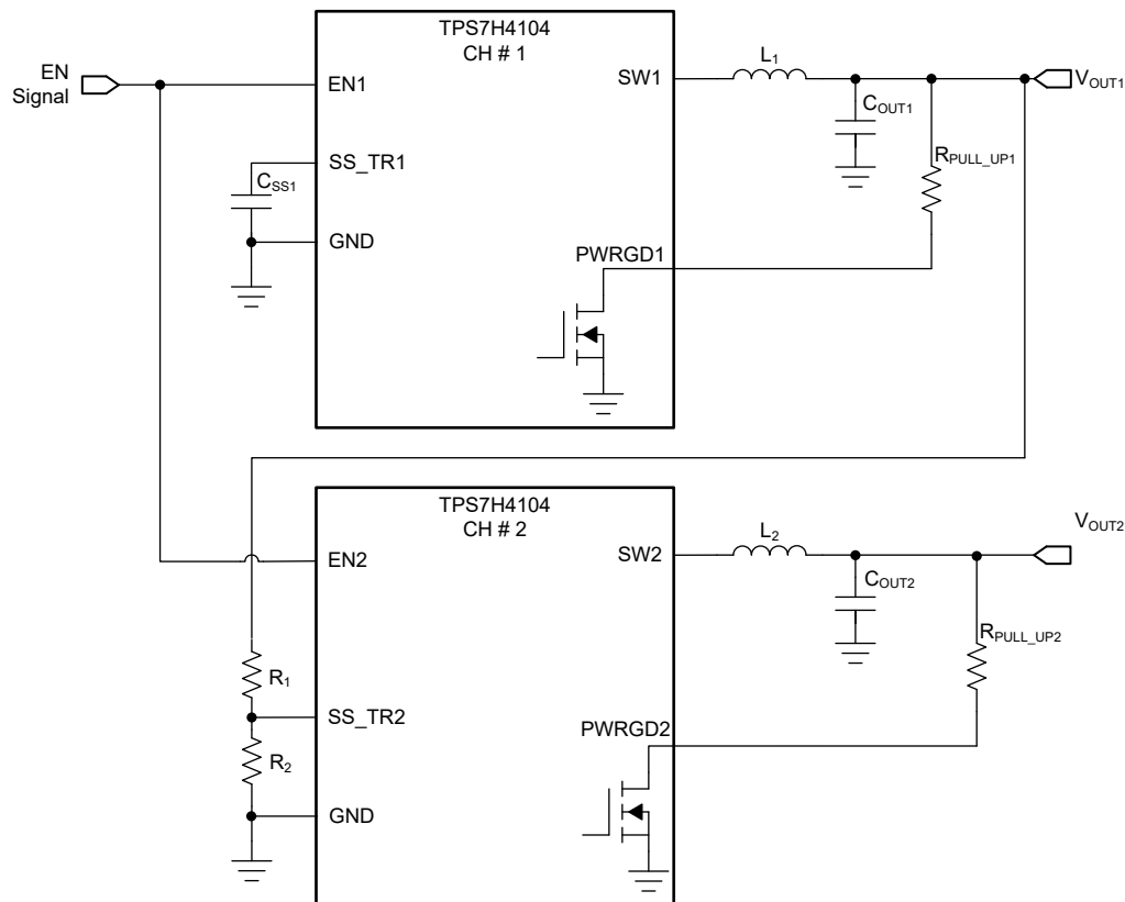
图 8-13. 比例式与同步启动序列
