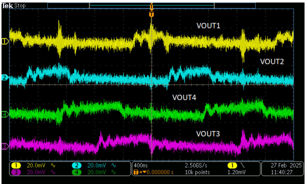
图 9-15. V OUTx 输出电压纹波
