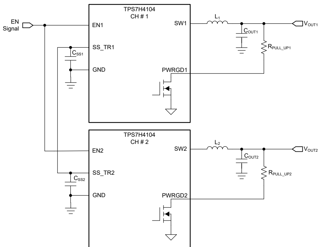
图 8-12. 比例式启动序列
