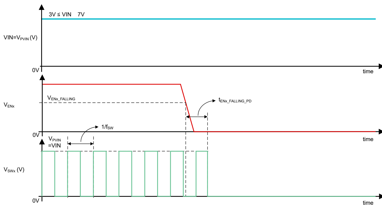
图 7-4. 下降使能传播延迟 ( t_{ENx\_FALLING\_PD} )
