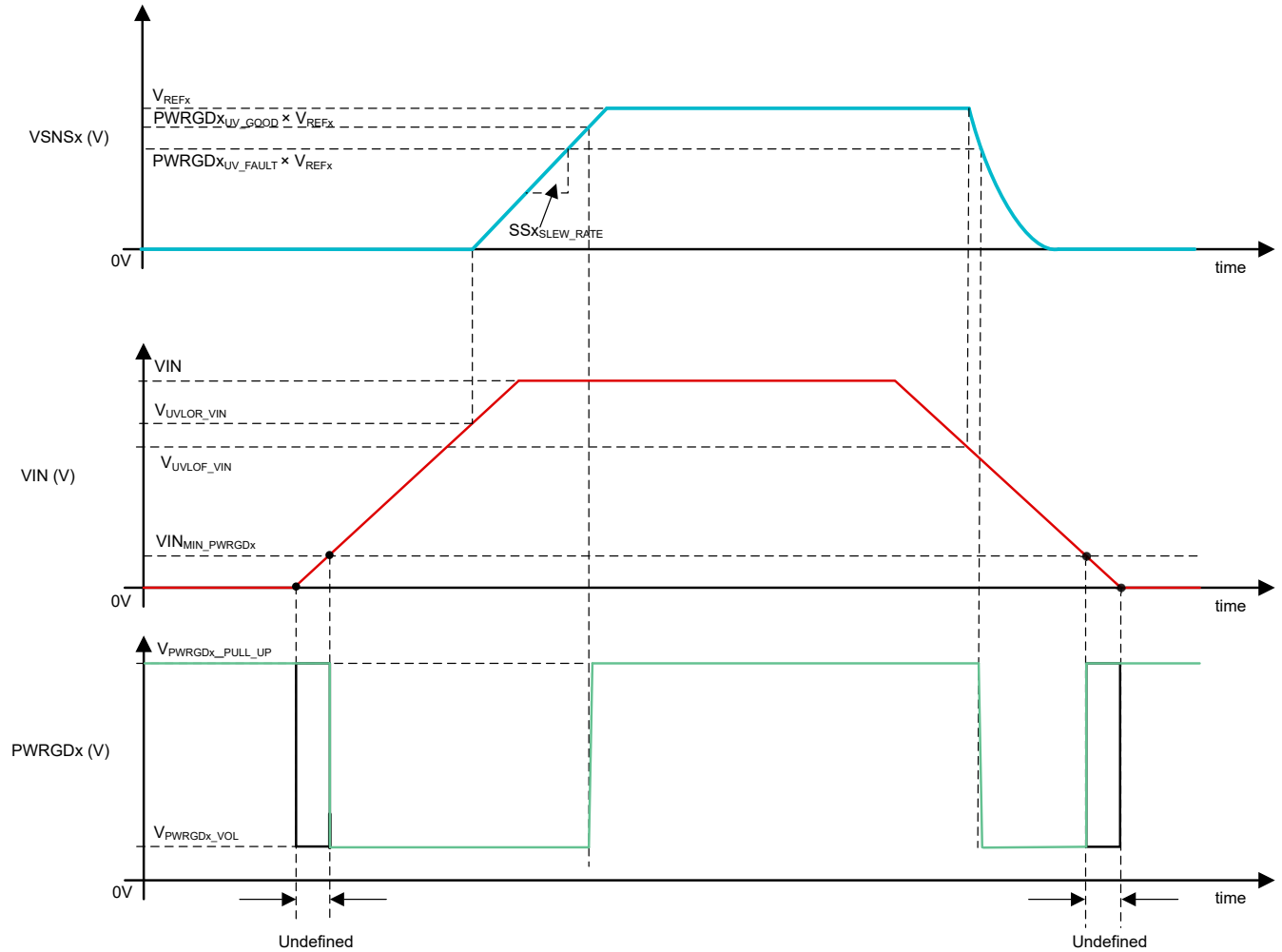
图 8-7. 在 V_{IN} > V_{IN\_MIN\_PWRGDx} 后，处于有效状态的 PWRGDx
