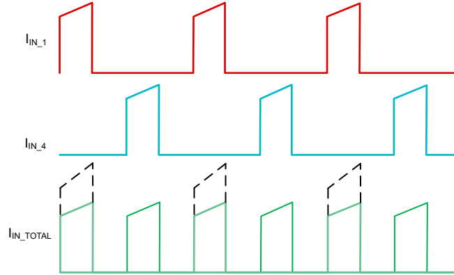
图 9-19. SW1 及 SW4 并联的输入电流波形
