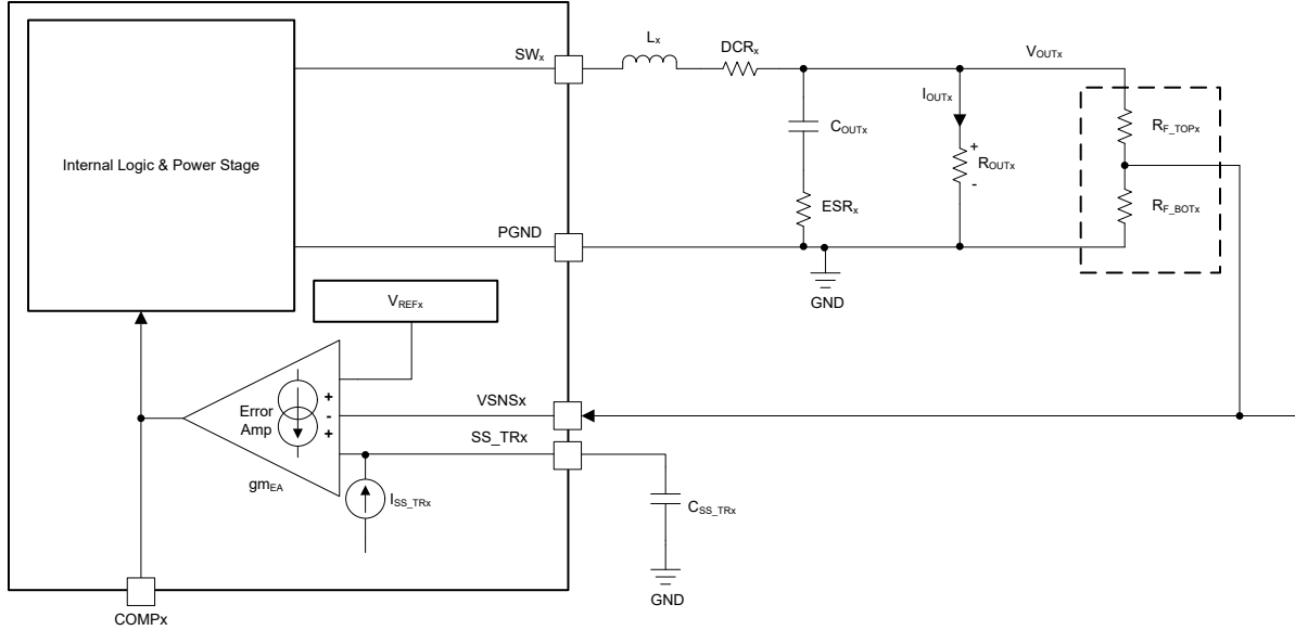
图 8-1. 利用电阻分压器进行 V_{OUTx} 编程
