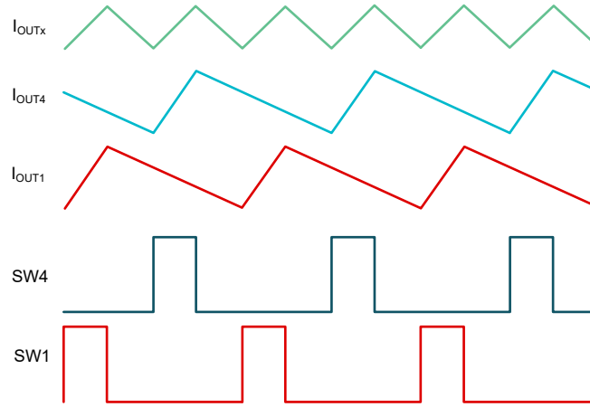
图 9-17. SW1 和 SW4 并联时的电感器纹波电流
