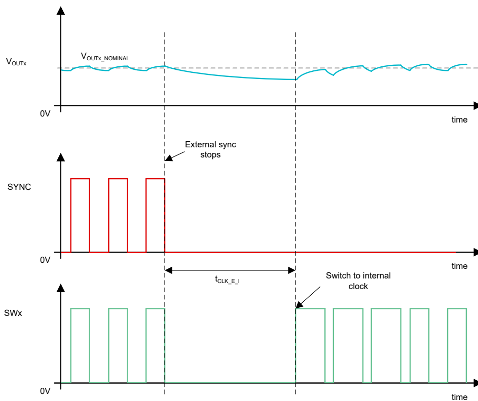
图 8-10. 外部至内部时钟转换
