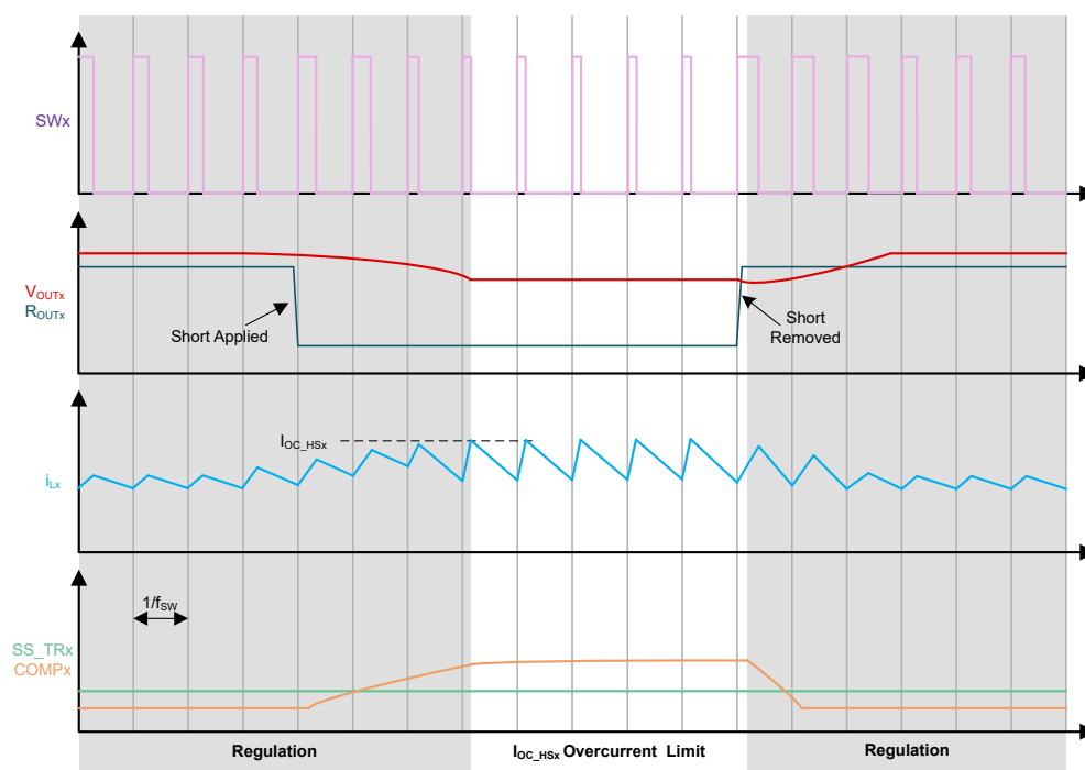
图 8-14. 高侧逐周期过流保护 ( I_{OC\_HSx} )
