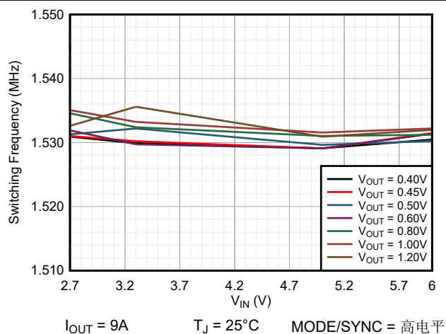
图 6-5. TPSM8287Bxx 开关频率与 V_{IN} 间的关系
