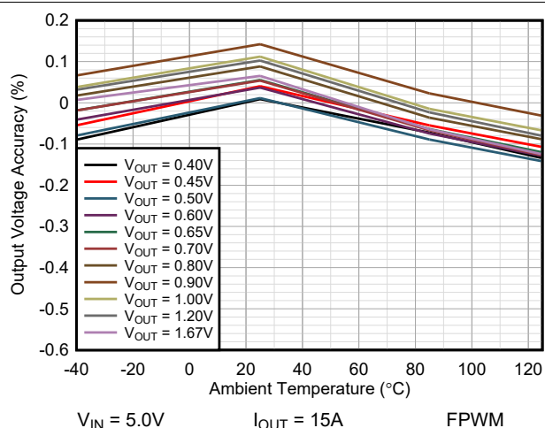
图 9-19. TPSM8287B30xx Vout 精度与温度间的关系
