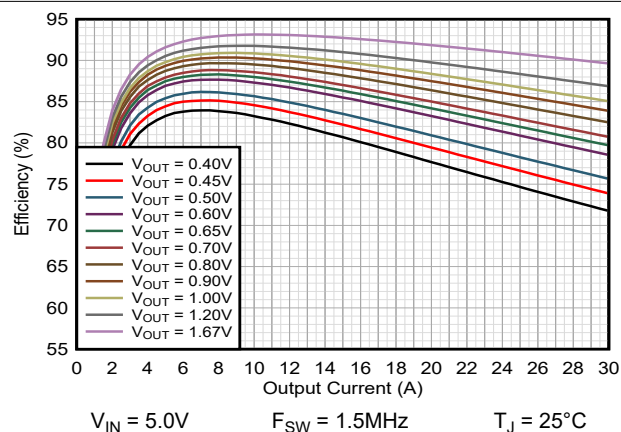
图 9-6. 效率 TPSM8287B30xx FPWM
