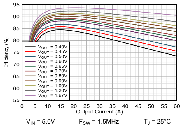
图 9-41. 效率 TPSM8287B30xx FPWM
