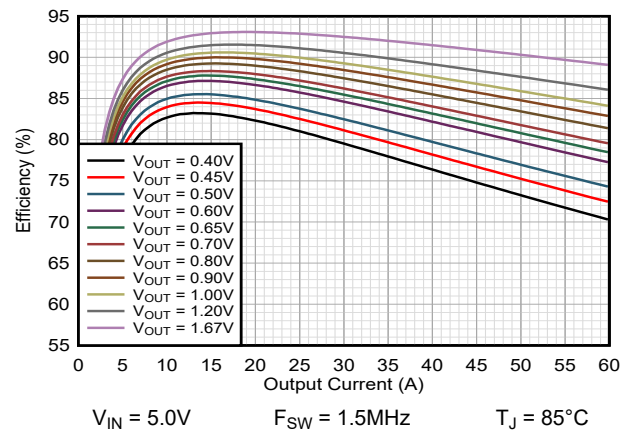
图 9-42. 效率 TPSM8287B30xx FPWM
