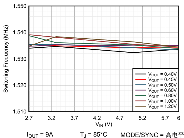
图 6-6. TPSM8287Bxx 开关频率与 V_{IN} 间的关系
