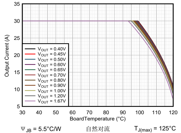
图 9-35. TPSM8287B30xx 安全工作区, V_{IN} = 5.0\text{V}
