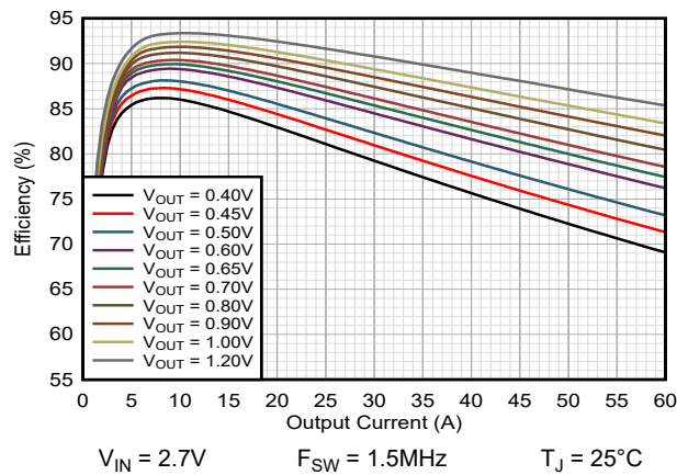
图 9-37. 效率 TPSM8287B30xx FPWM
