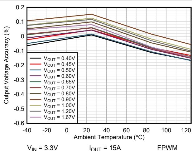
图 9-17. TPSM8287B30xx Vout 精度与温度间的关系
