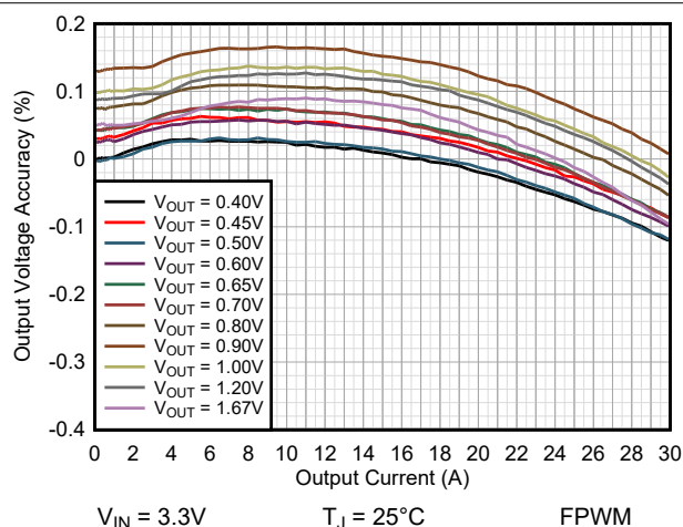
图 9-16. TPSM8287B30xx 负载调整率
