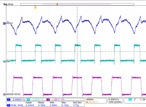
图 9-23. TPSM8287B30HAPx PWM-DCM 运行
