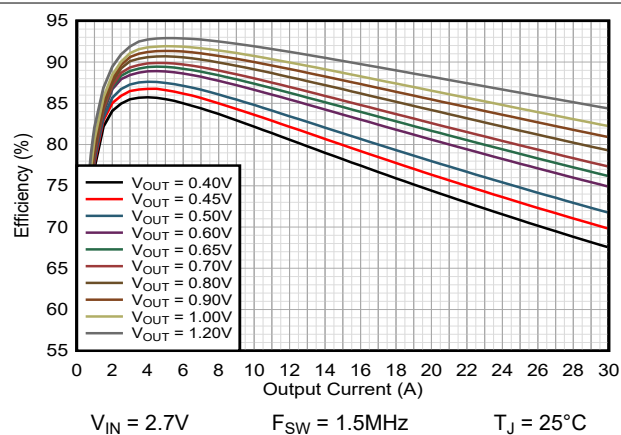
图 9-2. 效率 TPSM8287B30xx FPWM
