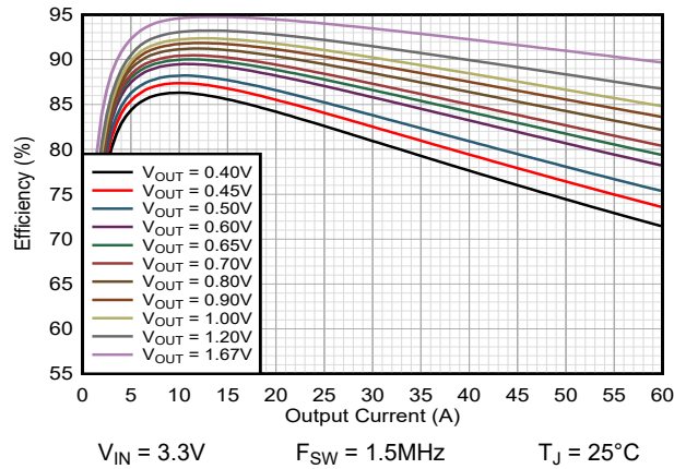
图 9-39. 效率 TPSM8287B30xx FPWM
