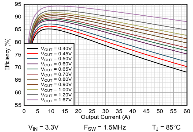
图 9-40. 效率 TPSM8287B30xx FPWM
