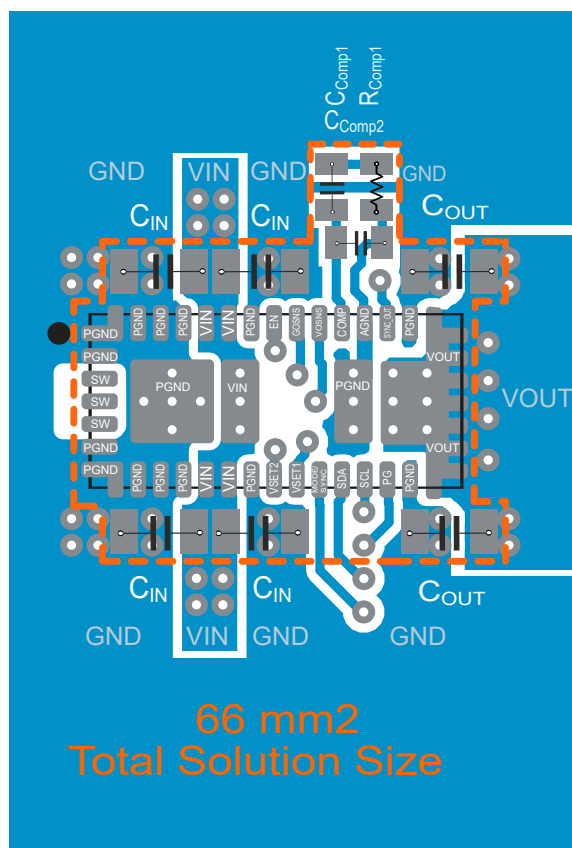
图 9-47. 布局示例
