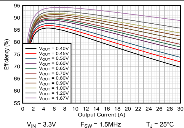
图 9-4. 效率 TPSM8287B30xx FPWM
