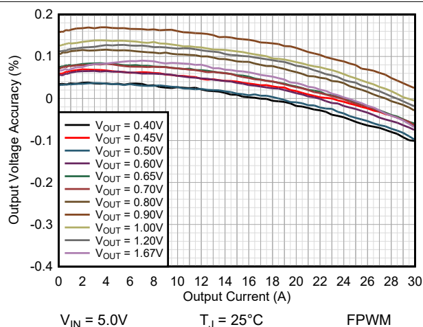
图 9-18. TPSM8287B30xx 负载调整率
