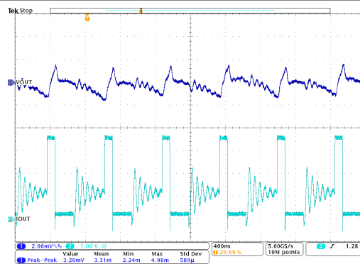
图 9-21. 负载瞬态 TPSM8287B30HAPx
