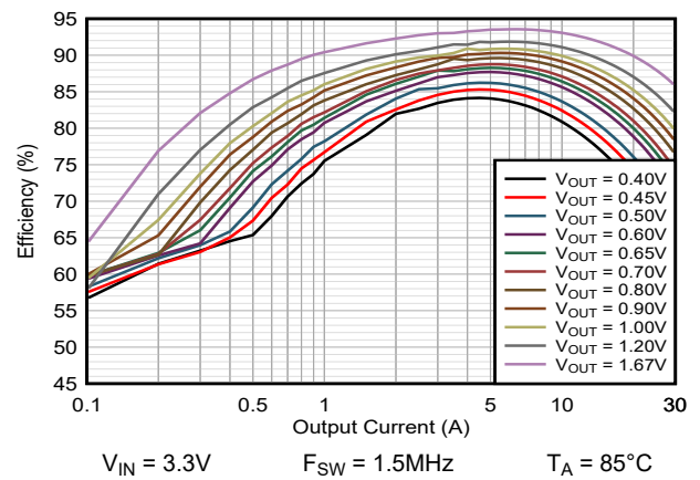
图 9-11. 效率 TPSM8287B30xx PSM
