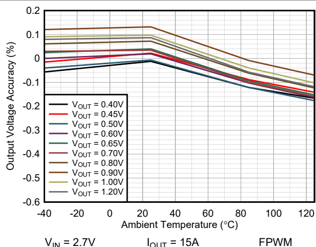
图 9-15. TPSM8287B30xx Vout 精度与温度间的关系
