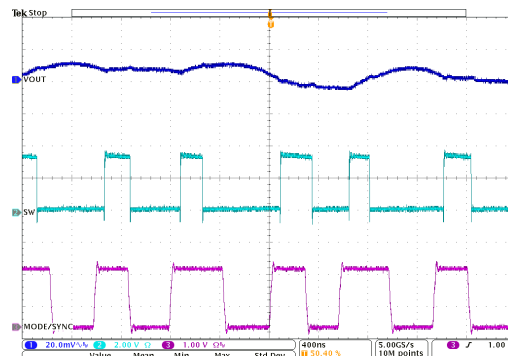
图 9-27. TPSM8287B30HAPx 与随机外部时钟同步
