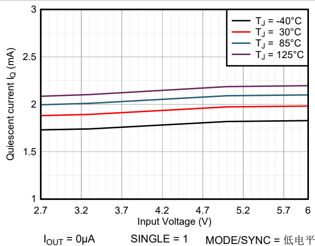
图 6-1. 工作电源电流 (节能模式)
