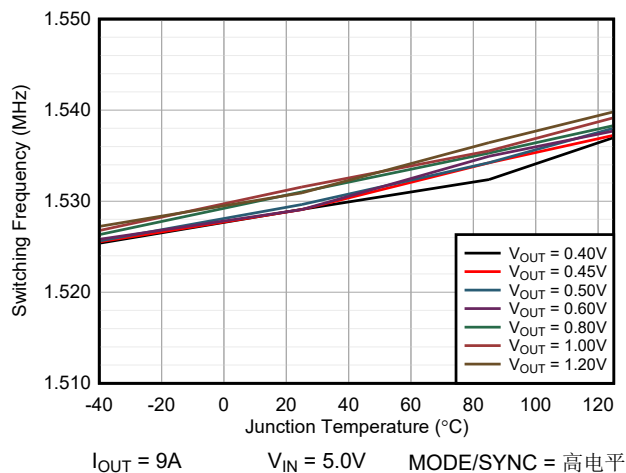
图 6-4. TPSM8287Bxx 开关频率与 T_J 间的关系
