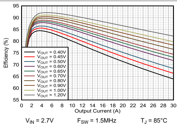
图 9-3. 效率 TPSM8287B30xx FPWM
