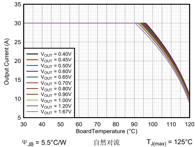
图 9-34. TPSM8287B30xx 安全工作区, V_{IN} = 3.3\text{V}
