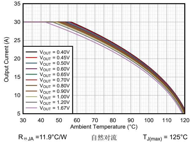
图 9-32. TPSM8287B30xx 安全工作区, V_{IN} = 3.3\text{V}
