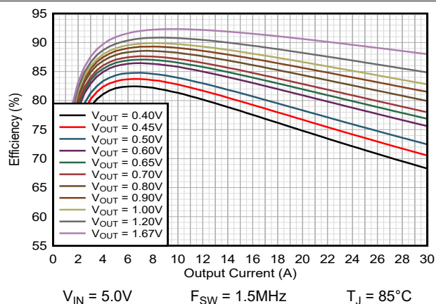
图 9-7. 效率 TPSM8287B30xx FPWM
