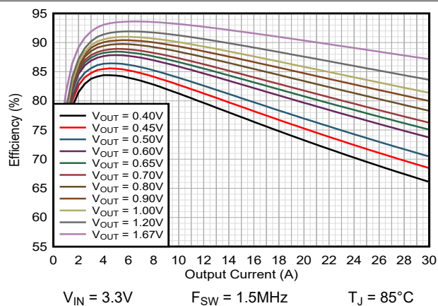
图 9-5. 效率 TPSM8287B30xx FPWM
