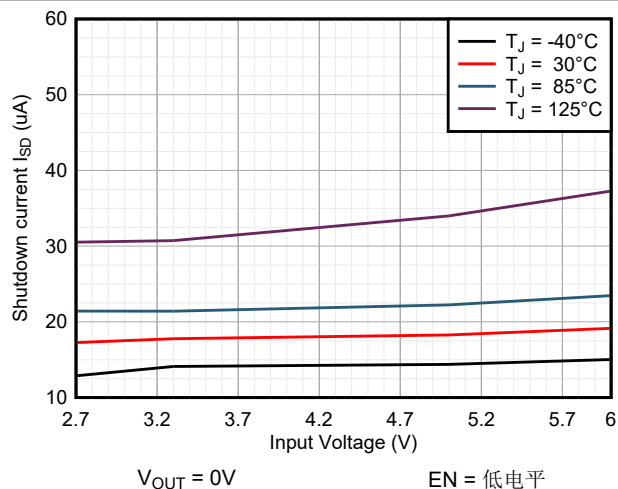
图 6-2. 关断电流
