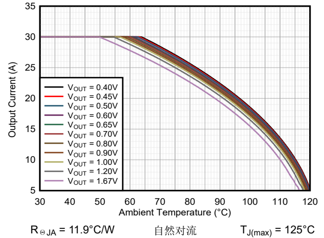
图 9-33. TPSM8287B30xx 安全工作区, V_{IN} = 5.0\text{V}
