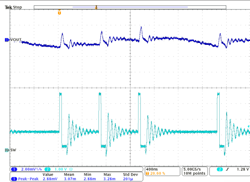
图 9-22. TPSM8287B30HAPx PWM-CCM 运行
