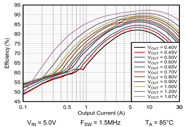
图 9-13. 效率 TPSM8287B30xx PSM
