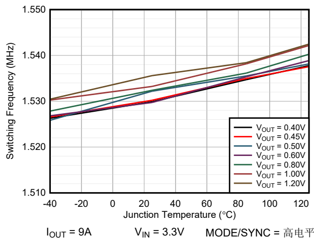
图 6-3. TPSM8287Bxx 开关频率与 T_J 间的关系
