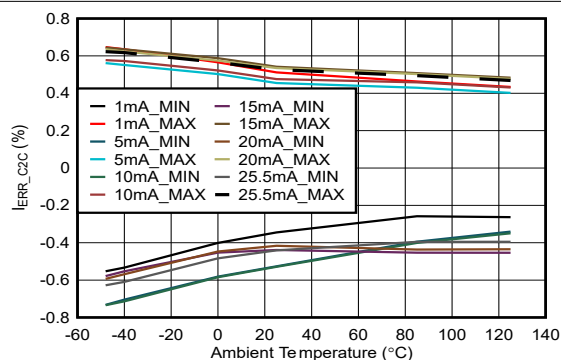
图 6-12. 通道间电流精度与温度间的关系 (MC = 0, VCC = 3.6V)
