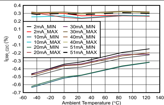
图 6-13. 通道间电流精度与温度间的关系 (MC = 1, VCC = 3.6V)
