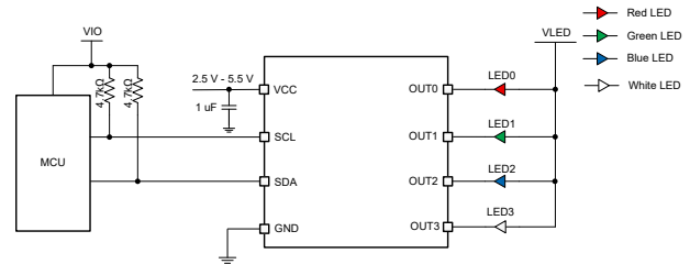
LP5816 简化原理图
