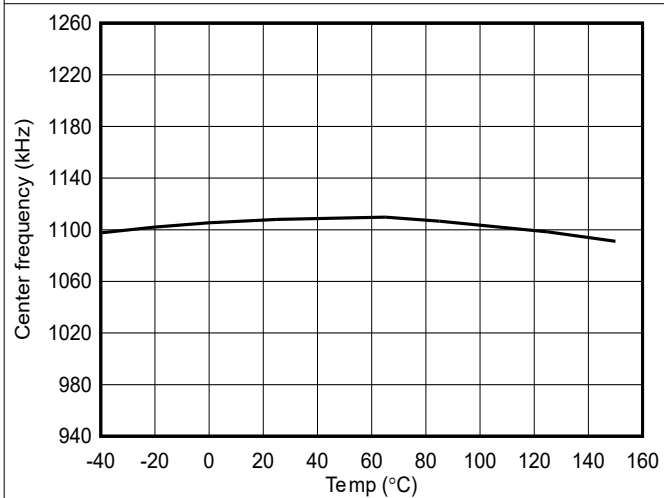
图 5-5. 中心开关频率与结温间的关系
