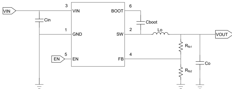
TPS561300 简化原理图
