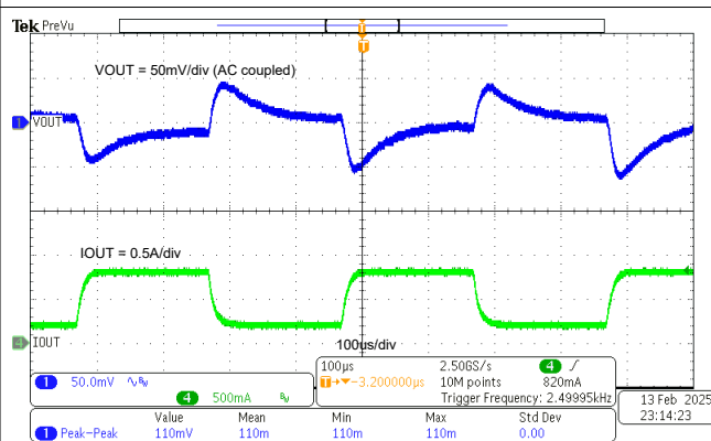
图 7-5. TPS561300EVM 负载瞬态响应, 0.2A 至 0.8A 负载阶跃
