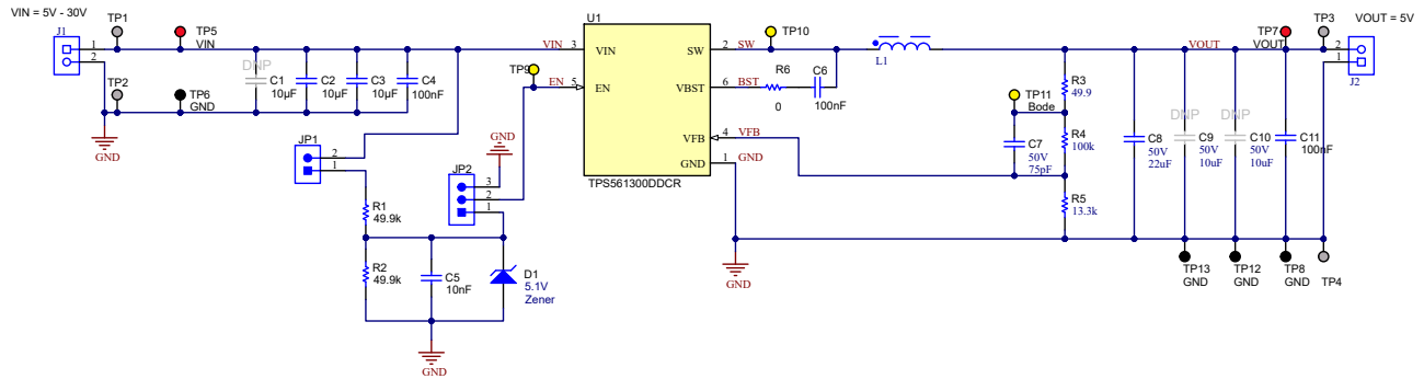
图 7-1. 5V、1A 参考设计
