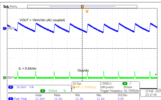
图 7-3. TPS561300EVM 输出电压纹波, I_{OUT} = 0.01A
