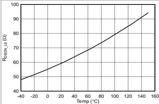
图 5-3. 低侧 FET 导电电阻与结温间的关系
