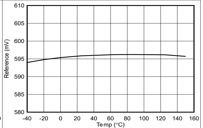
图 5-4. 基准电压与结温间的关系
