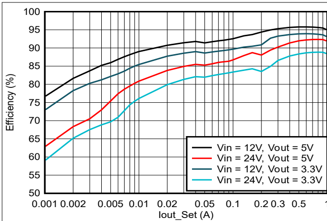
图 7-8. TPS561300EVM 效率与输出电流间的关系
