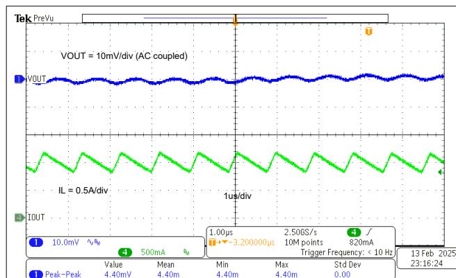
图 7-2. TPS561300EVM 输出电压纹波, I_{OUT} = 1A
