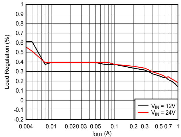
图 7-9. TPS561300EVM 负载调整率
