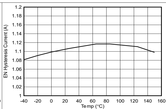
图 5-8. EN 迟滞电流与结温间的关系
