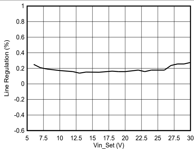
图 7-10. TPS561300EVM 线性调整率, I_{OUT} = 1A
