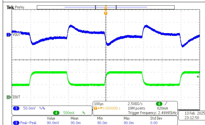
图 7-4. TPS561300EVM 负载瞬态响应, 0.5A 至 1A 负载阶跃
