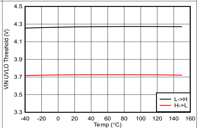
图 5-6. VIN UVLO 阈值与结温间的关系
