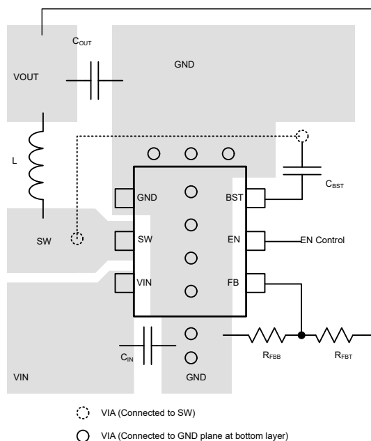
图 7-12. 电路板布局
