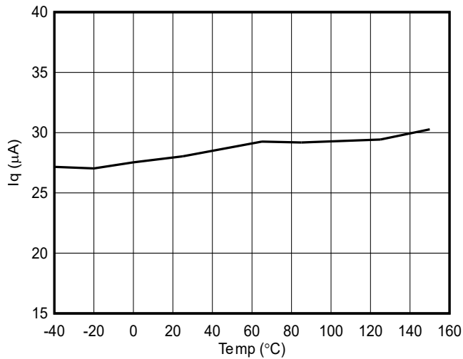
图 5-1. 非开关工作静态电流与结温间的关系
