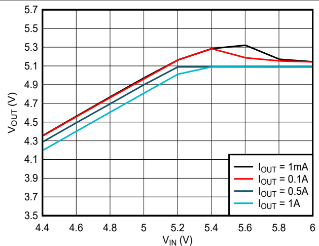
图 7-11. TPS561300EVM 压降
