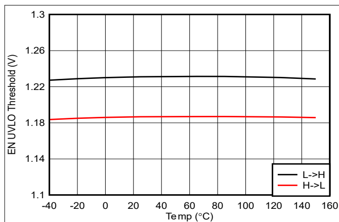
图 5-7. EN 阈值与结温间的关系
