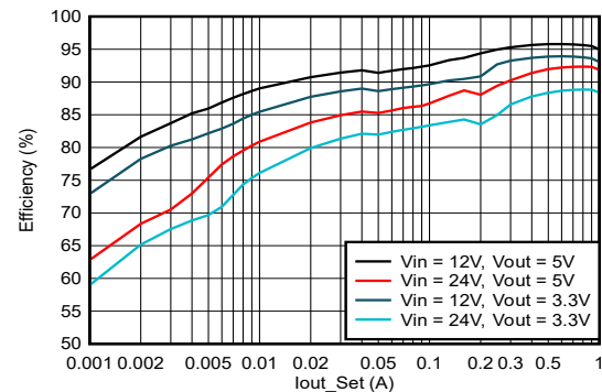
效率与输出电流之间的关系
