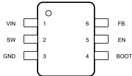
图 4-2. 6 引脚 SOT-563 DRL 封装 (顶视图)
