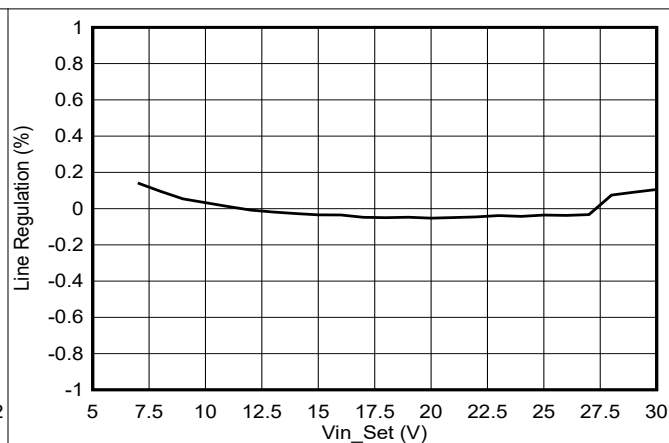
图 7-3. TPS542021EVM 线性调整率, I_{OUT} = 2A
