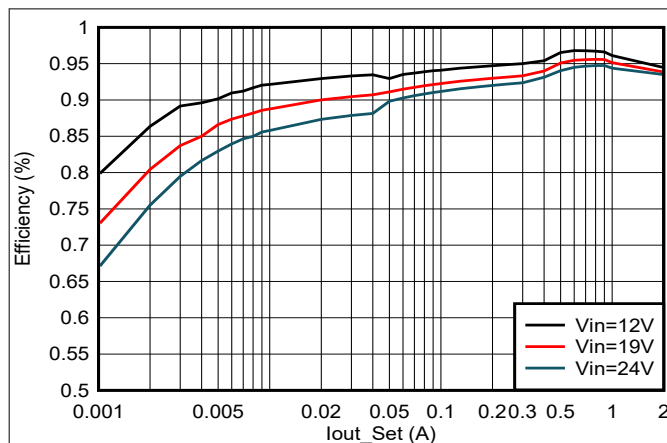
图 7-2. TPS542021EVM 效率
