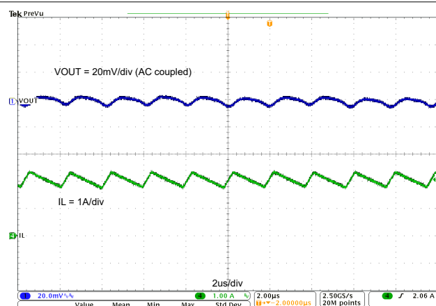
图 7-5. TPS542021EVM 输出电压纹波, I_{OUT} = 2A
