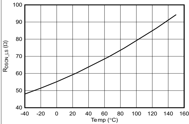
图 5-3. 低侧 FET 导通电阻与结温间的关系
