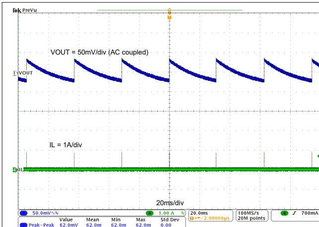
图 7-8. TPS542021EVM 输出电压纹波, I_{OUT} = 0A
