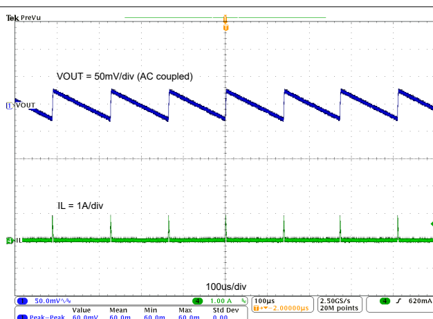
图 7-7. TPS542021EVM 输出电压纹波, I_{OUT} = 0.01A
